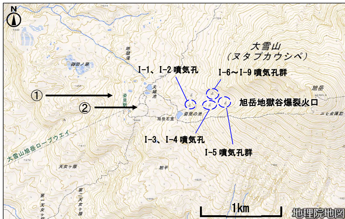
図3 大雪山 旭岳地獄谷爆裂火口内の噴気孔の位置（破線囲み）および写真の撮影方向（矢印）
