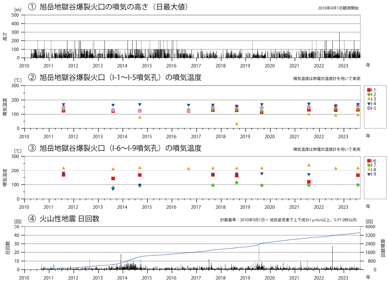
図2 大雪山 火山活動経過図（2010年4月～2023年8月）
