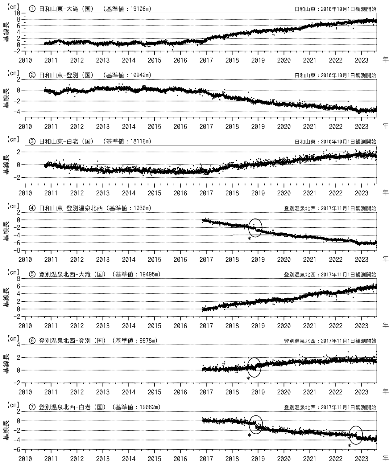
図3 倶多楽 GNSS連続観測による基線長変化 (2010年10月～2023年7月)
