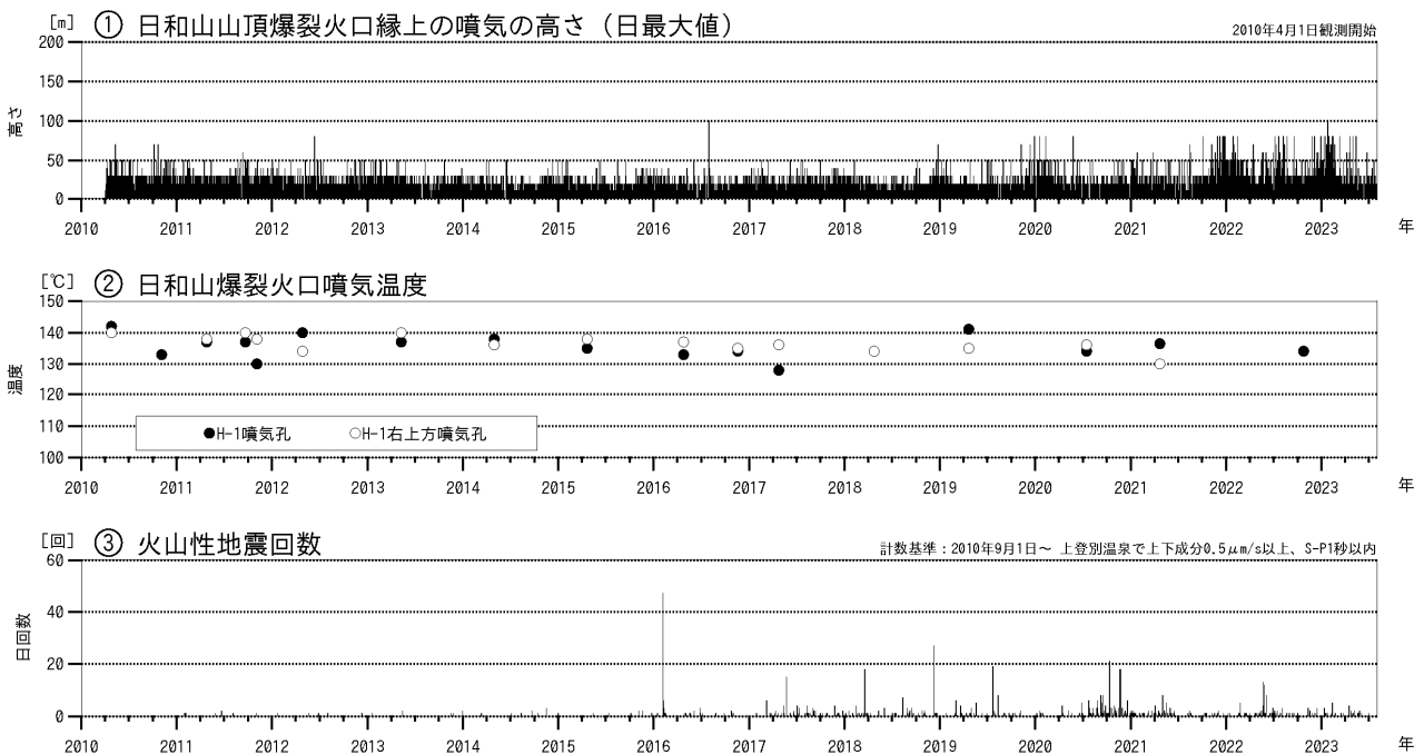
図2 倶多楽 火山活動経過図（2010年1月～2023年7月）
