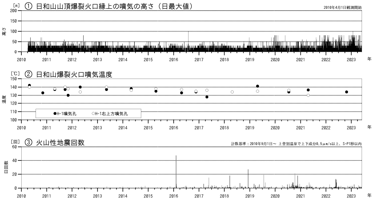
図2 倶多楽 火山活動経過図（2010年1月～2023年5月）
