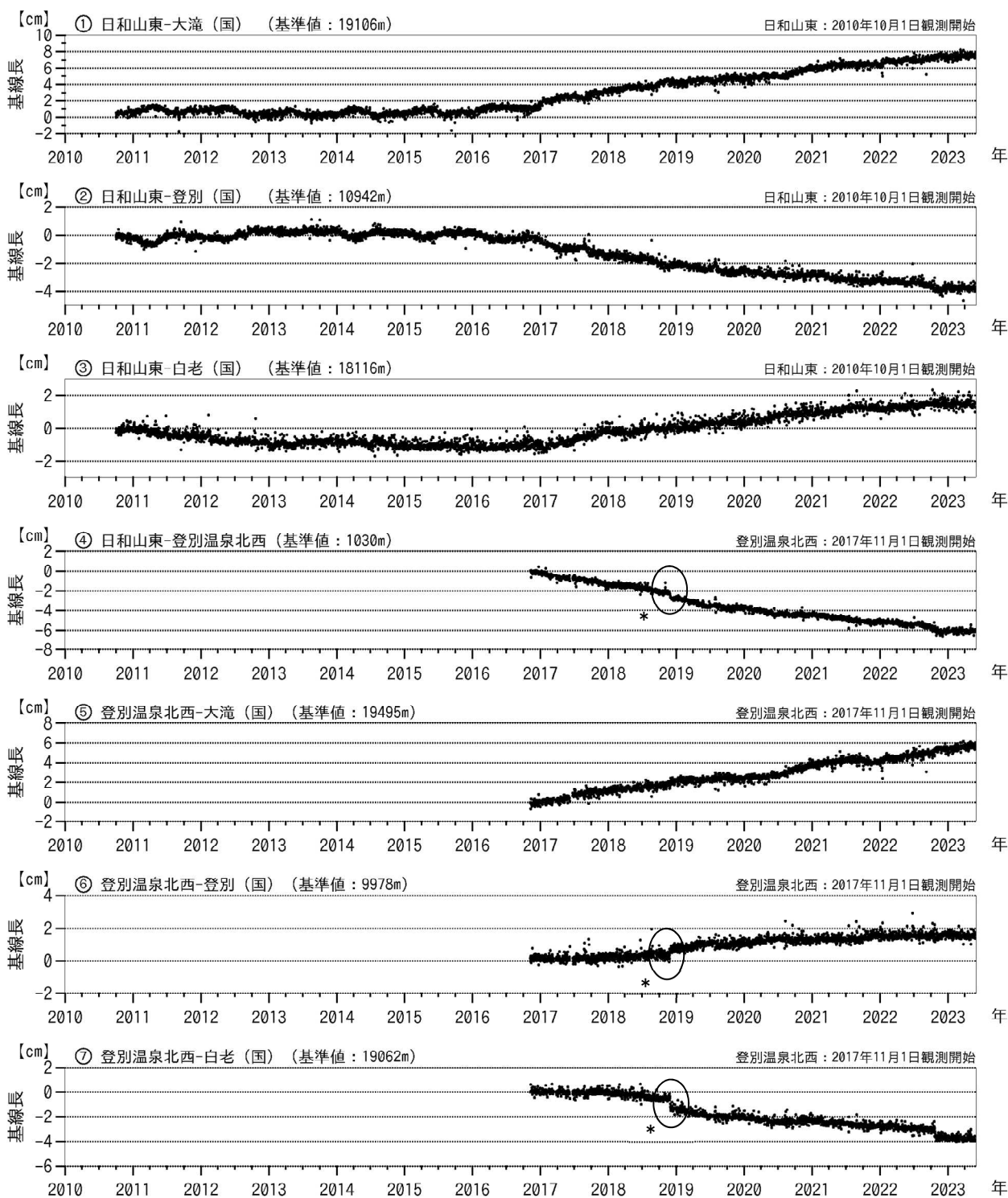
図3 倶多楽 GNSS連続観測による基線長変化 (2010年10月~2023年5月) グラフ①~⑦は観測点配置図 (図4) の基線①~⑦に対応しています。 ④、⑥及び⑦の楕円内の変動 (*) は、登別温泉北西観測点の局所的な動きによるものと 考えられます。
