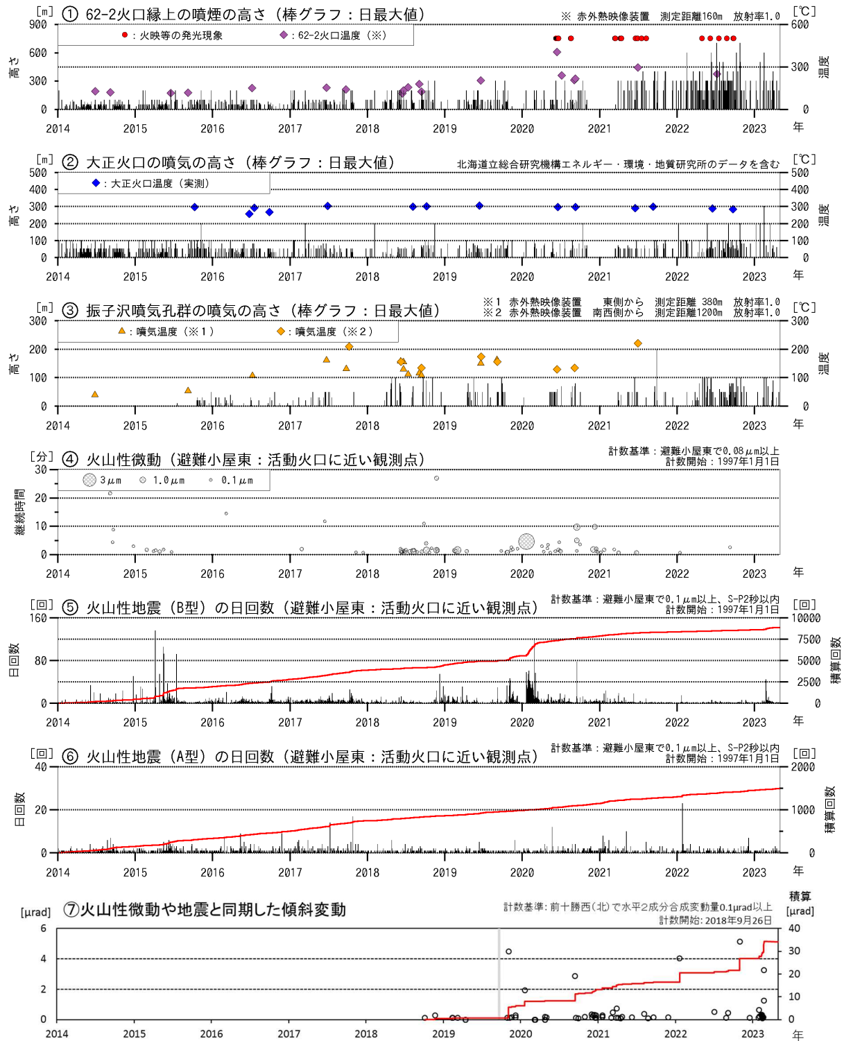
図2 十勝岳 火山活動経過図（2014年1月～2023年4月）
