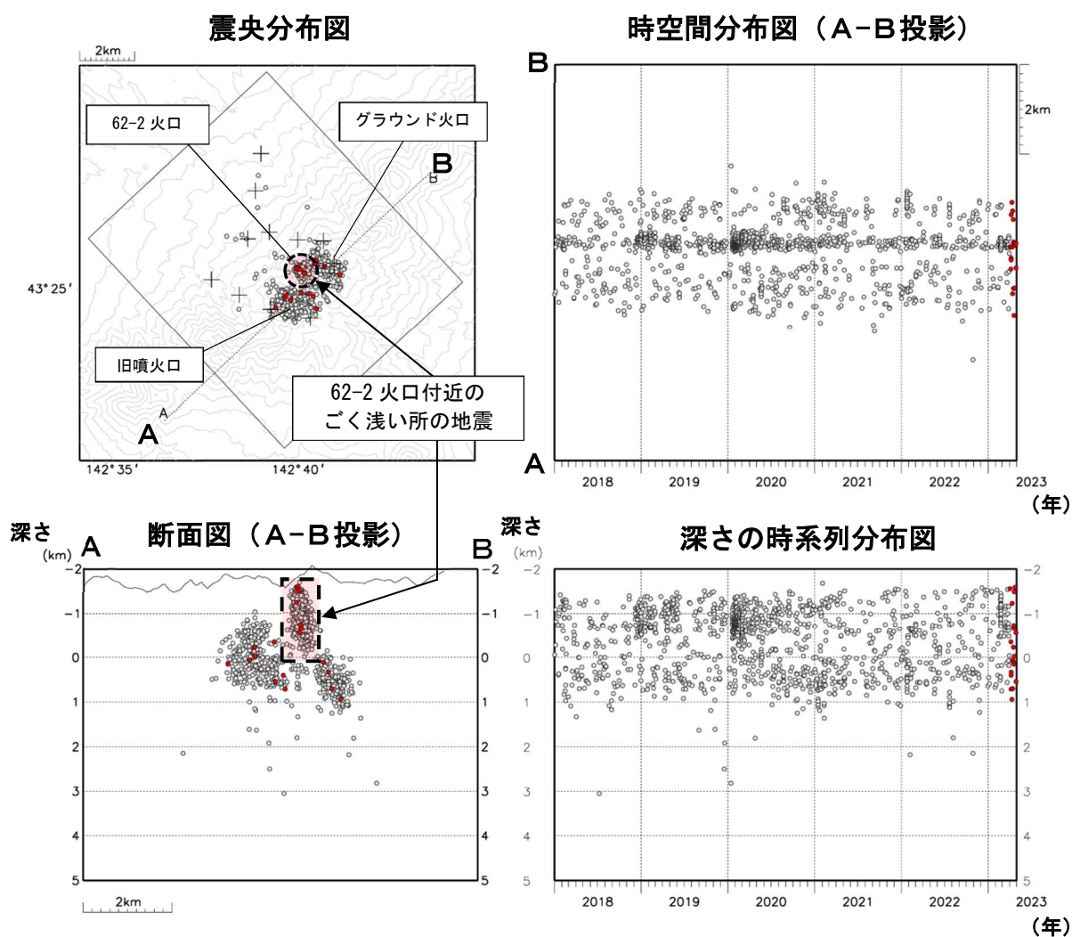
図4 十勝岳 火山性地震の震源分布（2018年1月～2023年4月）
