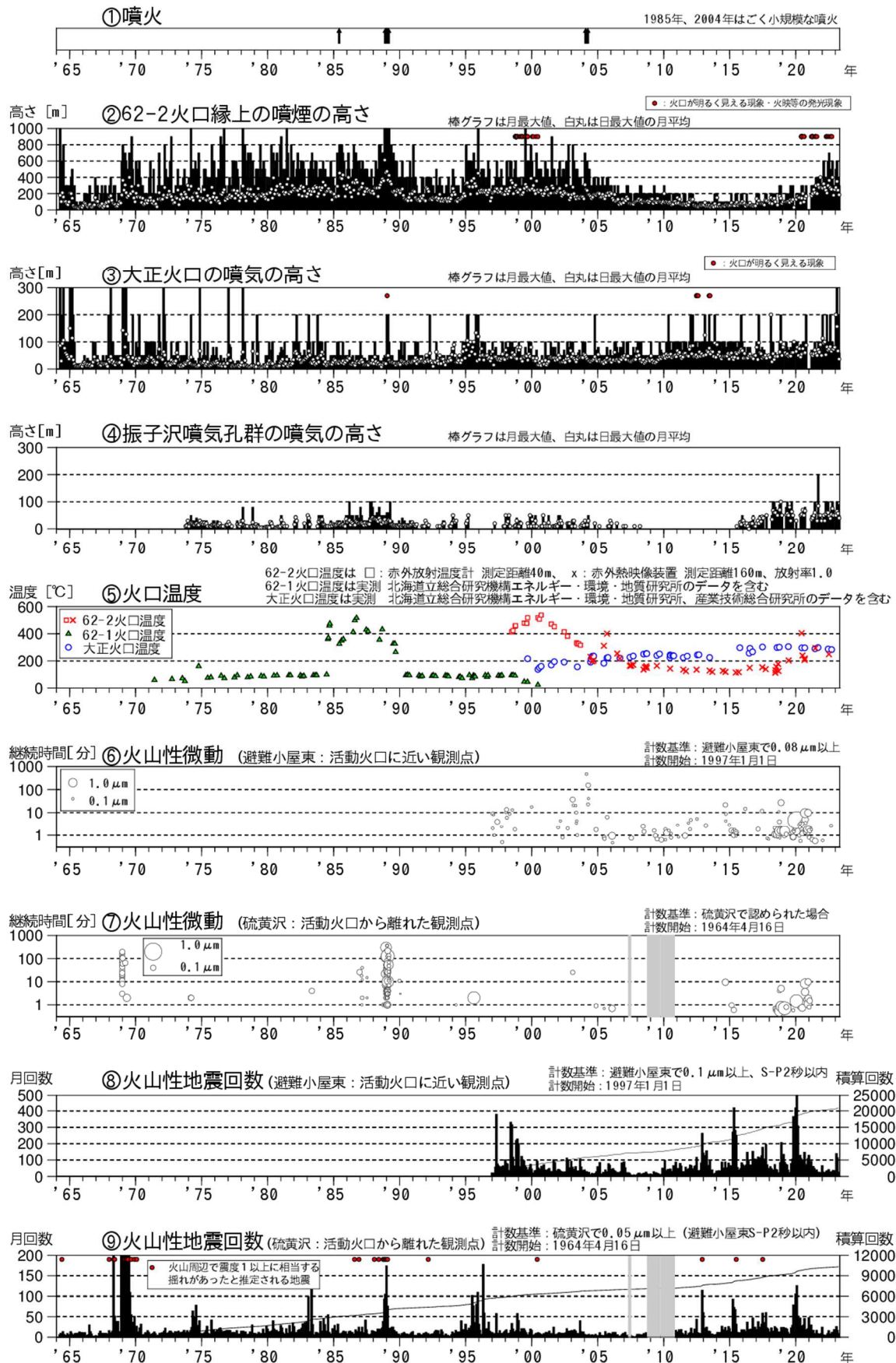
図1 十勝岳 火山活動経過図（1964年1月～2023年4月）
