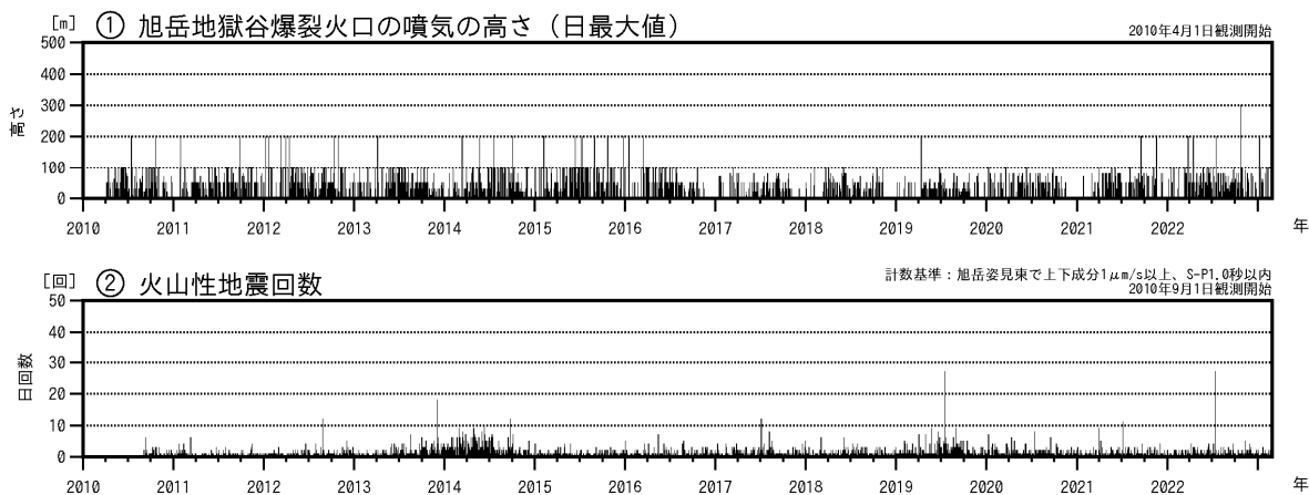
図1 大雪山 火山活動経過図（2010年4月～2023年2月）
