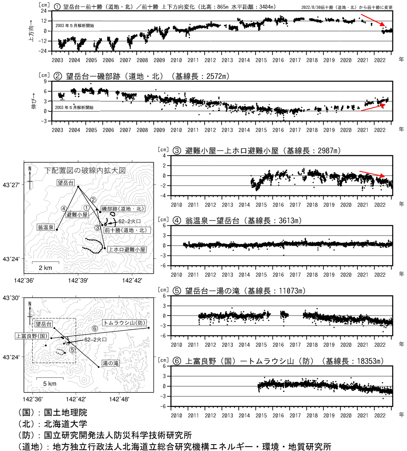
図5 十勝岳 GNSS連続観測による上下方向変化及び基線長変化（2003年5月～2023年1月）及び観測点配置図
