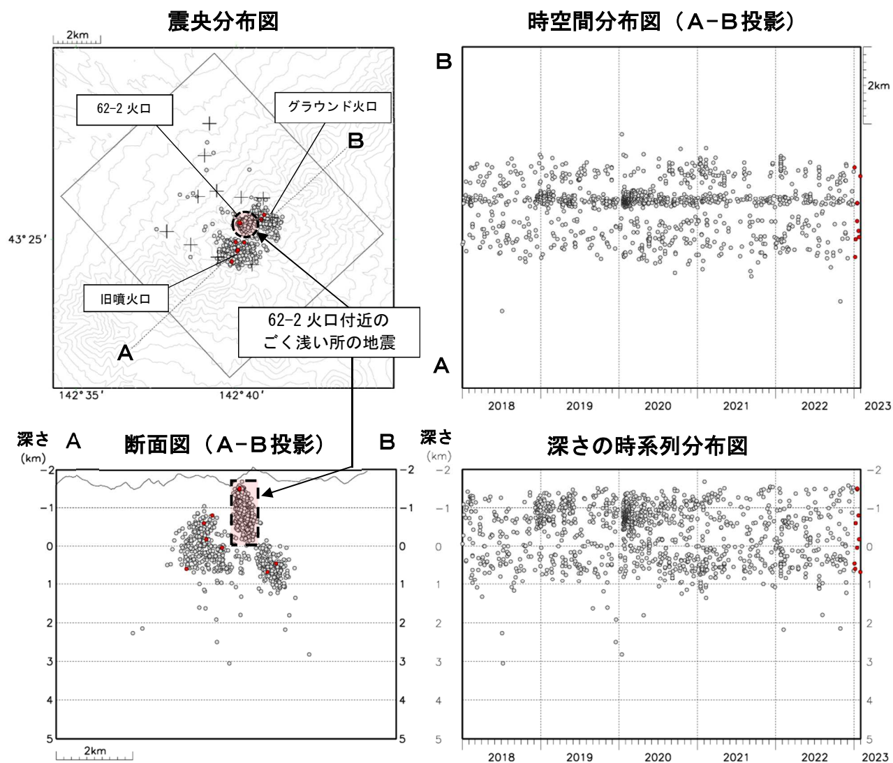
図4 十勝岳 火山性地震の震源分布（2018年1月～2023年1月） ●：2018年1月～2022年12月の震源 ●：2023年1月の震源 ＋：地震観測点
