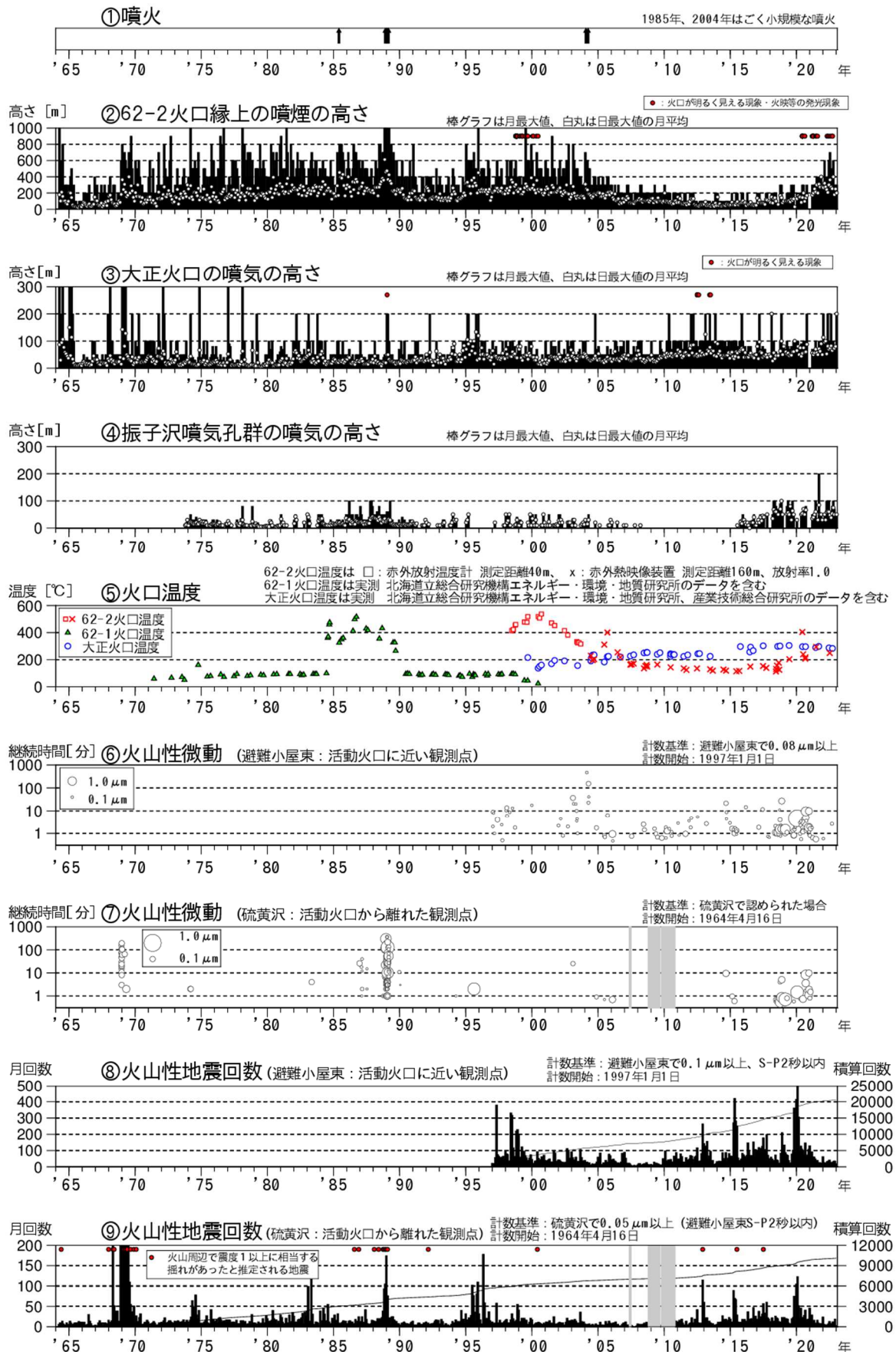
図1 十勝岳 火山活動経過図（1964年1月～2023年1月）
