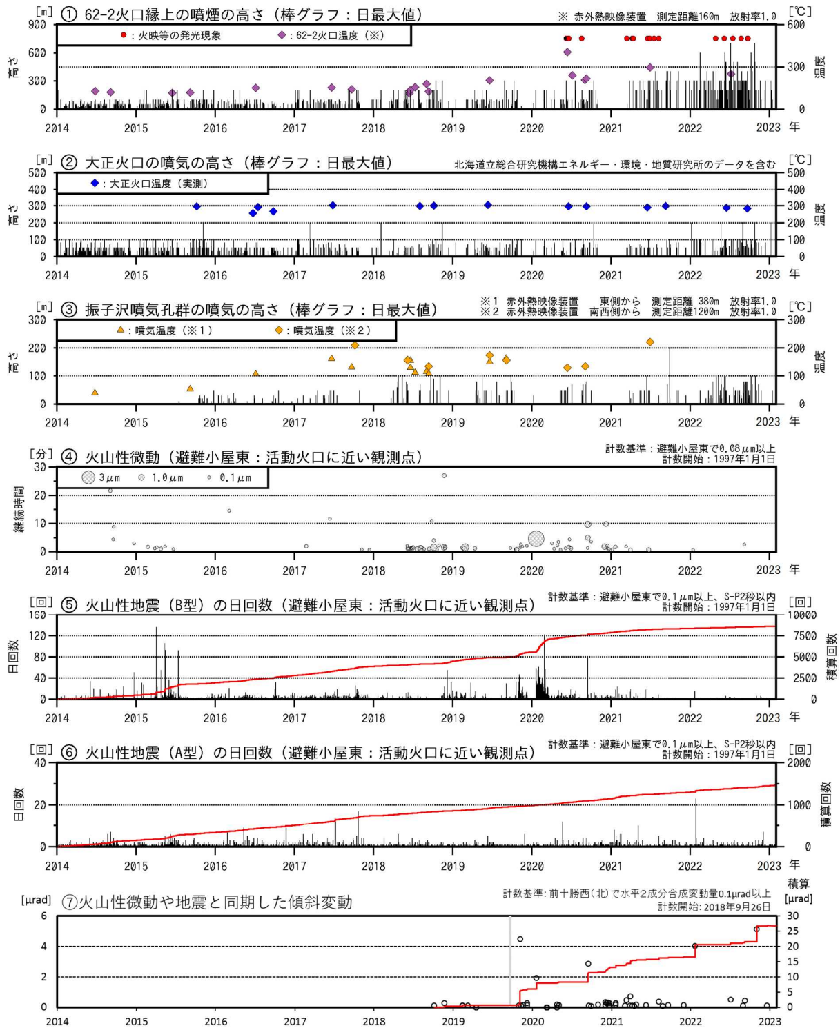
図2 十勝岳 火山活動経過図（2014年1月～2023年1月）
