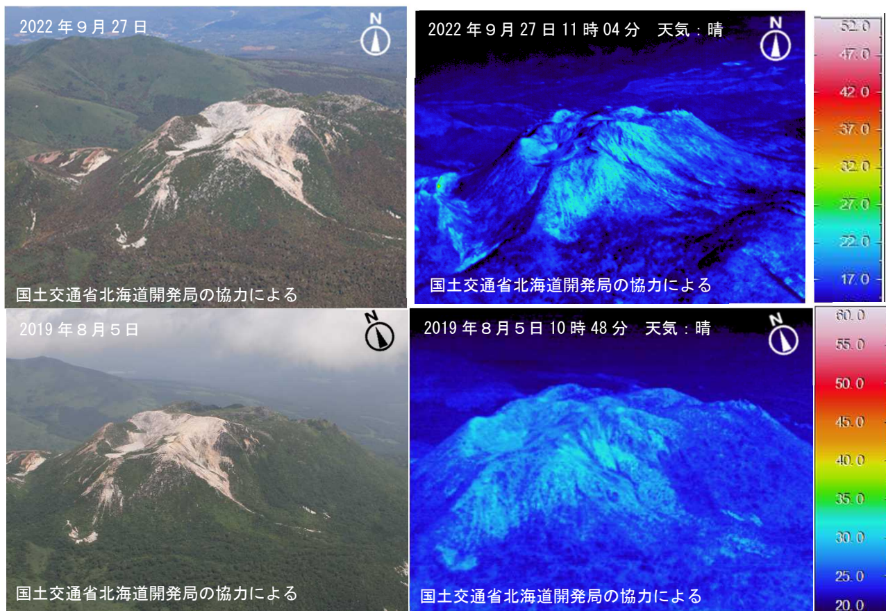
図3 ニセコ 赤外熱映像装置によるイワオヌプリ山頂部の地表面温度分布 上段：南側上空（図1の②）から撮影 下段：南南西側上空（図1の③）から撮影 ・前回の観測（2019年8月）と同様、イワオヌプリ山頂部には噴気や地熱域は認められませんでした（一部領域で周囲に比べて温度が高く見えるのは日射による影響と考えられます）。
