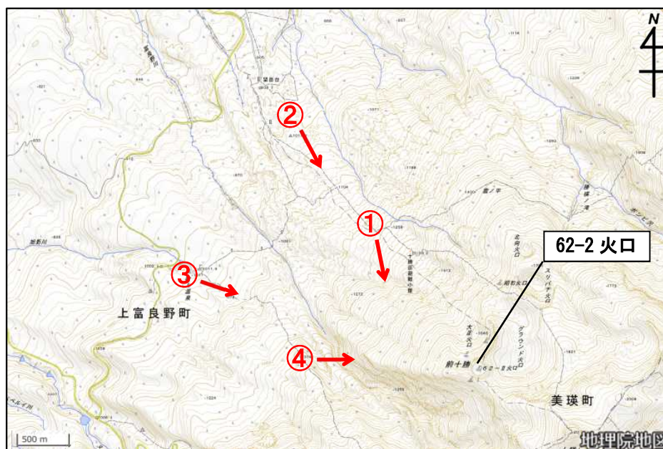
図5 十勝岳 写真及び赤外熱映像の撮影方向（矢印）
