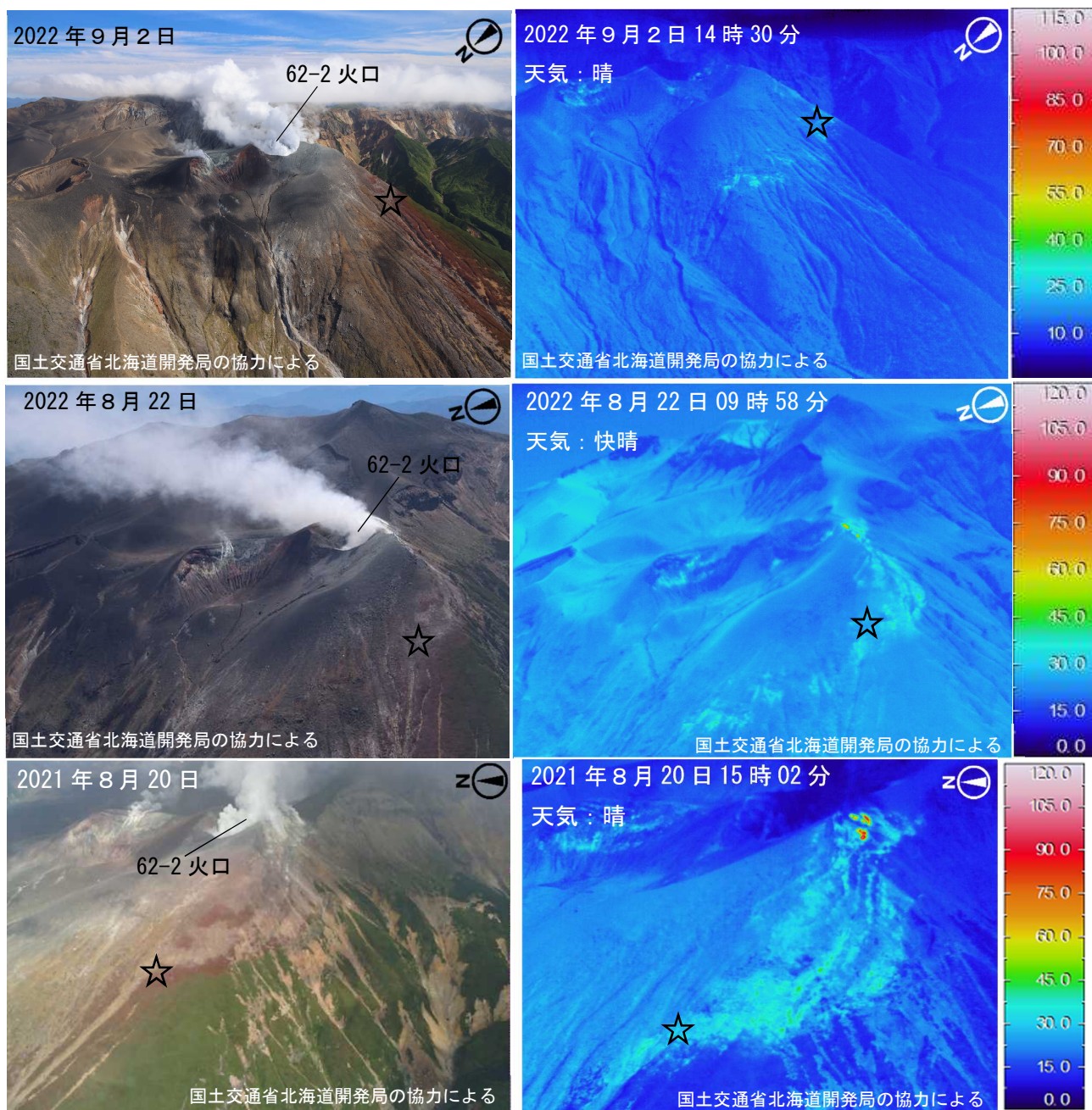
図6 十勝岳 赤外熱映像装置による前十勝北西側の地表面温度分布
