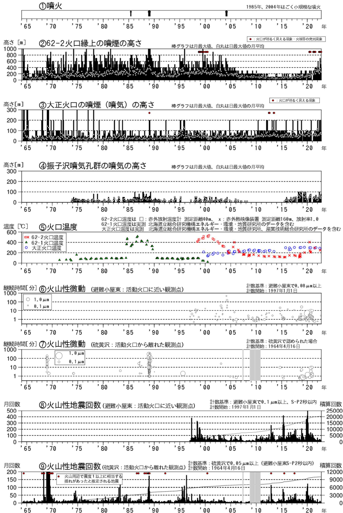
図1 十勝岳 火山活動経過図（1964年1月～2022年9月）
