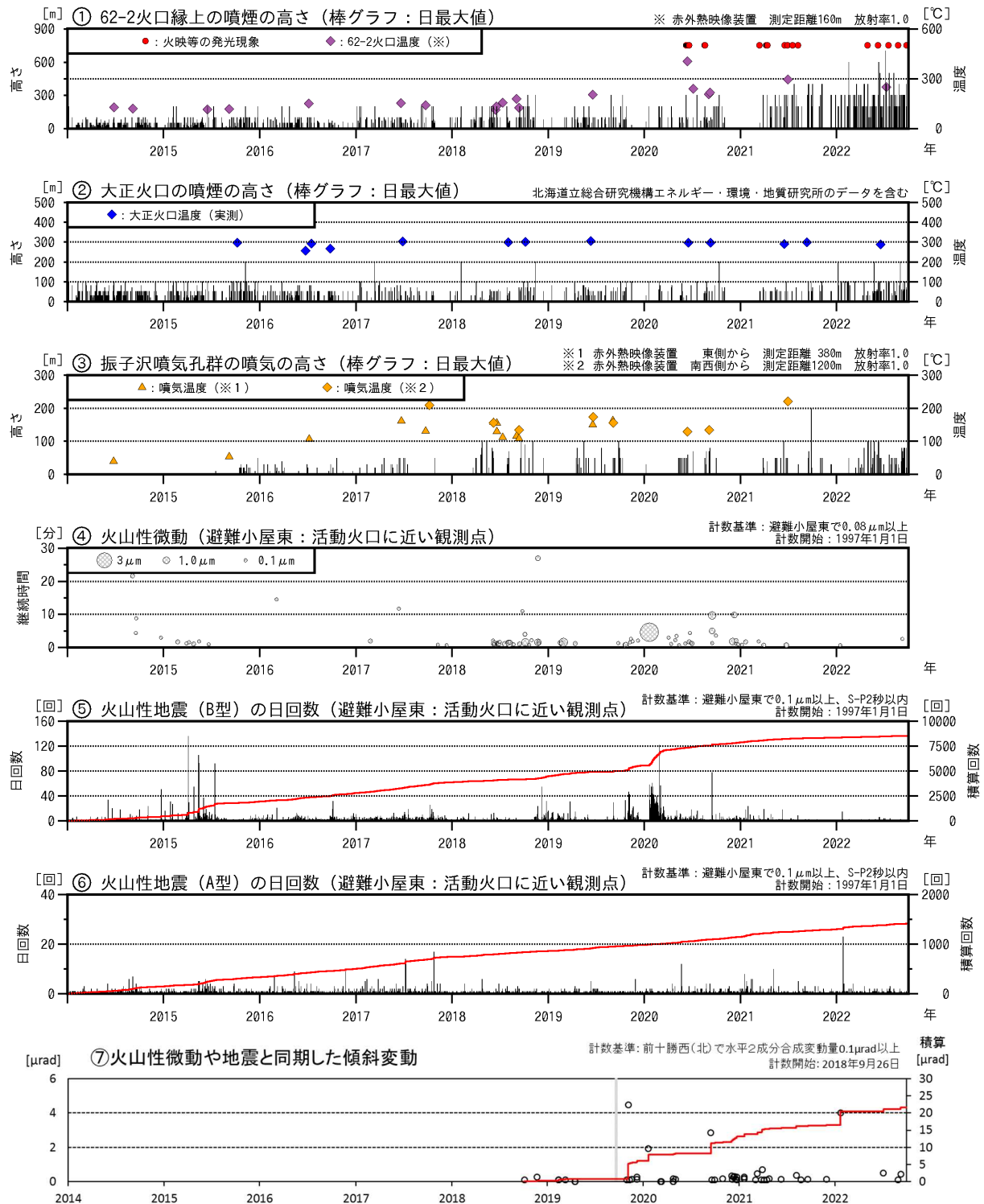
図2 十勝岳 火山活動経過図（2014年1月～2022年9月）
