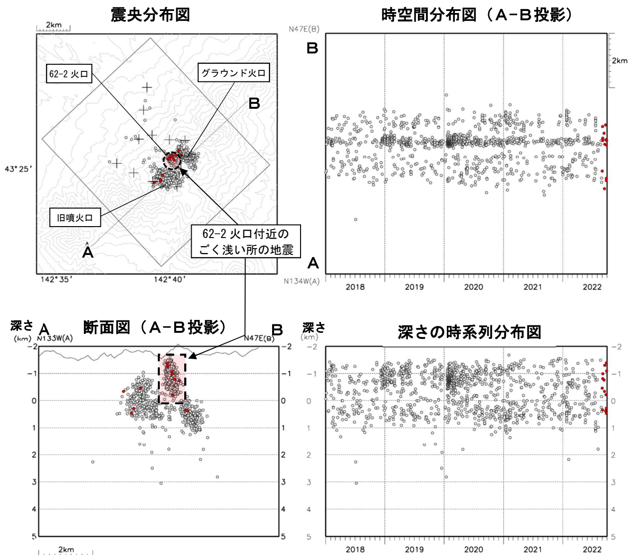
図7 十勝岳 火山性地震の震源分布（2018年1月～2022年9月）
