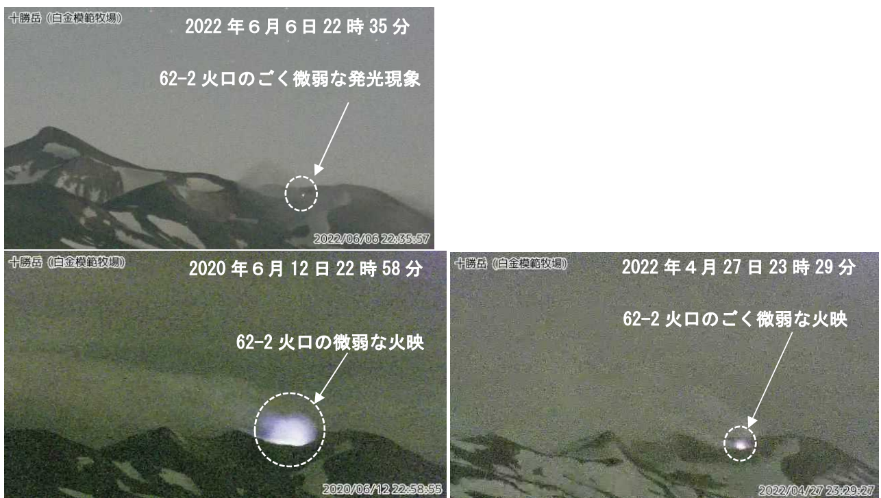
図4 十勝岳 62-2 火口で観測されたごく微弱な発光現象（白金模範牧場監視カメラによる） 撮影方向は図3と同様
