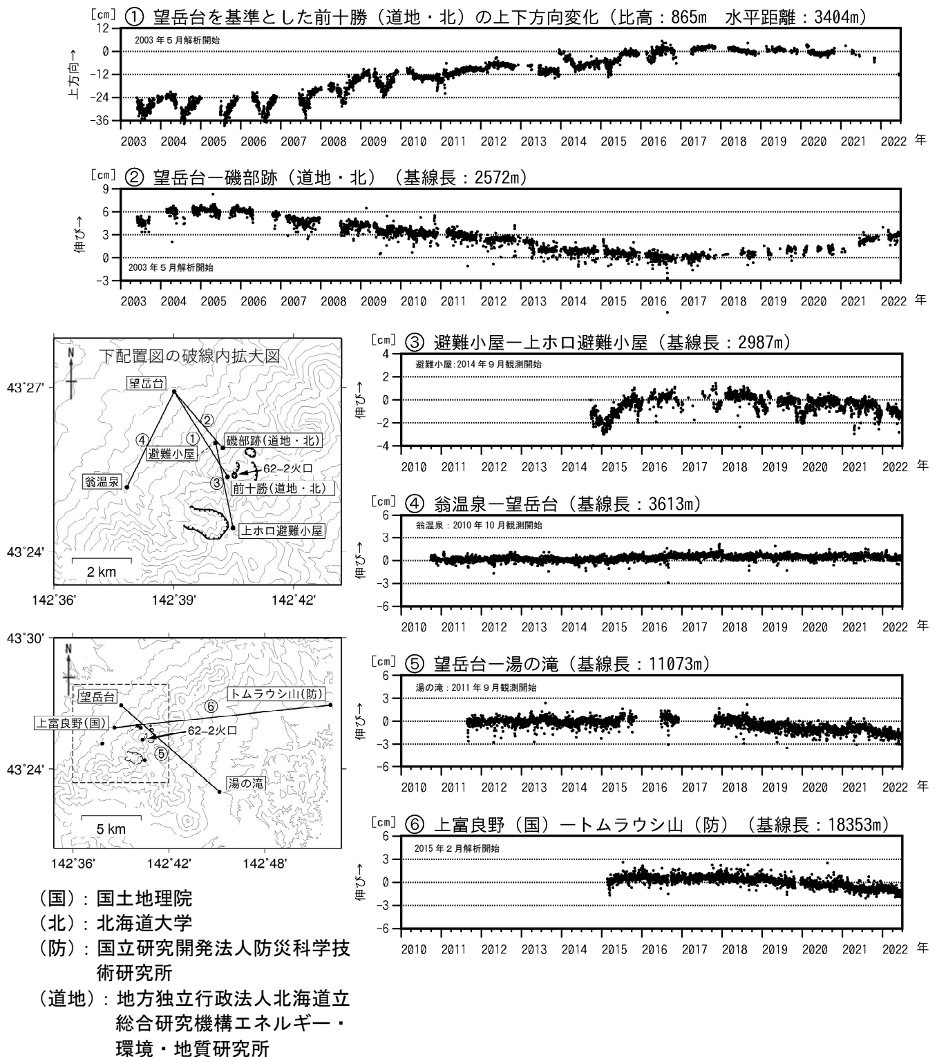
図7 十勝岳 GNSS連続観測による上下方向変化及び基線長変化（2003年5月～2022年6月）及び観測点配置図
