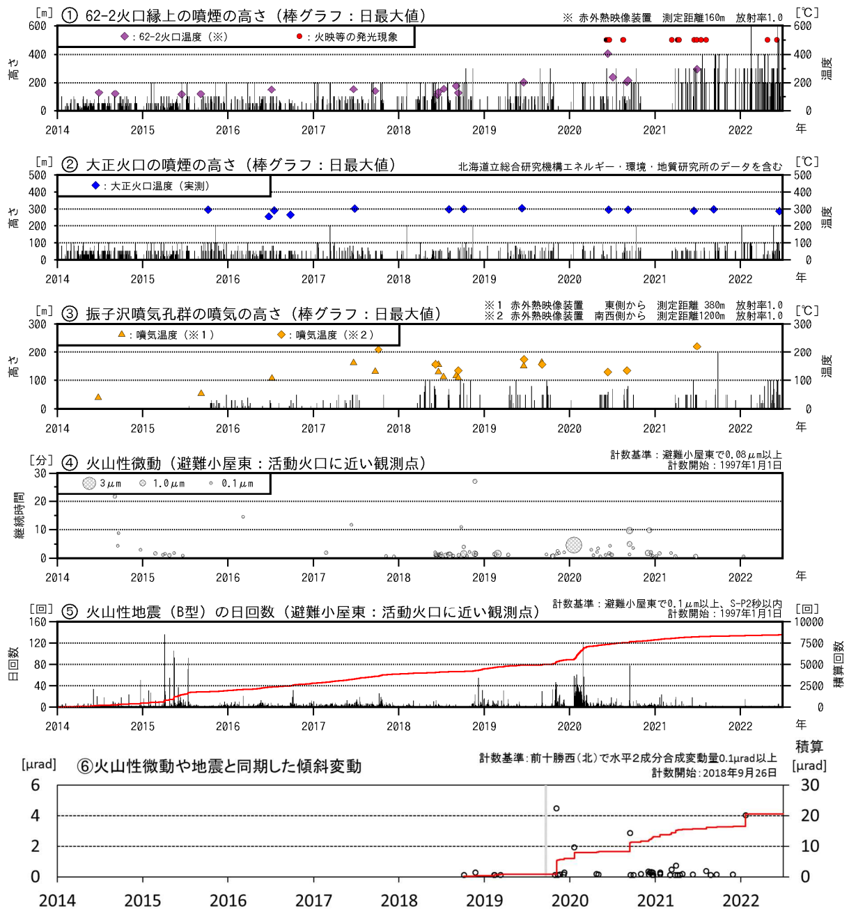
図2 十勝岳 火山活動経過図（2014年1月～2022年6月）
