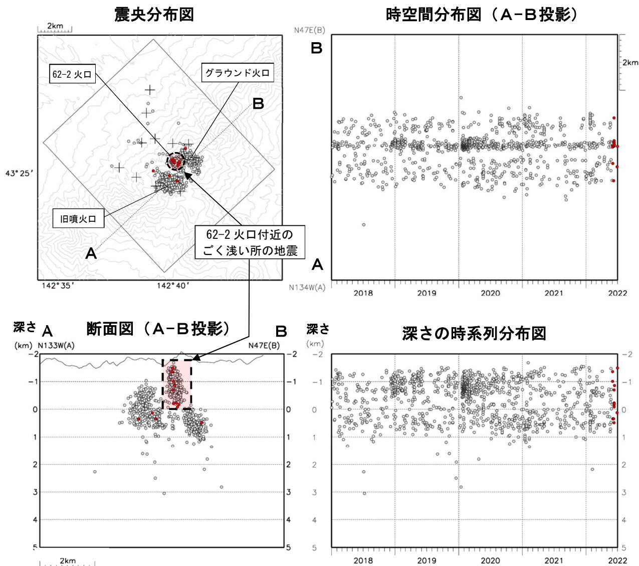
図5 十勝岳 火山性地震の震源分布（2018年1月～2022年6月）
