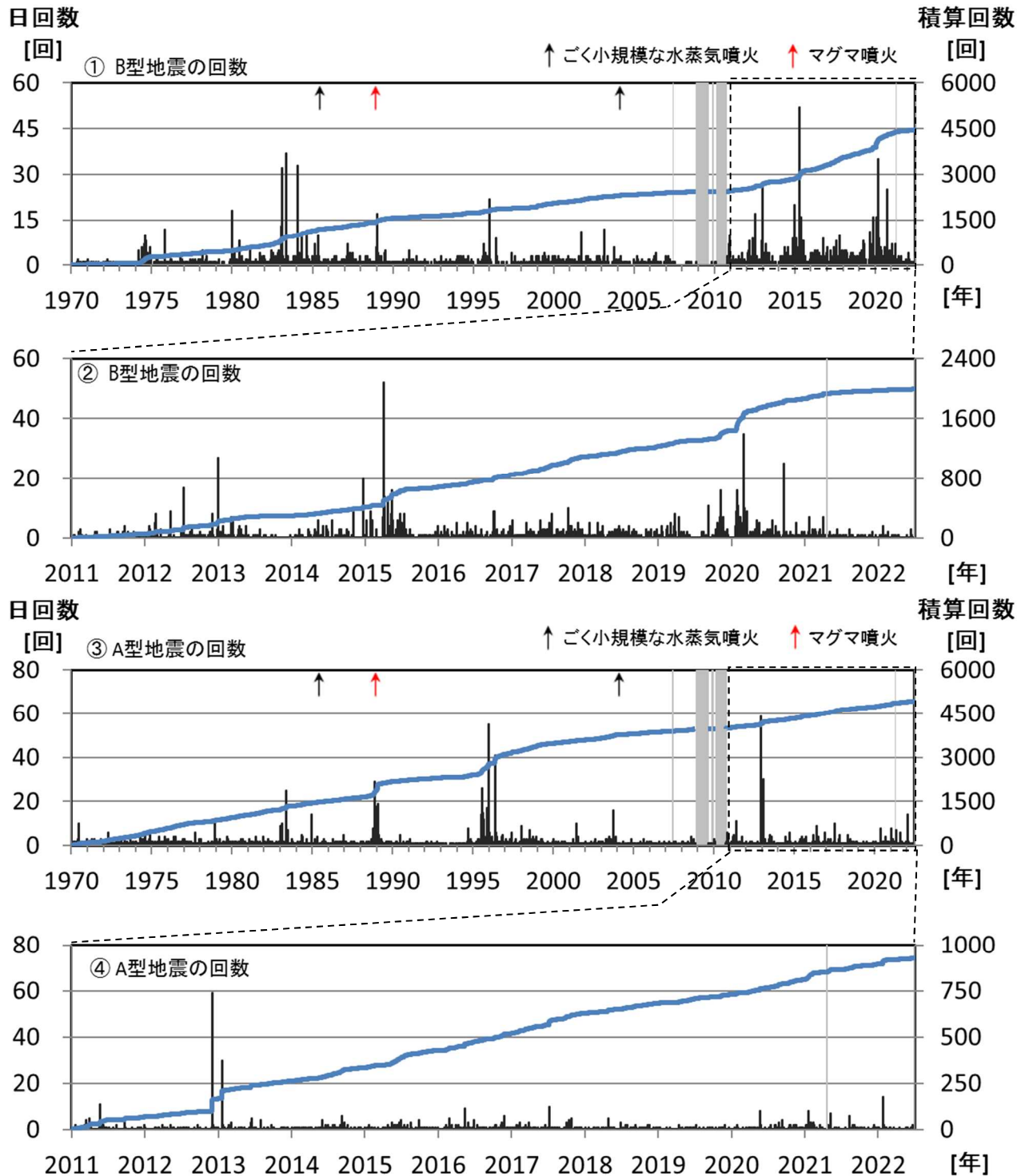
図6 十勝岳 地震の日回数及び積算回数（①③：1970年～2022年6月 ②④：2011年～2022年6月） 硫黄沢観測点（山麓点）で計測した回数（計数基準：0.05 \mu m以上）を示します。 B型地震①②は主に62-2火口付近のごく浅い所、A型地震③④は主にグラウンド火口周辺や旧噴火口 付近で発生したと推測されます。 図中の青線は積算回数を示し、灰色の部分は欠測を示します。
