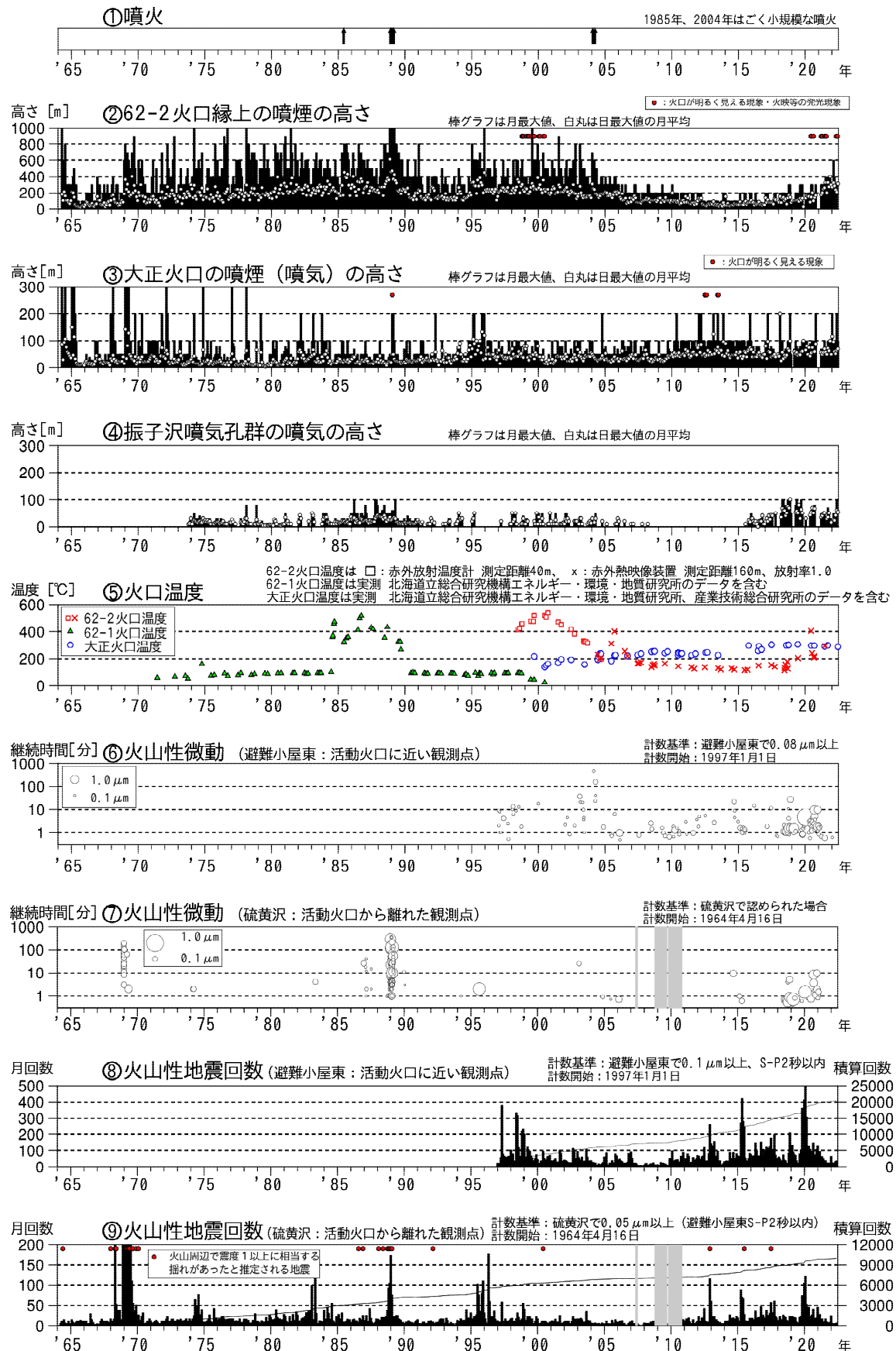
図1 十勝岳 火山活動経過図（1964年1月～2022年6月）
