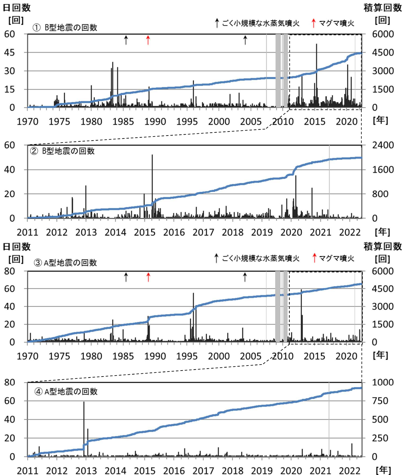
図5 十勝岳 地震の日回数及び積算回数（①③：1970年～2022年5月 ②④：2011年～2022年5月） 硫黄沢観測点（山麓点）で計測した回数（計数基準：0.05 \mu m以上）を示します。 B型地震①②は主に62-2火口付近のごく浅い所、A型地震③④は主にグラウンド火口周辺や旧噴火口 付近で発生したと推測されます。 図中の青線は積算回数を示し、灰色の部分は欠測を示します。
