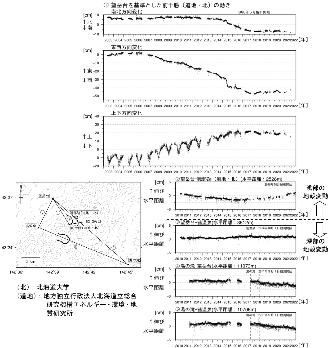
図6 十勝岳 GNSS連続観測による南北・東西・上下方向変化及び水平距離変化（2003年5月～2022年5月）及び観測点配置図
