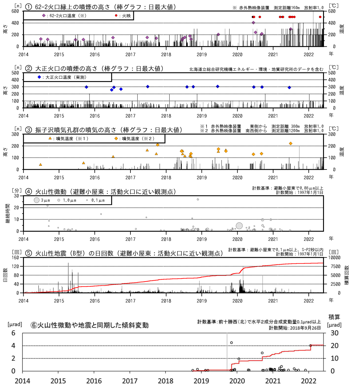
図2 十勝岳 火山活動経過図（2014年1月～2022年5月）
