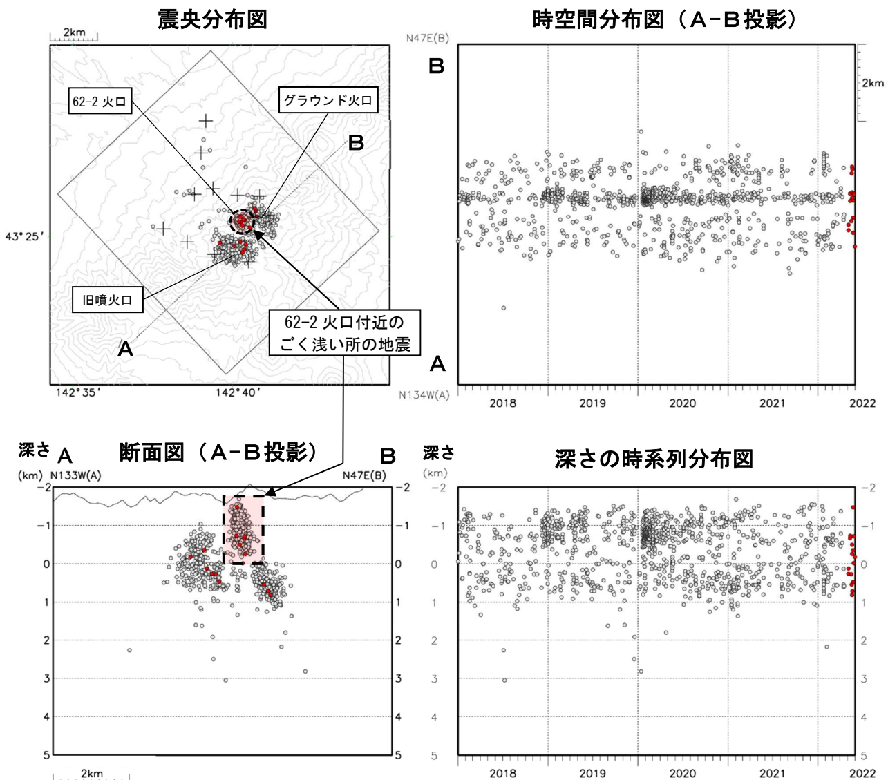
図4 十勝岳 火山性地震の震源分布（2018年1月～2022年5月）
