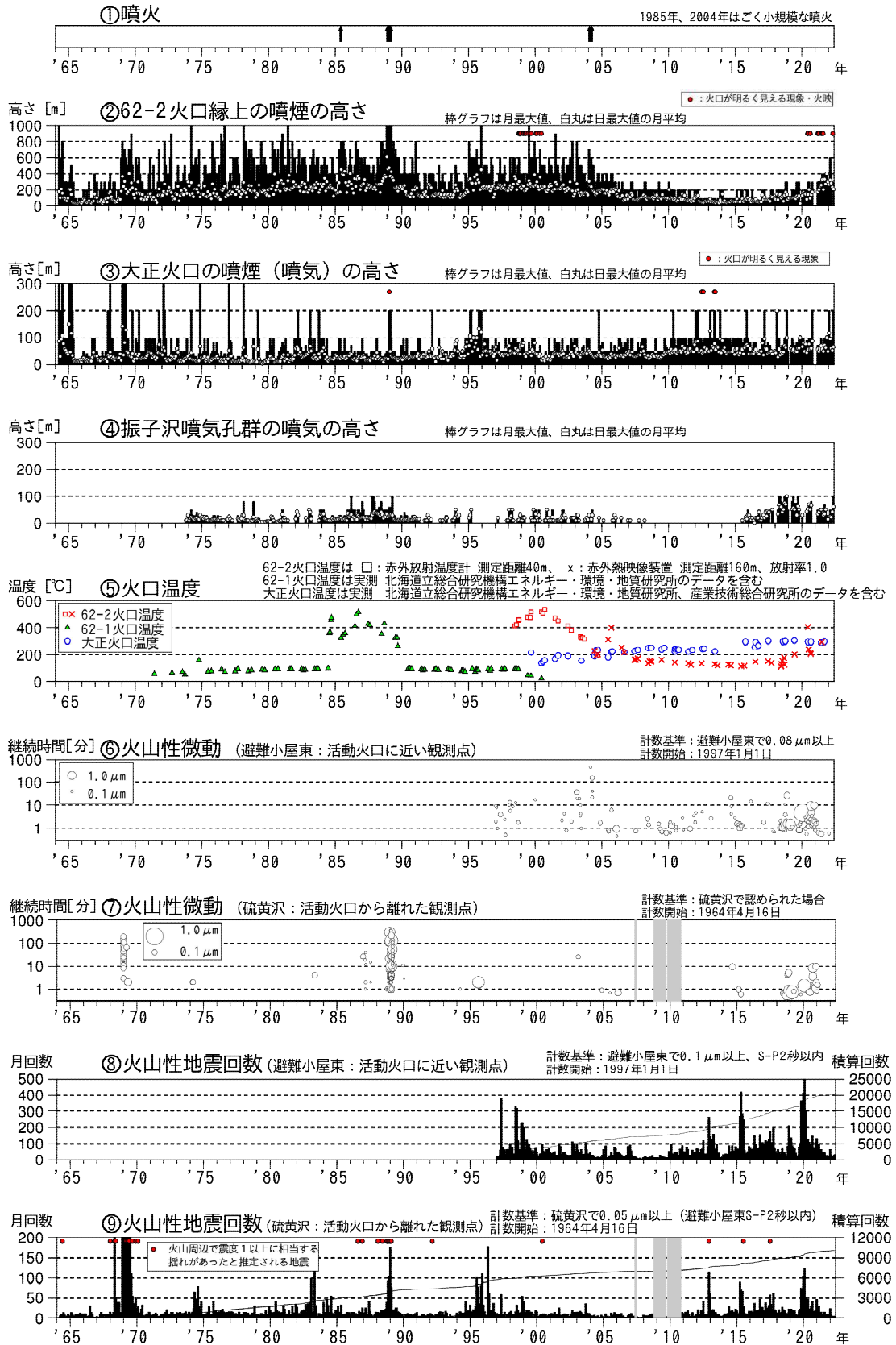
図1 十勝岳 火山活動経過図 (1964年1月~2022年5月) ⑦⑨の灰色部分は機器障害による欠測期間を示します。
