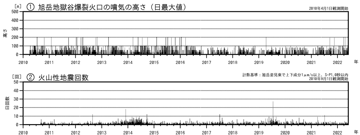
図1 大雪山 火山活動経過図（2010年4月～2022年5月）
