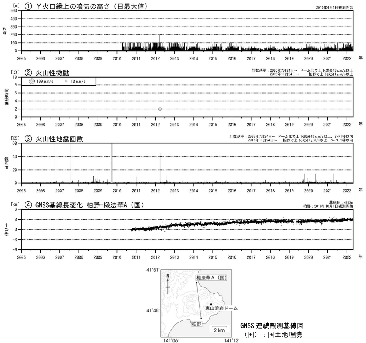
図2 恵山 火山活動経過図（2005年7月～2022年4月） ③の灰色部分は機器障害による欠測期間を示します。 ④のグラフは上図の基線に対応しています。 ④のグラフの空白部分は欠測を示します。
