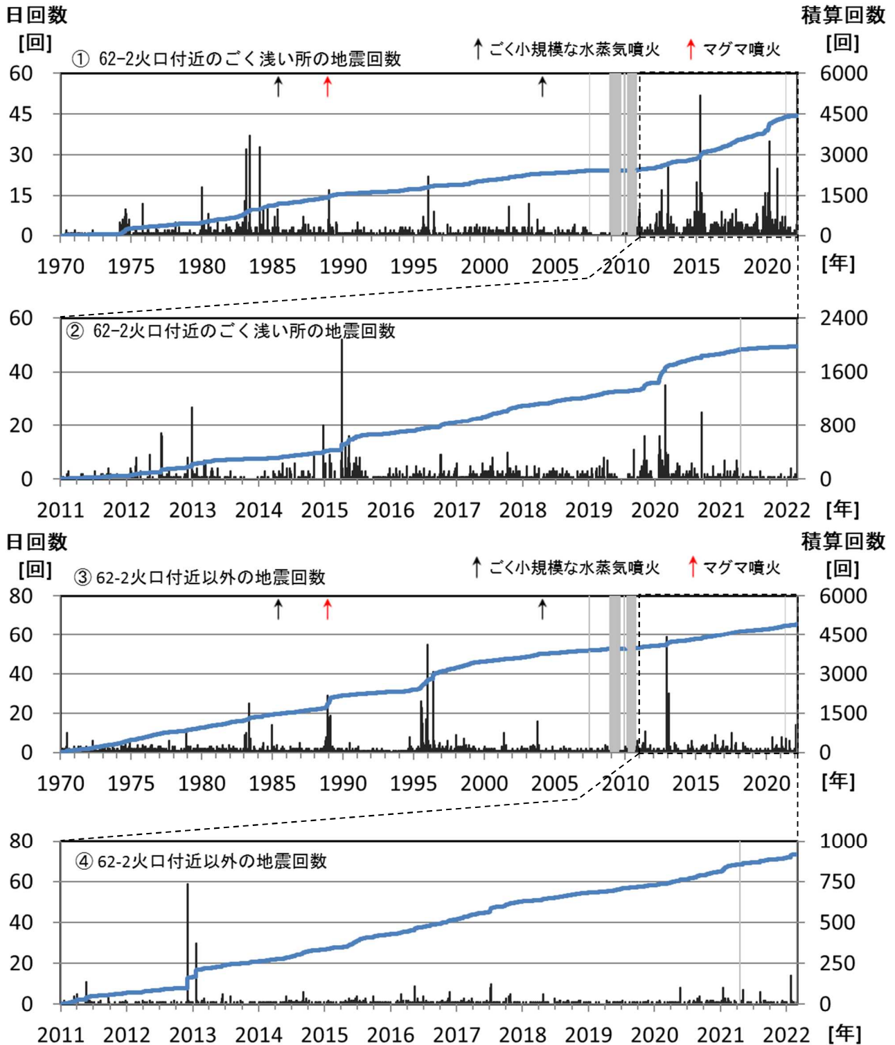
図5 十勝岳 地震の日回数及び積算回数（①③：1970年～2022年2月 ②④：2011年～2022年2月） 硫黄沢観測点（山麓点）で計測した回数（計数基準： 0.05\mu\text{m} 以上）を示します。 ①、②は主に62-2火口付近のごく浅い所（図4中の破線に囲まれた領域内）で発生したと推測される地震の回数を示します。また③、④の「62-2火口付近以外」は、主にグラウンド火口周辺や旧噴火口付近などで発生したと推測される地震の回数を示します。 図中の、青線は積算回数を示し、灰色の部分は欠測を示します。
