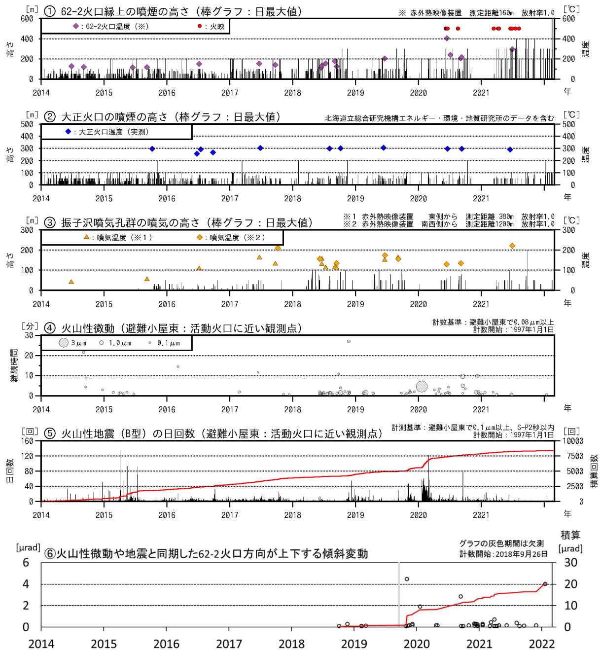
図2 十勝岳 火山活動経過図（2014年1月～2022年2月）
