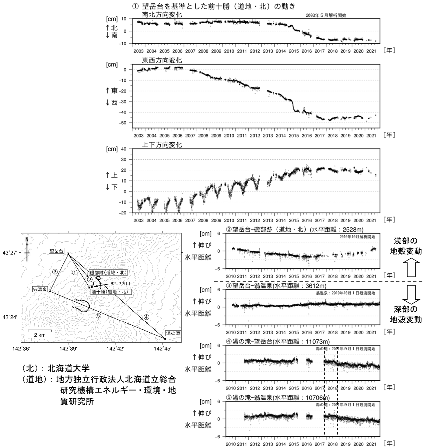
図6 十勝岳 GNSS連続観測による南北・東西・上下方向変化及び水平距離変化（2003年5月～2022年2月）及び観測点配置図
