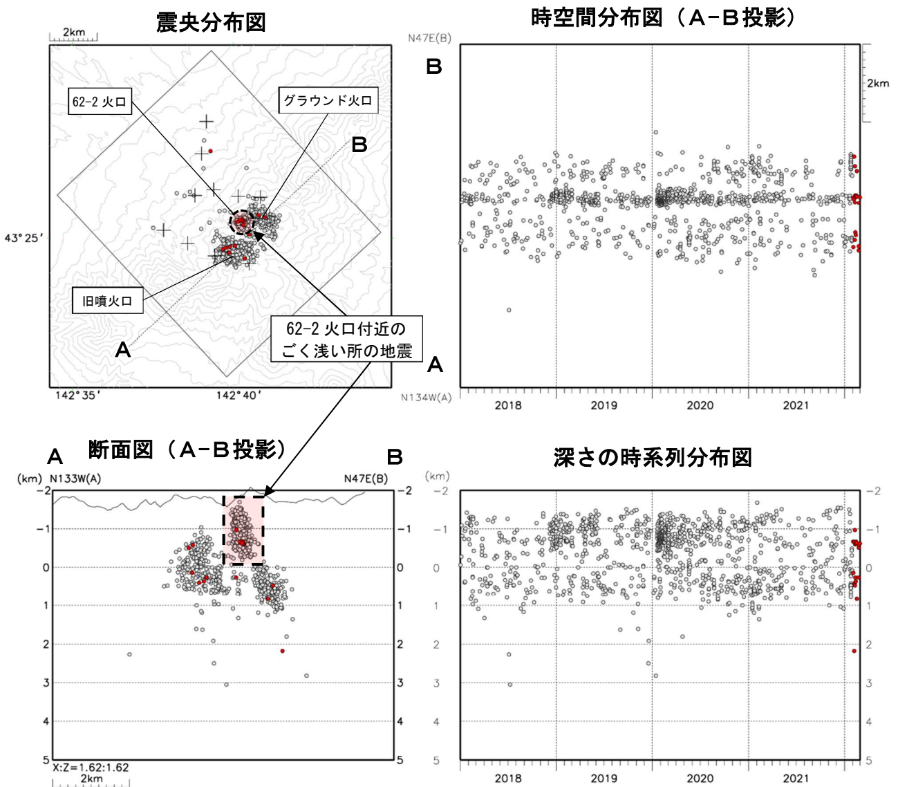
図4 十勝岳 火山性地震の震源分布（2018年1月～2022年2月） ●：2018年1月～2022年1月の震源 ●：2022年2月の震源 ＋：地震観測点
