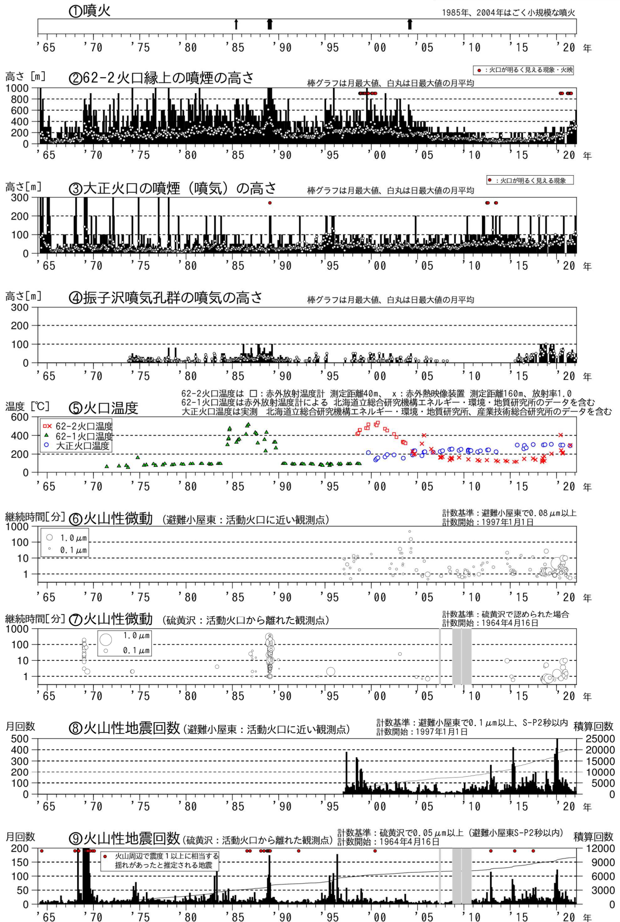
図1 十勝岳 火山活動経過図（1964年1月～2022年2月）
