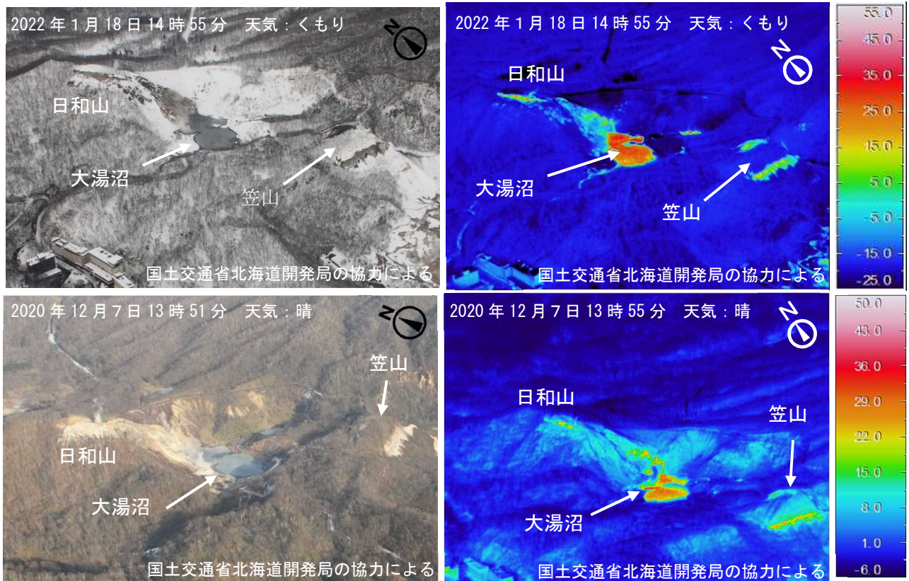
図4 倶多楽 赤外熱映像装置による日和山・大湯沼・笠山周辺の地表面温度分布
