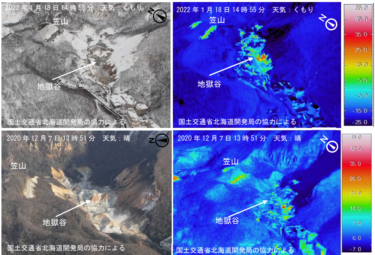
図5 倶多楽 赤外熱映像装置による地獄谷の地表面温度分布 上：南西側上空（図3の④）から撮影 左下：西側上空（図3の⑤）から撮影 右下：南西側上空（図3の⑥）から撮影 ・地獄谷の噴気の状況や地表面温度分布に特段の変化は認められませんでした。
