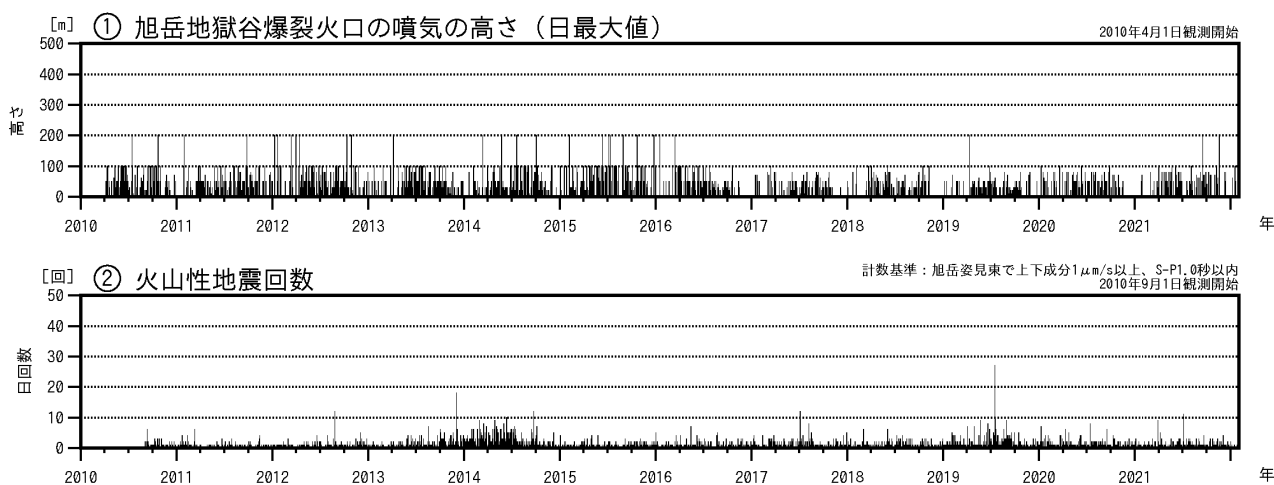
図1 大雪山 火山活動経過図（2010年4月～2022年1月）
