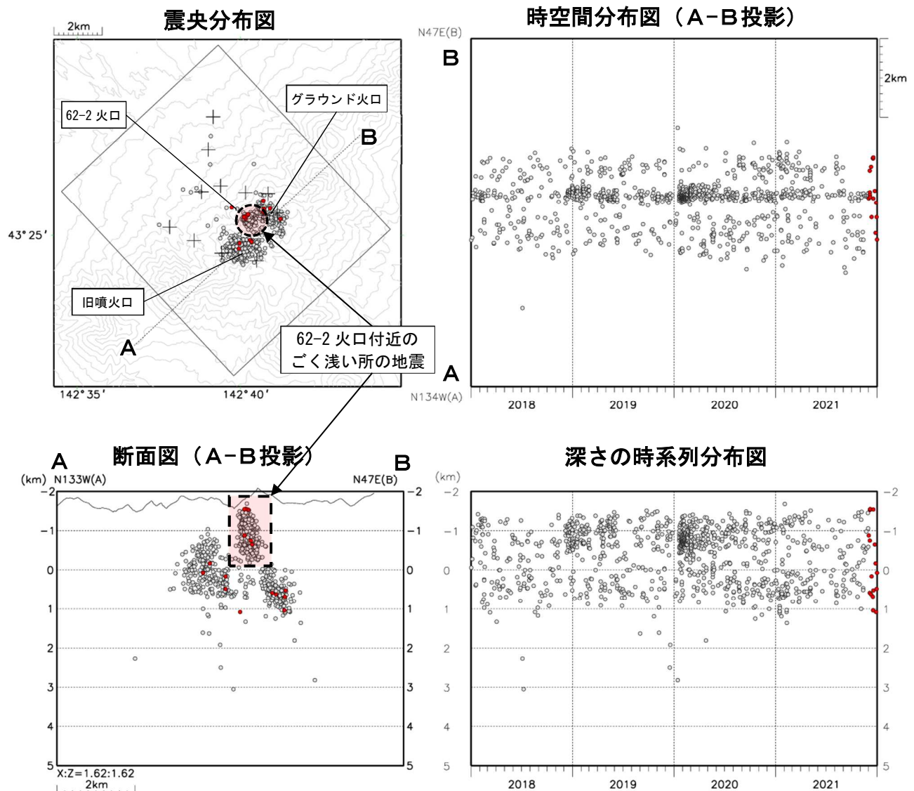
図4 十勝岳 火山性地震の震源分布（2018年1月～2021年12月） ●: 2018年1月～2021年11月の震源 ●: 2021年12月の震源 +: 地震観測点
