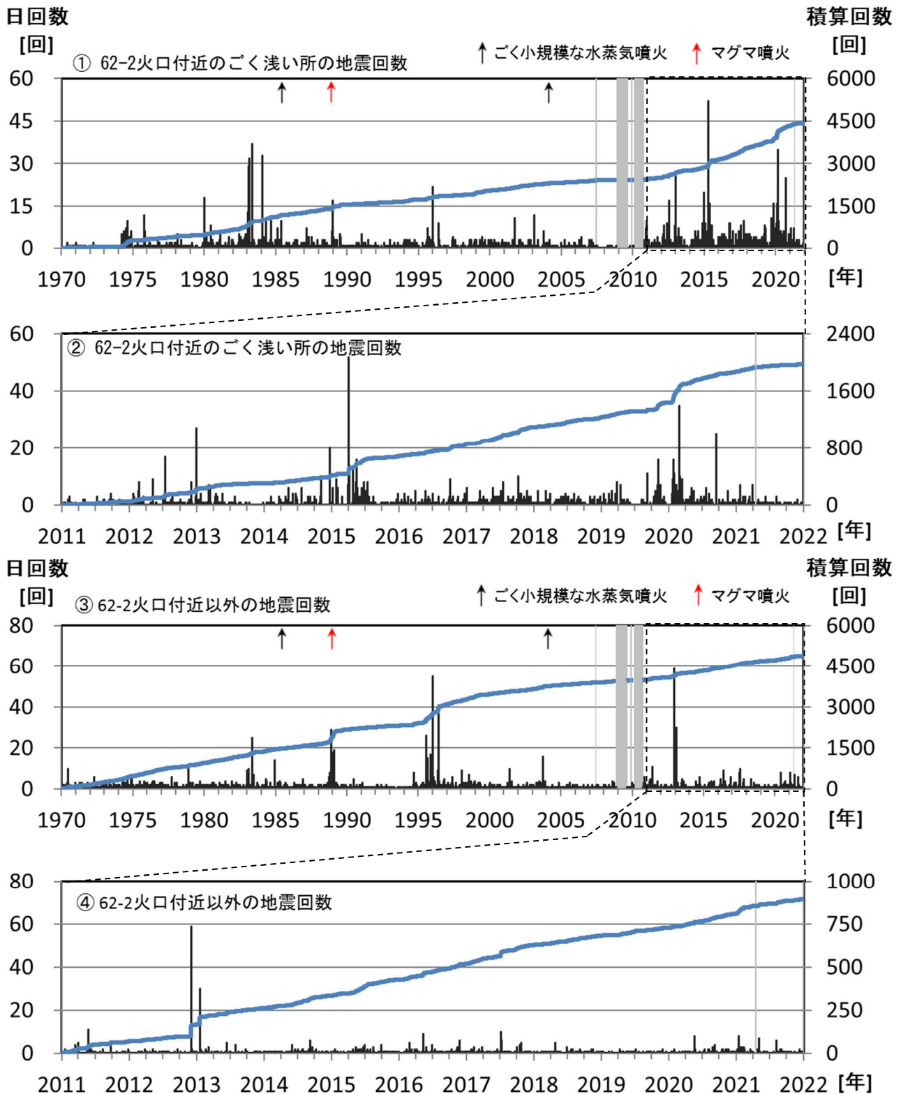
図5 十勝岳 地震の日回数及び積算回数（①③：1970年～2021年12月 ②④：2011年～2021年12月） 硫黄沢観測点（山麓点）で計測した回数（計数基準：0.05 \mu m以上）を示します。 ①、②は主に62-2火口付近のごく浅い所（図4中の破線に囲まれた領域内）で発生したと推測されるB型地震の回数を示します。また③、④の「62-2火口付近以外」は、主にグラウンド火口周辺や旧噴火口付近などで発生したと推測されるA型地震の回数を示します。 図中の、青線は積算回数を示し、灰色の部分欠測を示します。
