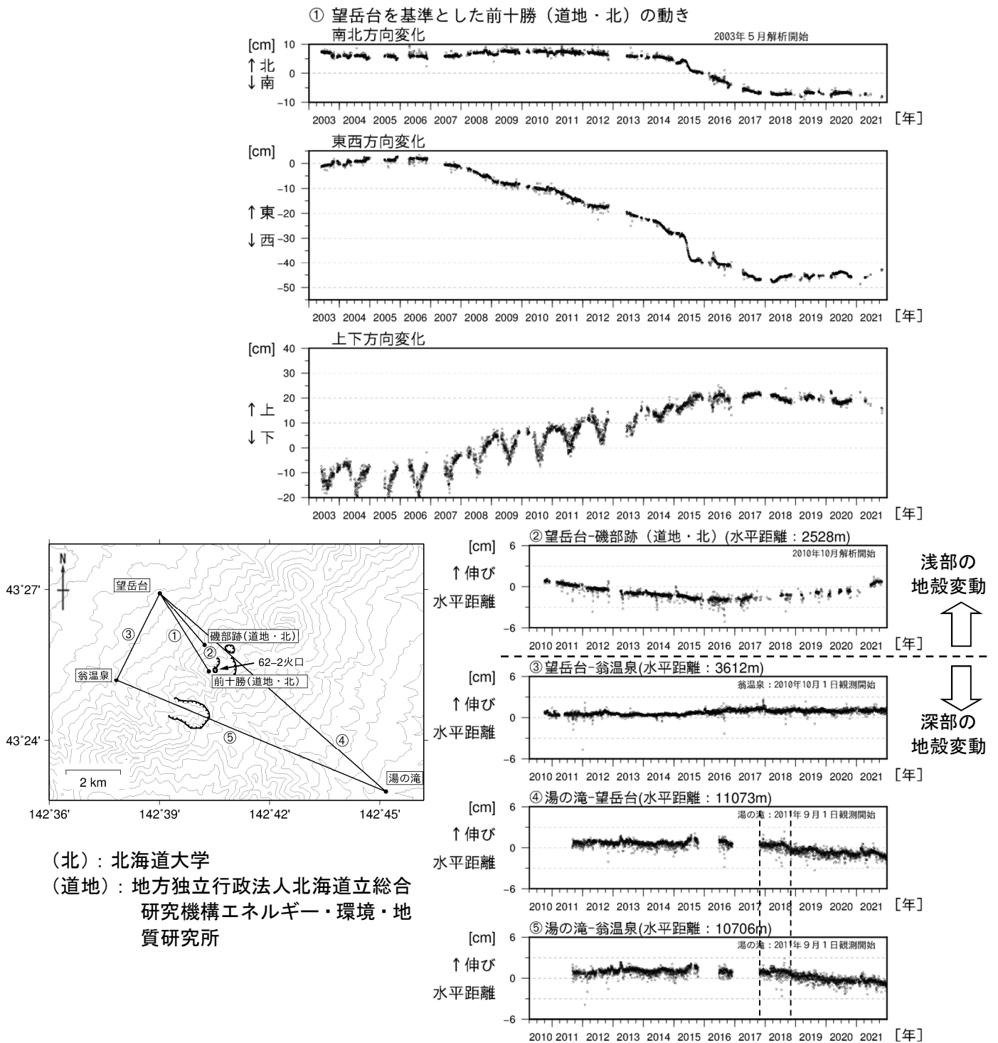
図6 十勝岳 GNSS連続観測による南北・東西・上下方向変化及び水平距離変化（2003年5月～2021年12月）及び観測点配置図
