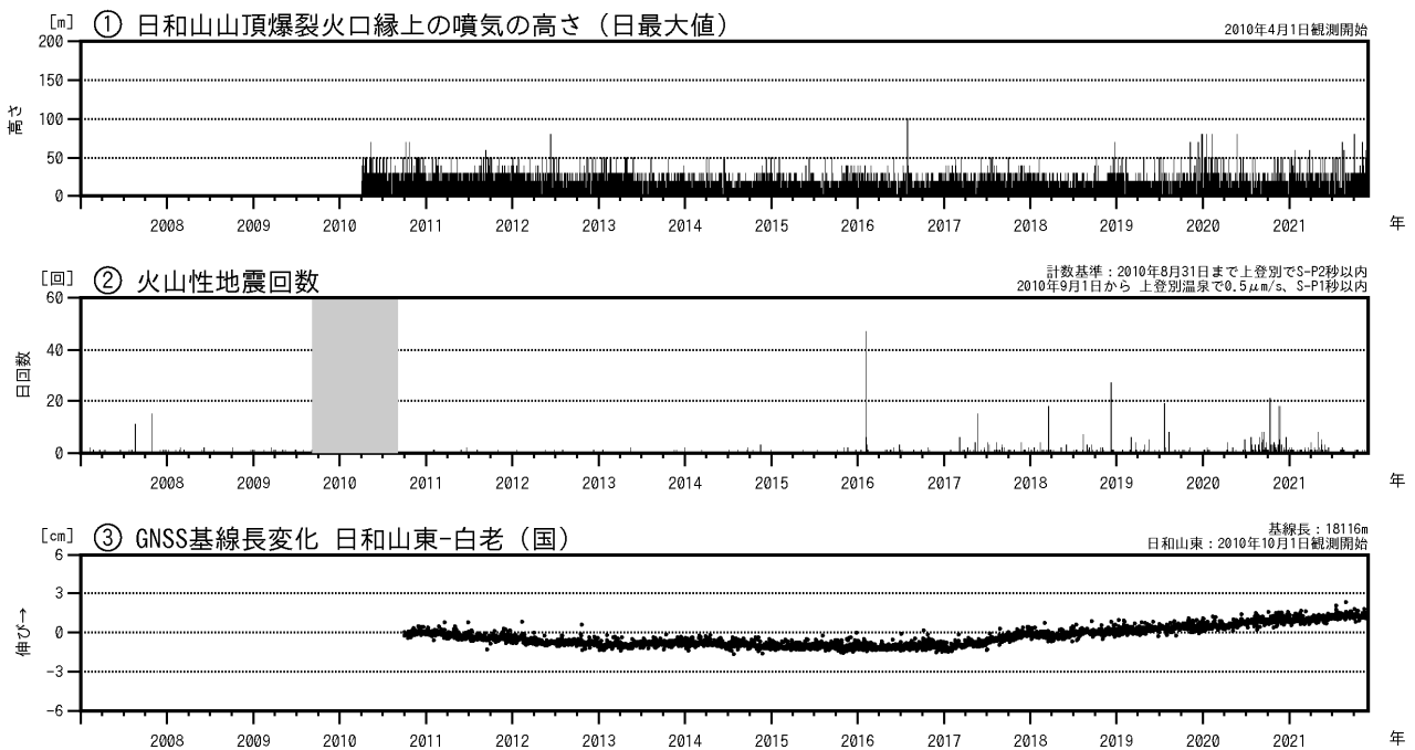
図2 倶多楽 火山活動経過図（2007年1月～2021年11月）
