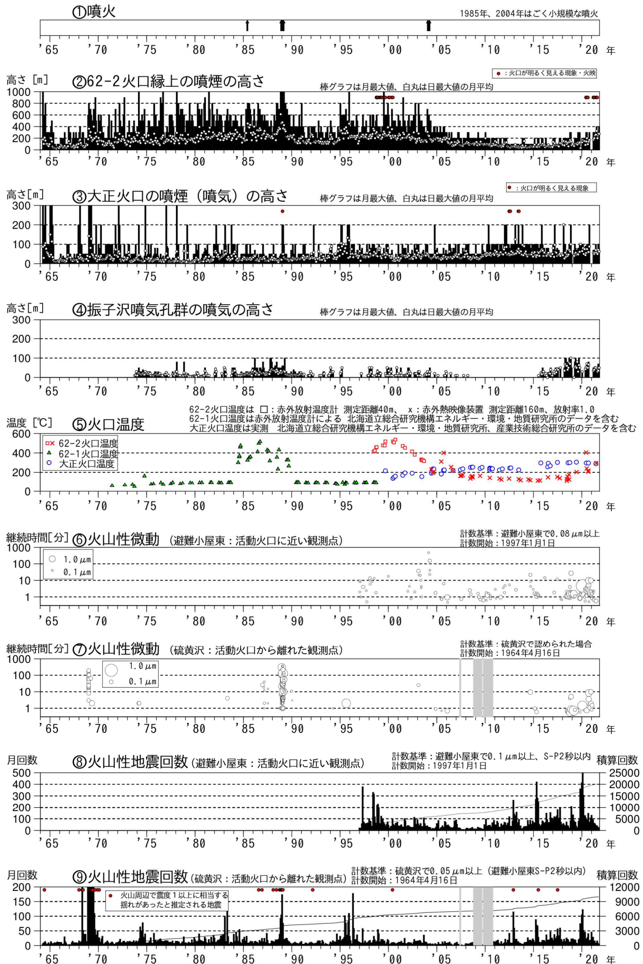
図1 十勝岳 火山活動経過図（1964年1月～2021年10月）
