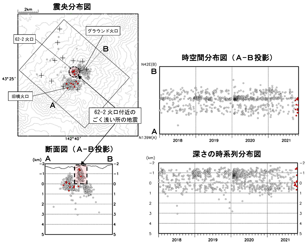
図4 十勝岳 火山性地震の震源分布（2018年1月～2021年10月） ●：2018年1月～2021年9月の震源 ●：2021年10月の震源 +：地震観測点
