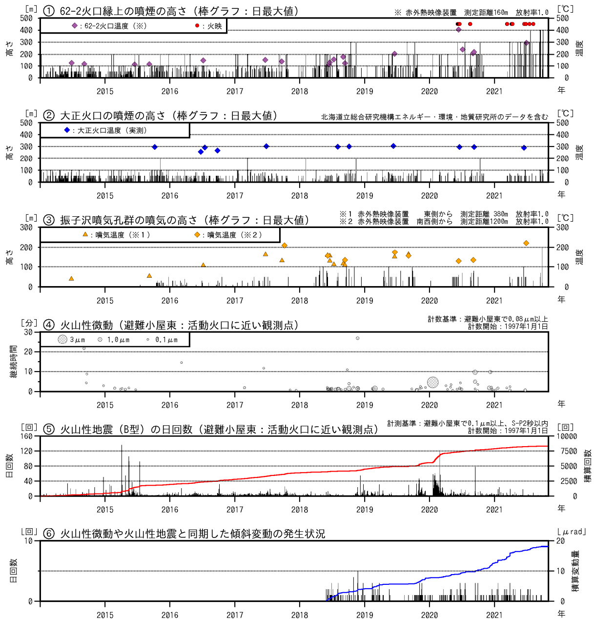
図2 十勝岳 火山活動経過図（2014年1月～2021年10月）
