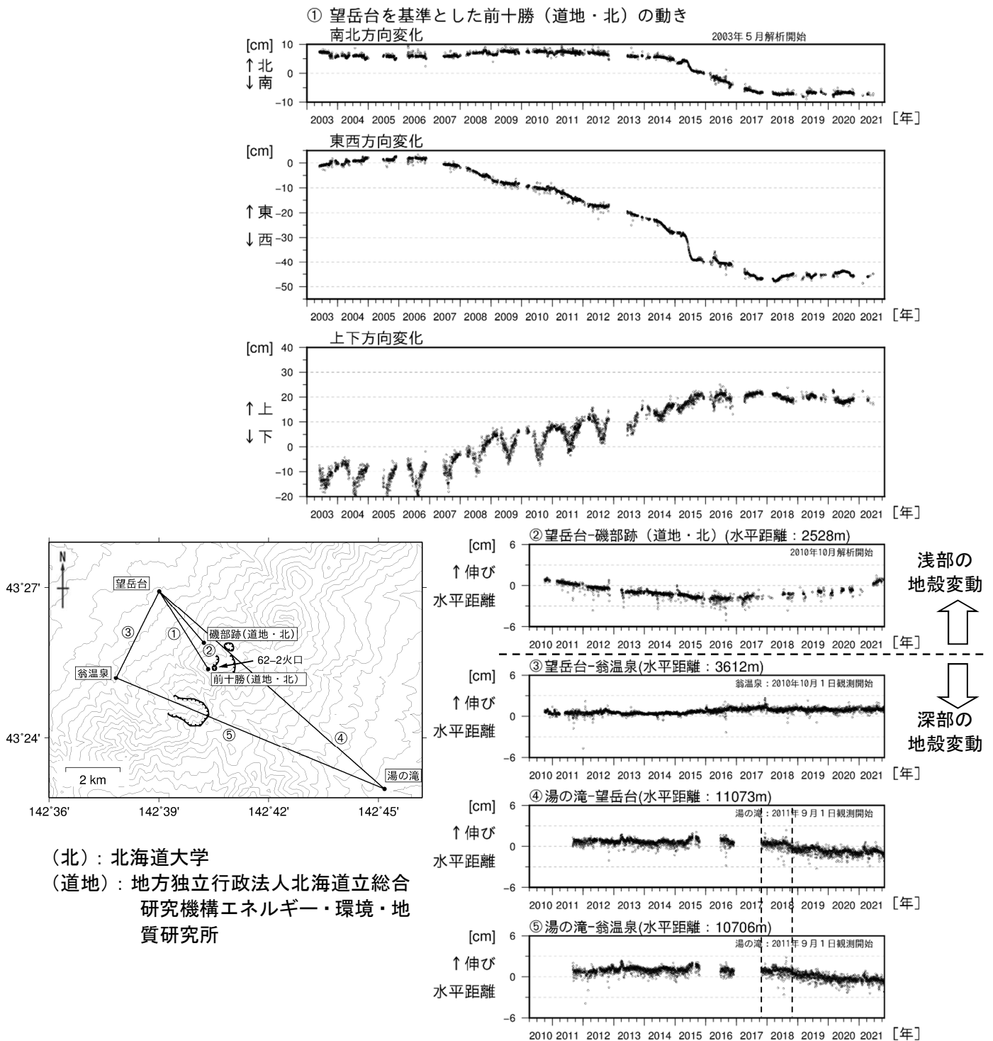
図6 十勝岳 GNSS連続観測による南北・東西・上下方向変化及び水平距離変化（2003年5月～2021年10月）及び観測点配置図
