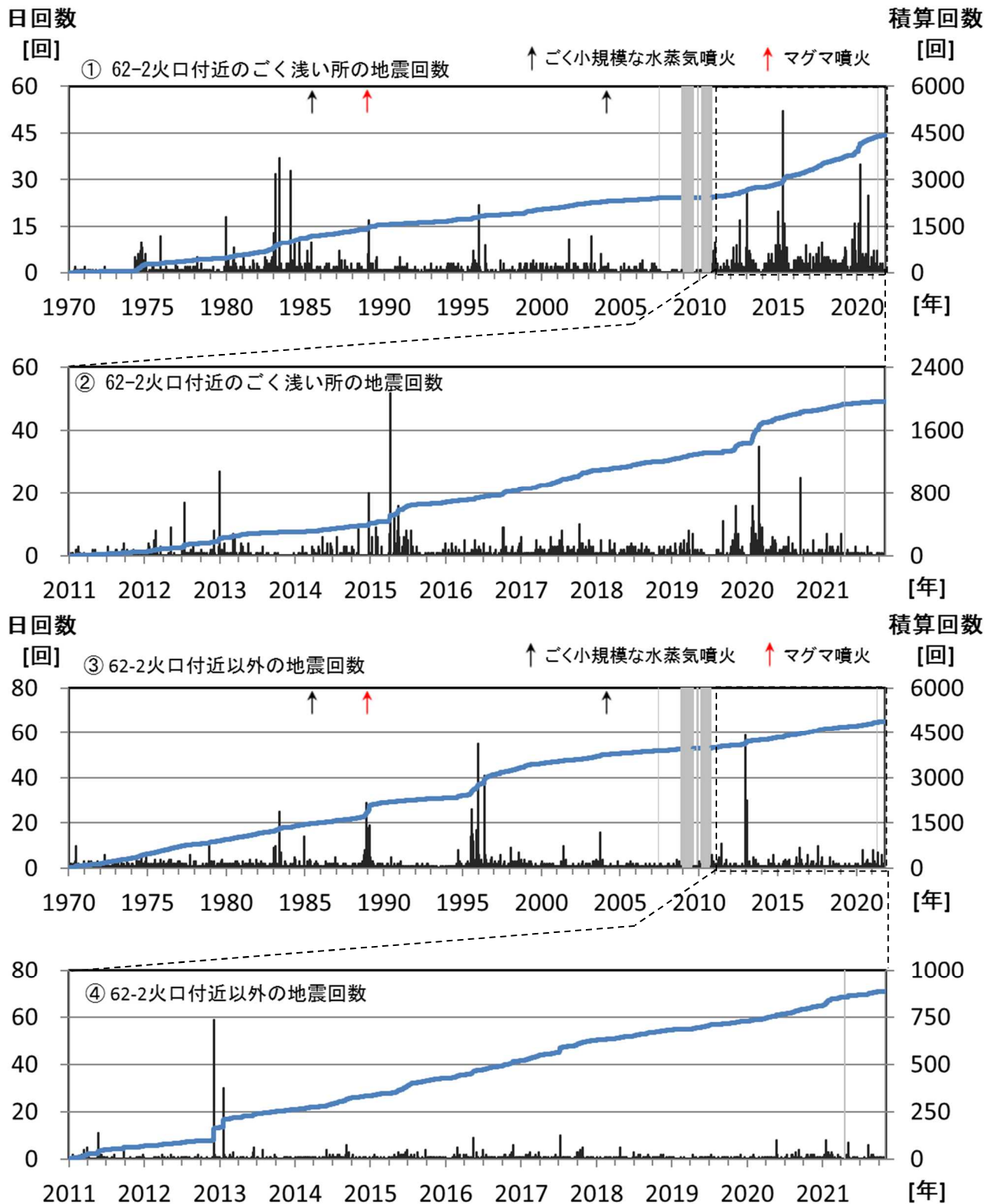
図5 十勝岳 地震の日回数及び積算回数（①③：1970年～2021年10月 ②④：2011年～2021年10月） 硫黄沢観測点（山麓点）で計測した回数（計数基準：0.05 \mu m以上）を示します。 ①、②は主に62-2火口付近のごく浅い所（図4中の破線に囲まれた領域内）で発生したと推測されるB型地震の回数を示します。また③、④の「62-2火口付近以外」は、主にグラウンド火口周辺や旧噴火口付近などで発生したと推測されるA型地震の回数を示します。 図中の、青線は積算回数を示し、灰色の部分は欠測を示します。
