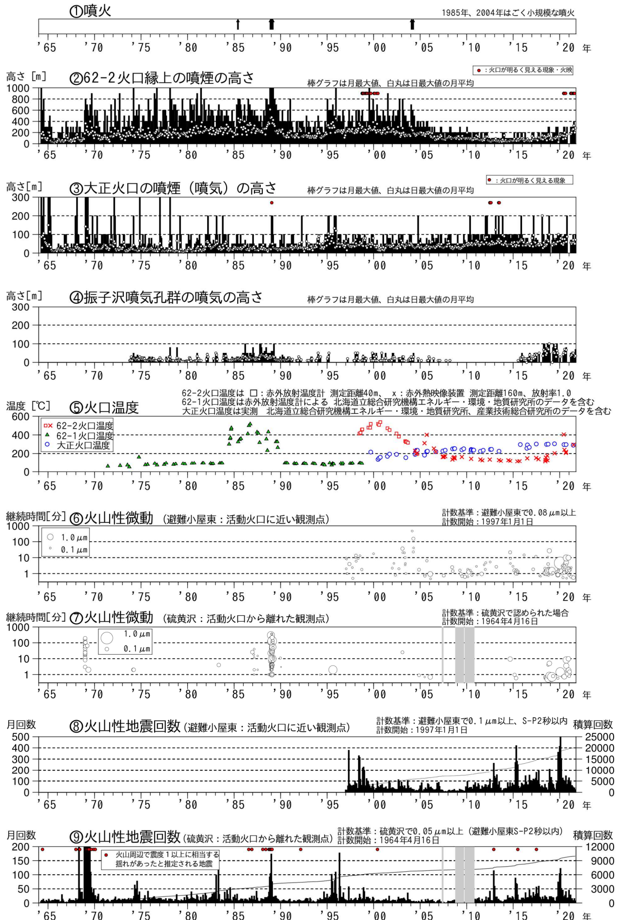
図1 十勝岳 火山活動経過図(1964年1月~2021年9月)
