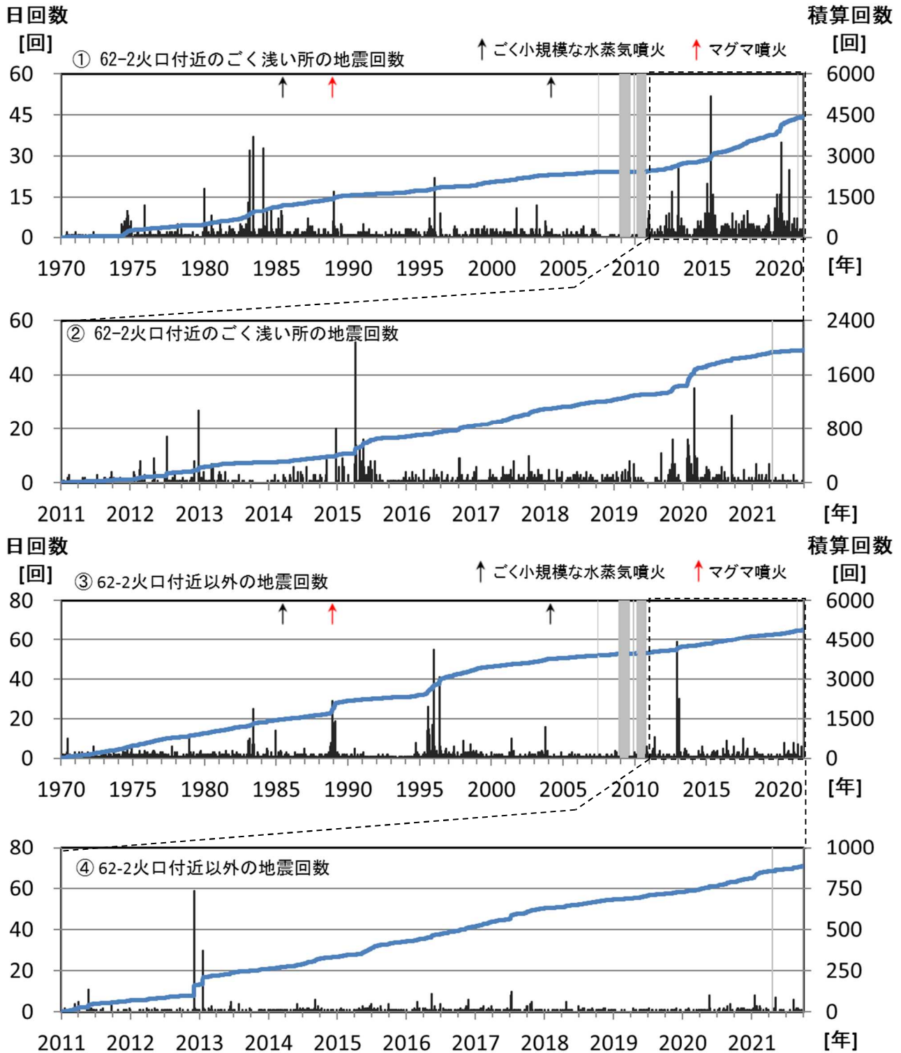
図7 十勝岳 地震の日回数及び積算回数（①③：1970年～2021年9月 ②④：2011年～2021年9月） 硫黄沢観測点（山麓点）で計測した回数（計数基準：0.05 \mu m以上）を示します。 ①、②は主に62-2火口付近のごく浅い所（図6中の破線に囲まれた領域内）で発生したと推測されるB型地震の回数を示します。また③、④の「62-2火口付近以外」は、主にグラウンド火口周辺や旧噴火口付近などで発生したと推測されるA型地震の回数を示します。 図中の、青線は積算回数を示し、灰色の部分は欠測を示します。
