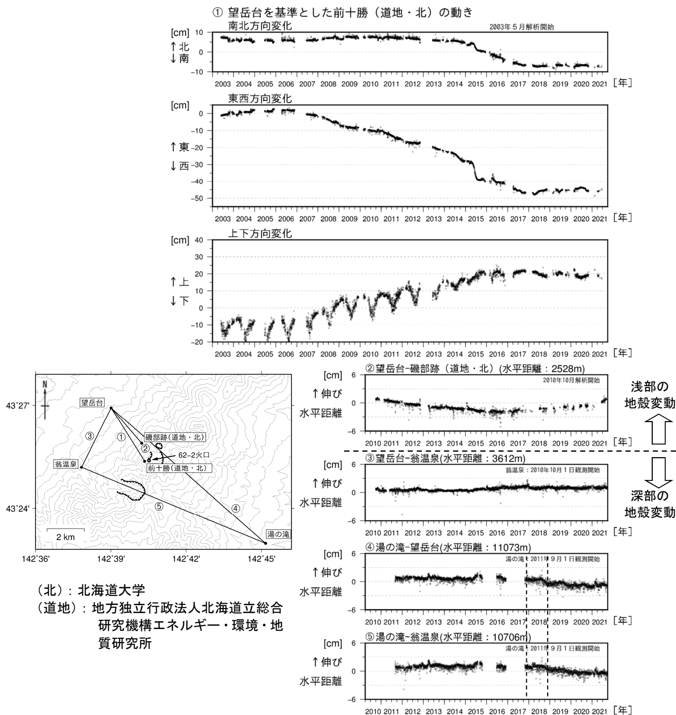
図8 十勝岳 GNSS連続観測による南北・東西・上下方向変化及び水平距離変化（2003年5月～2021年9月）及び観測点配置図
