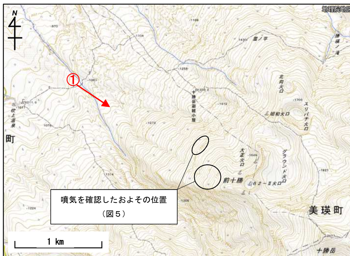
図4 十勝岳 火口周辺図と写真及び赤外熱映像の撮影方向（矢印）
