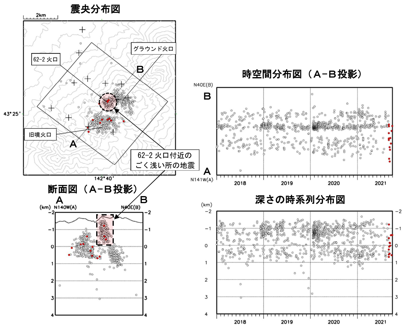
図6 十勝岳 火山性地震の震源分布（2018年1月～2021年9月） ●：2018年1月～2021年8月の震源 ●：2021年9月の震源 +：地震観測点
