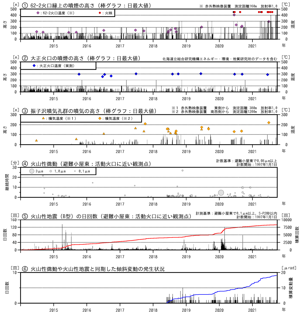
図2 十勝岳 火山活動経過図（2014年1月～2021年9月）
