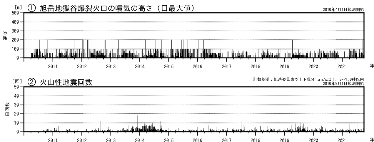
図1 大雪山 火山活動経過図（2010年4月～2021年9月）
