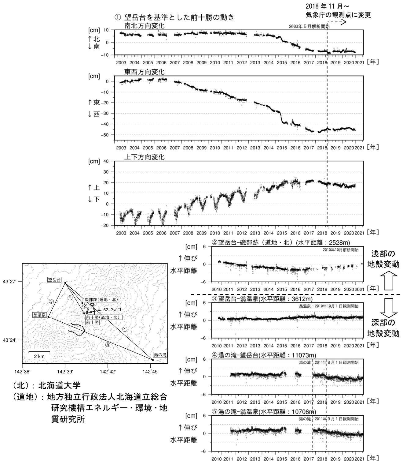
図7 十勝岳 GNSS連続観測による南北・東西・上下方向変化及び水平距離変化（2003年5月～2021年7月）及び観測点配置図
