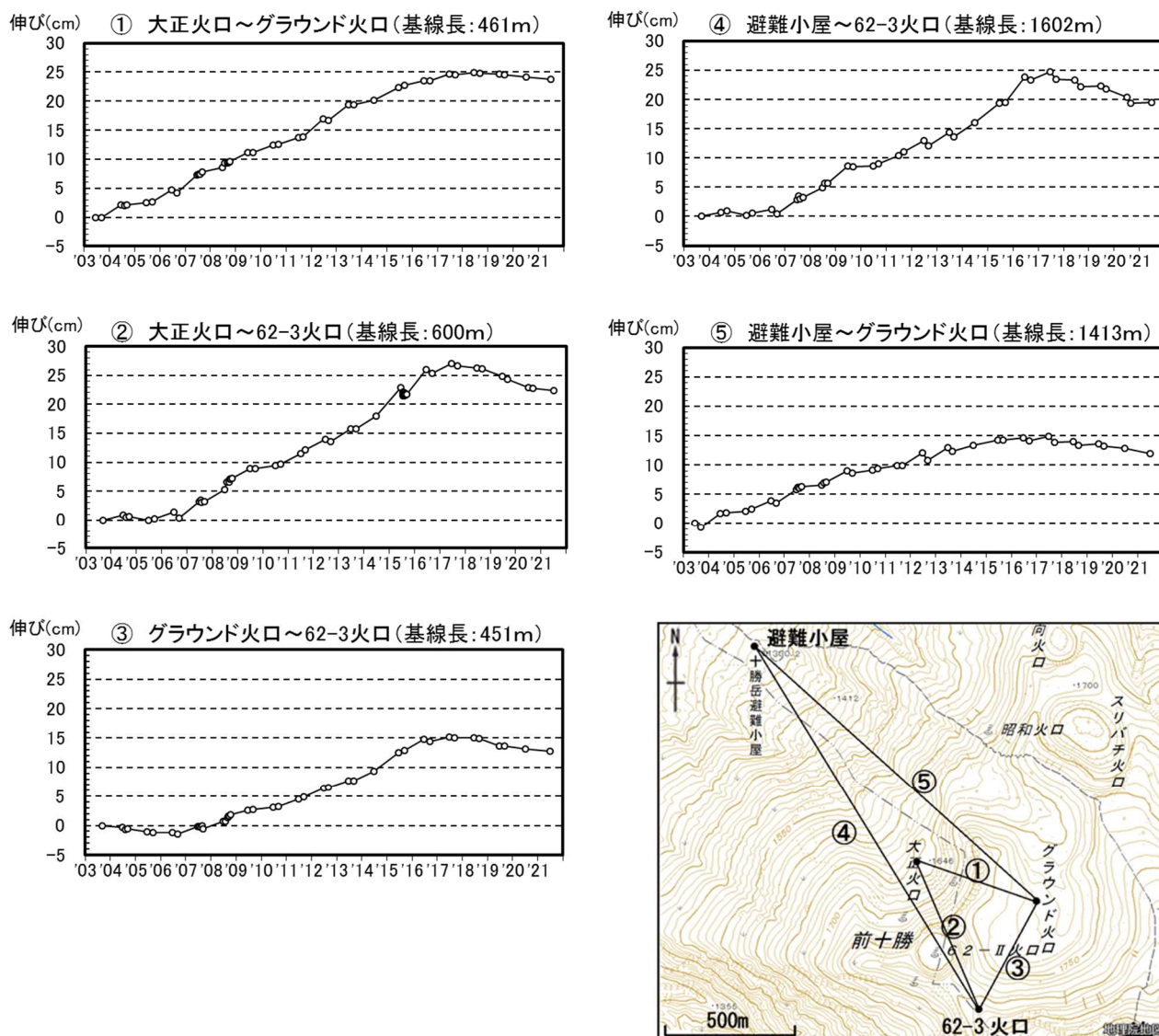
図8 十勝岳 GNSS繰り返し観測による基線長変化（2003年9月～2021年6月）及び観測点配置図 グラフ①～⑤は観測点配置図の基線①～⑤に対応しています。
