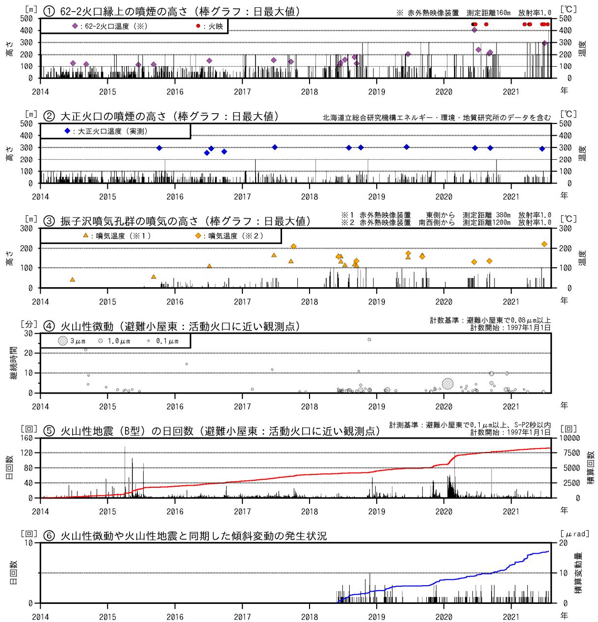
図2 十勝岳 火山活動経過図（2014年1月～2021年7月）
