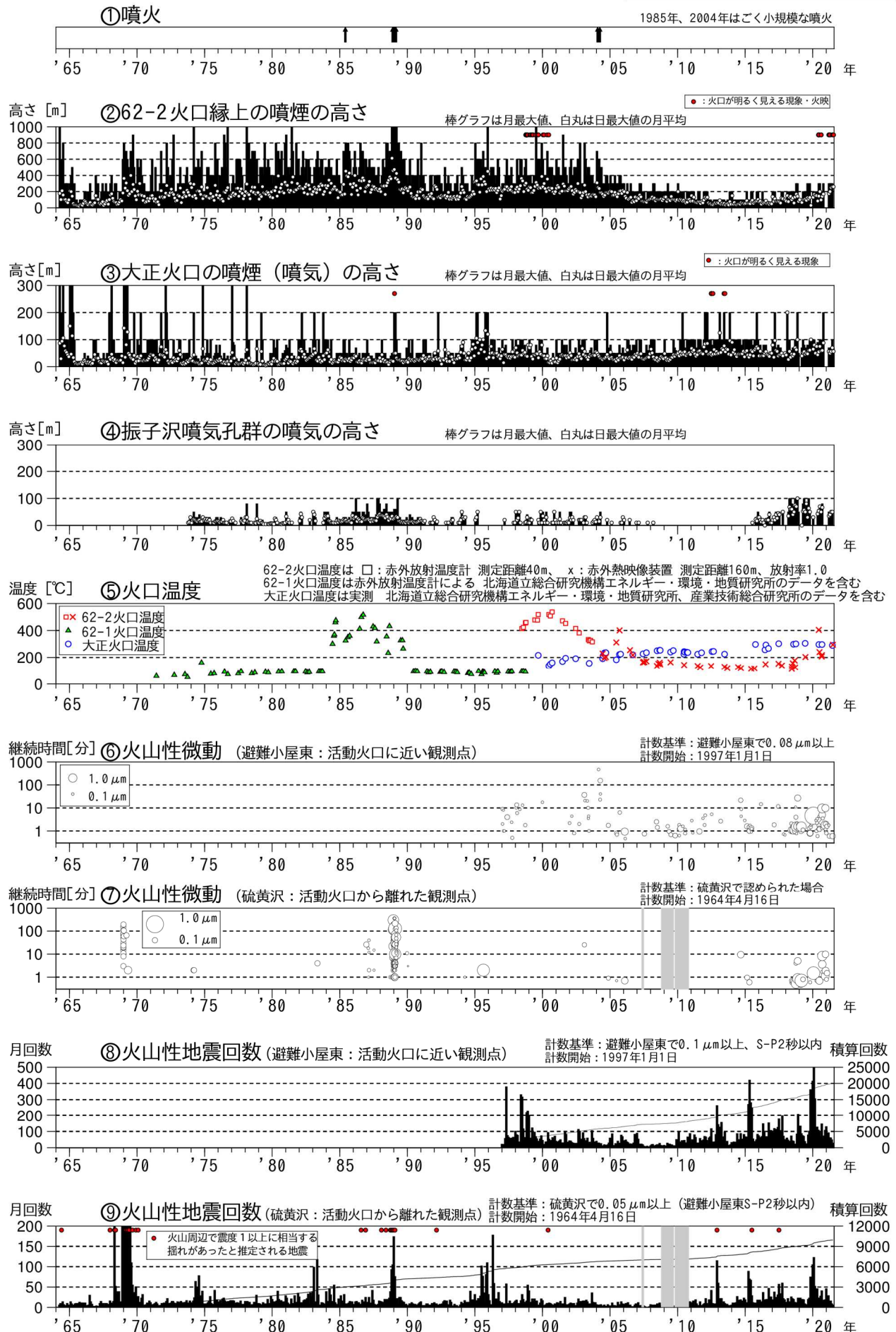
図1 十勝岳 火山活動経過図（1964年1月～2021年7月）
