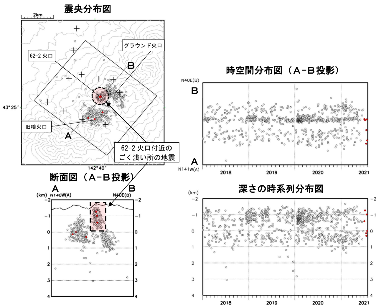
図5 十勝岳 火山性地震の震源分布（2018年1月～2021年7月） ●：2018年1月～2021年6月の震源 ●：2021年7月の震源 +：地震観測点
