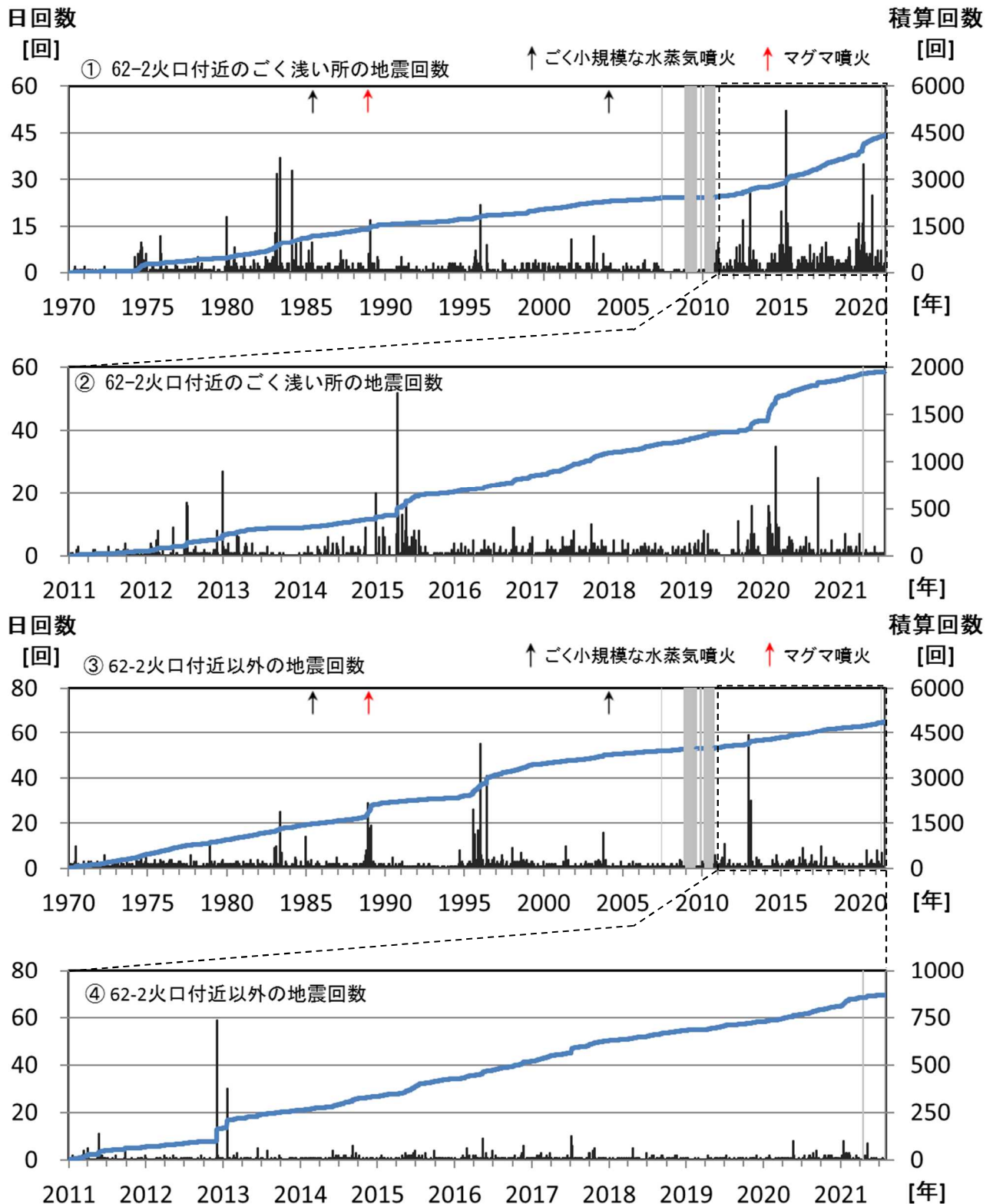
図6 十勝岳 地震の日回数及び積算回数（①③：1970年～2021年7月 ②④：2011年～2021年7月） 硫黄沢観測点（山麓点）で計測した回数（計数基準：0.05 \mu m以上）を示します。 ①、②は主に62-2火口付近のごく浅い所（図5中の破線に囲まれた領域内）で発生したと推測されるB型地震の回数を示します。また③、④の「62-2火口付近以外」は、主にグラウンド火口周辺や旧噴火口付近などで発生したと推測されるA型地震の回数を示します。 図中の、青線は積算回数を示し、灰色の部分は欠測を示します。
