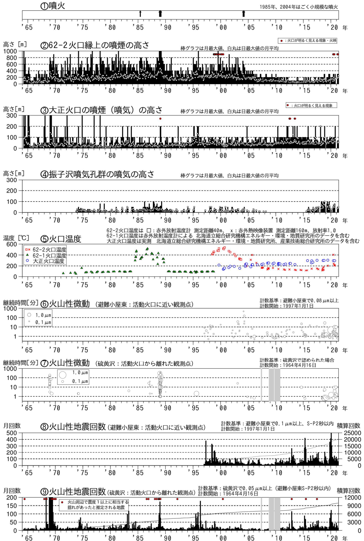
図1 十勝岳 火山活動経過図 (1964年1月~2021年5月)
