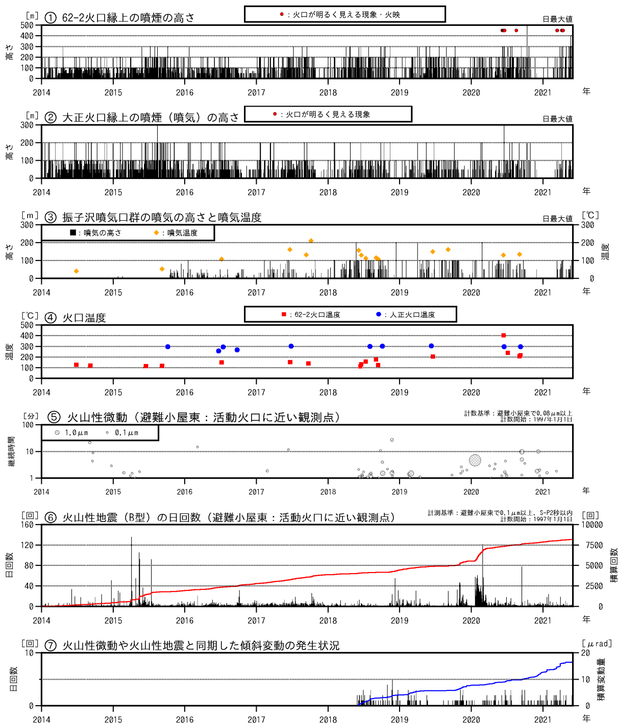
図2 十勝岳 火山活動経過図（2014年1月～2021年5月）
