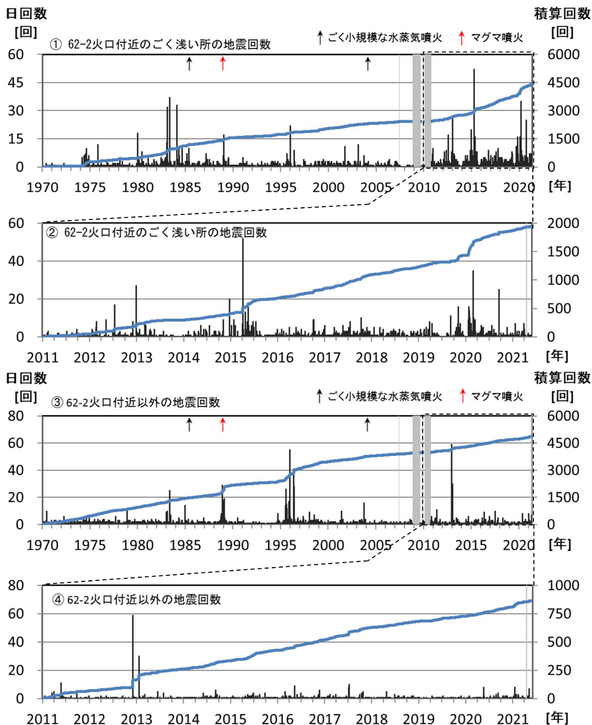
図5 十勝岳 地震の日回数及び積算回数（①③：1970年～2021年5月 ②④：2011年～2021年5月） 硫黄沢観測点（山麓点）で計測した回数（計数基準：0.05 \mu m以上）を示します。 ①、②は主に62-2火口付近のごく浅い所（図4中の破線に囲まれた領域内）で発生したと推測されるB型地震の回数を示します。また③、④の「62-2火口付近以外」は、主にグラウンド火口周辺や旧噴火口付近などで発生したと推測されるA型地震の回数を示します。 図中の、青線は積算回数を示し、灰色の部分は欠測を示します。
