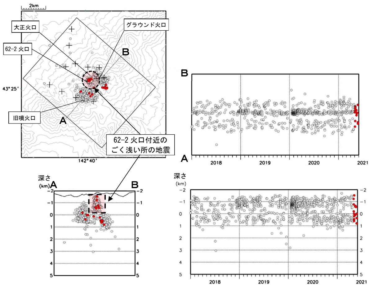
図4 十勝岳 火山性地震の震源分布 (2018年1月～2021年5月) ●: 2018年1月～2021年4月の震源 ●: 2021年5月の震源 +: 地震観測点
