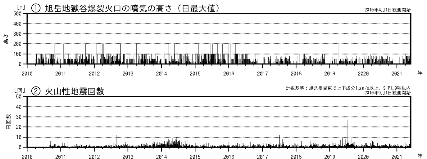
図1 大雪山 火山活動経過図（2010年4月～2021年5月）
