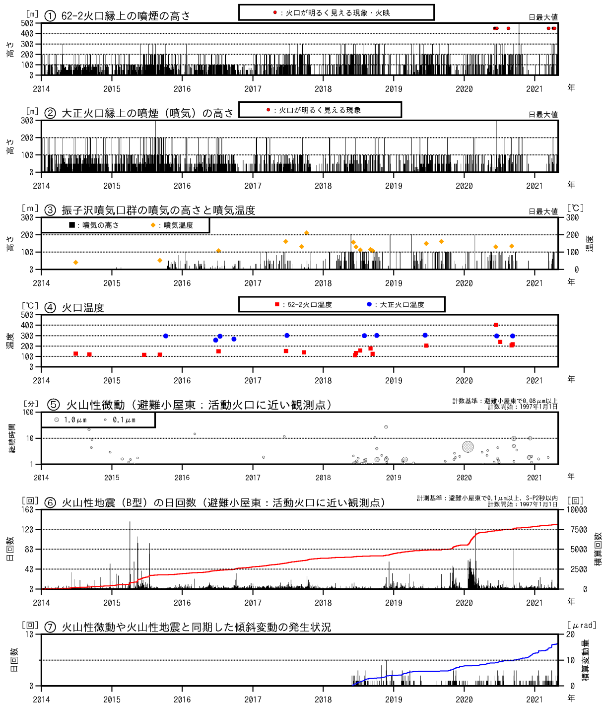
図2 十勝岳 火山活動経過図（2014年1月～2021年4月）
