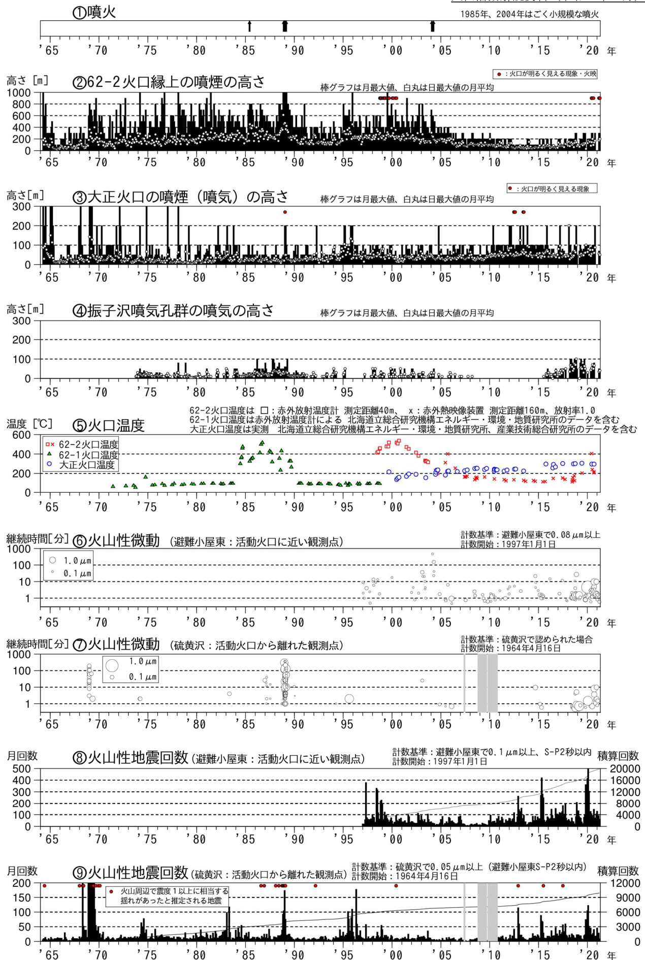
図1 十勝岳 火山活動経過図（1964年1月～2021年4月）
