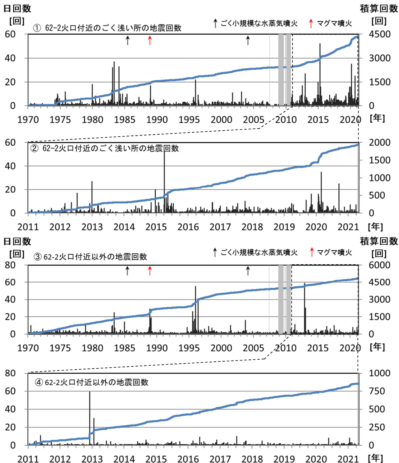
図6 十勝岳 地震の日回数及び積算回数（①③：1970年～2021年4月 ②④：2011年～2021年4月） 硫黄沢観測点（山麓点）で計測した回数（計数基準：0.05 \mu m以上）を示します。 ①、②は主に62-2火口付近のごく浅い所（図5中の破線に囲まれた領域内）で発生したと推測されるB型地震の回数を示します。また③、④の「62-2火口付近以外」は、主にグラウンド火口周辺や旧噴火口付近などで発生したと推測されるA型地震の回数を示します。 図中の、青線は積算回数を示し、灰色の部分は欠測を示します。
