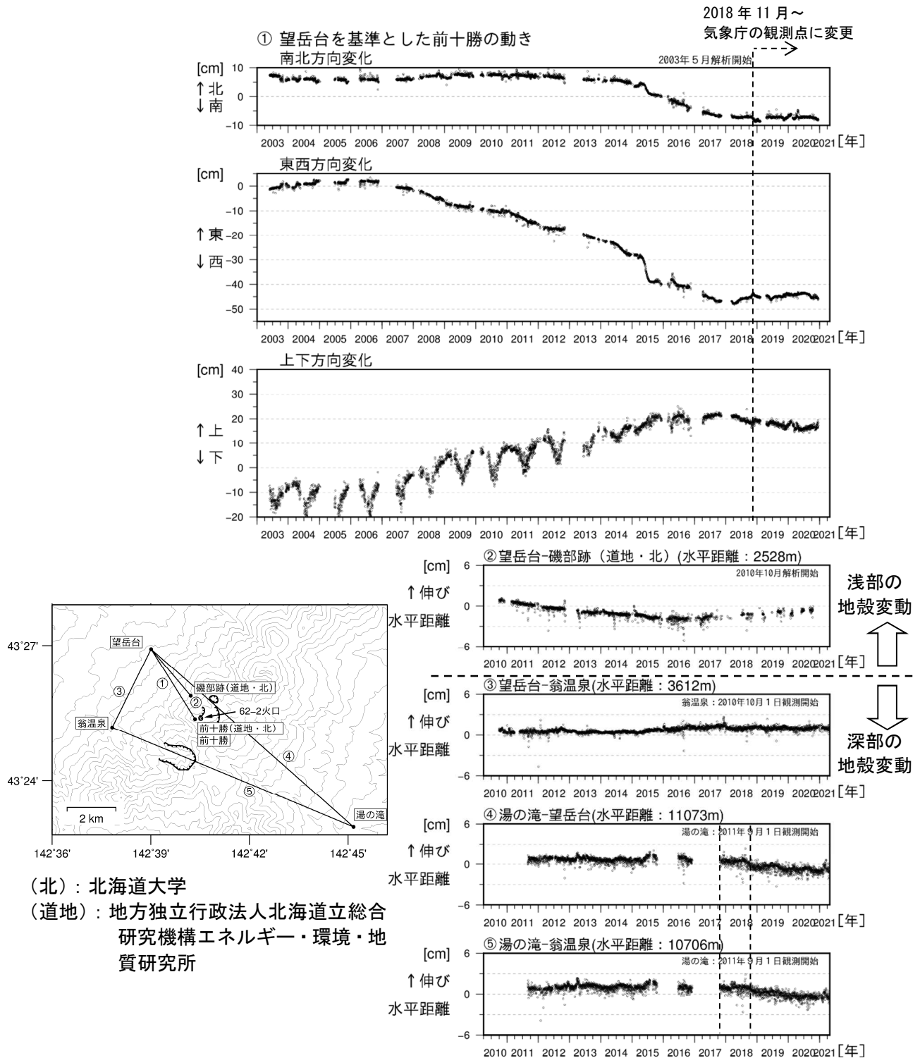
図7 十勝岳 GNSS連続観測による南北・東西・上下方向変化及び水平距離変化と観測点配置図 (2003年5月～2021年4月)
