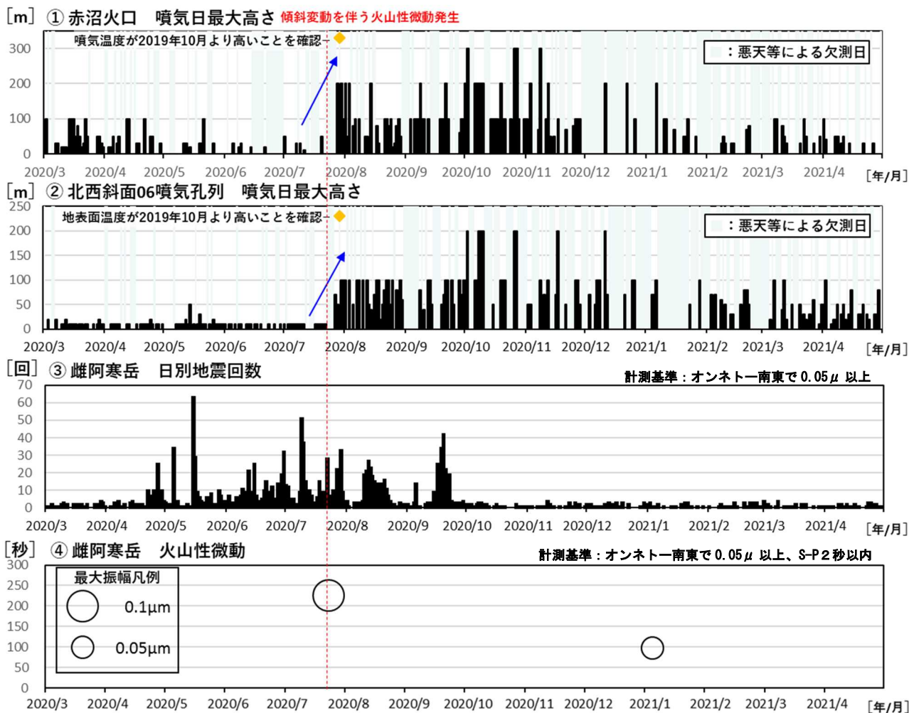
図5 雌阿寒岳 2020年7月以降の噴気活動及び地震活動等の活動経過（2020年3月～2021年4月）
