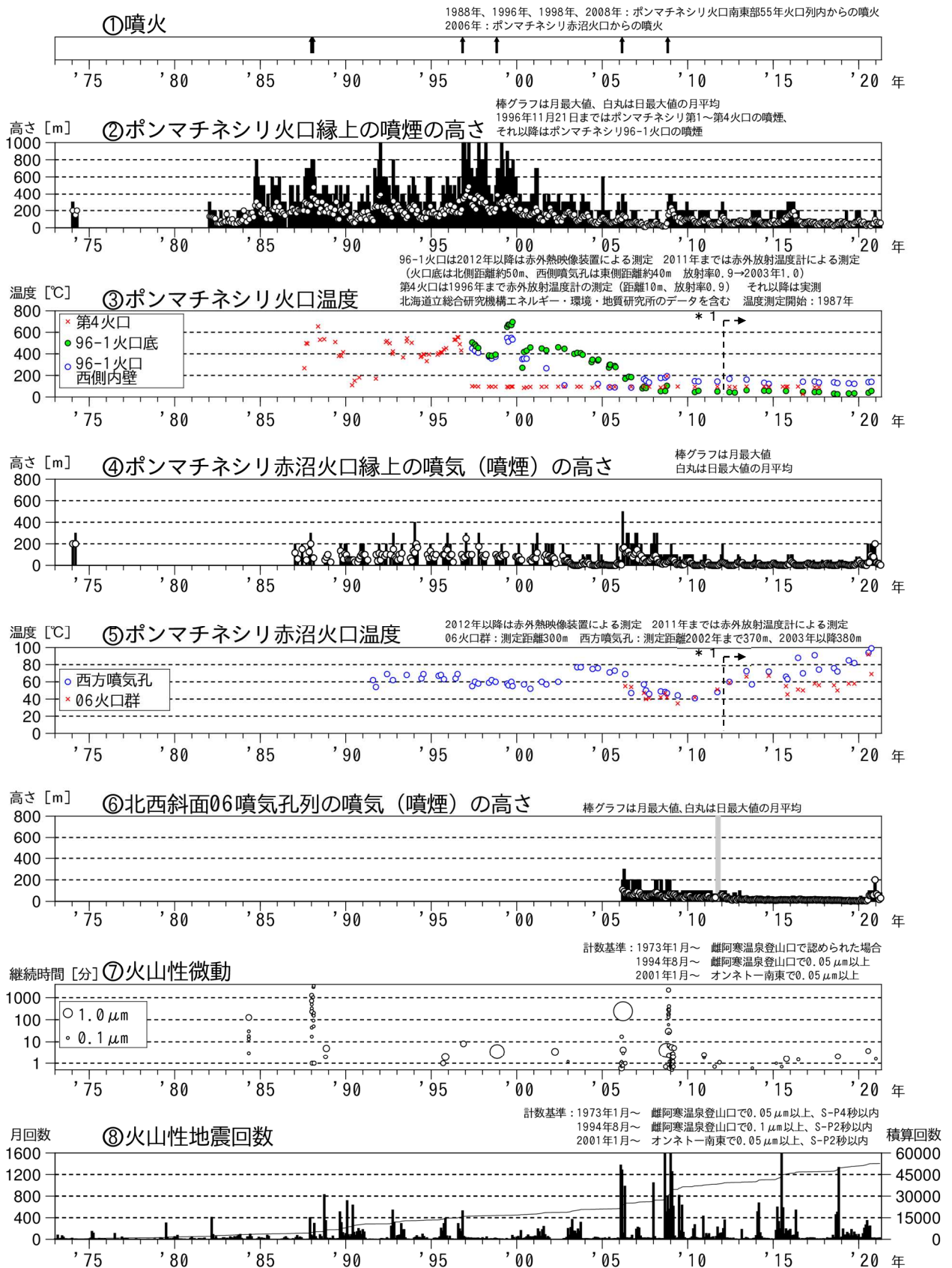
図1 雌阿寒岳 火山活動経過図 (1973年1月～2021年4月)
