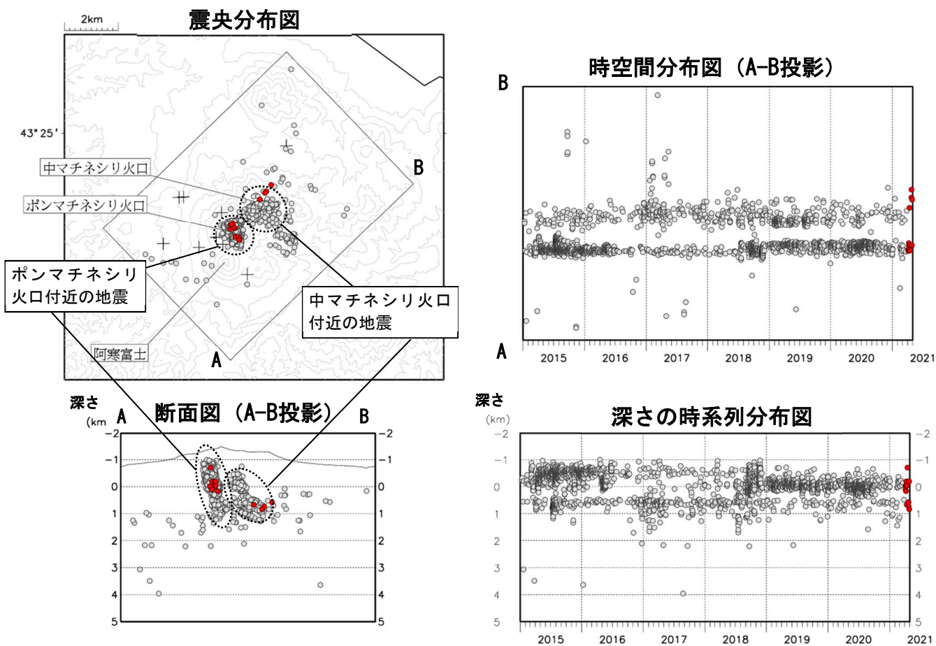
図8 雌阿寒岳 火山性地震の震源分布（2015年1月～2021年4月） ●印：2015年1月～2021年3月の震源、●印：2021年4月の震源、+印：地震観測点
