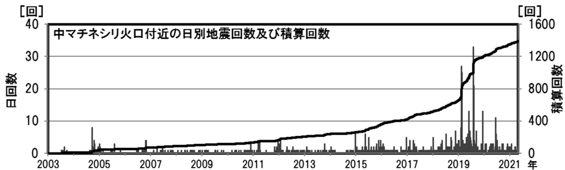
図7 雌阿寒岳 中マチネシリ火口付近の日別地震回数（2003年～2021年4月） ・中マチネシリ火口付近で発生する地震の回数は少なく経過しました。地震回数は増減を繰り返しながら2014年以前よりもやや多い状態となっています。
