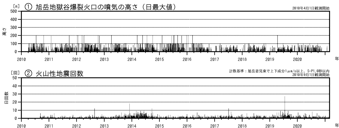
図1 大雪山 火山活動経過図（2010年4月～2021年2月）
