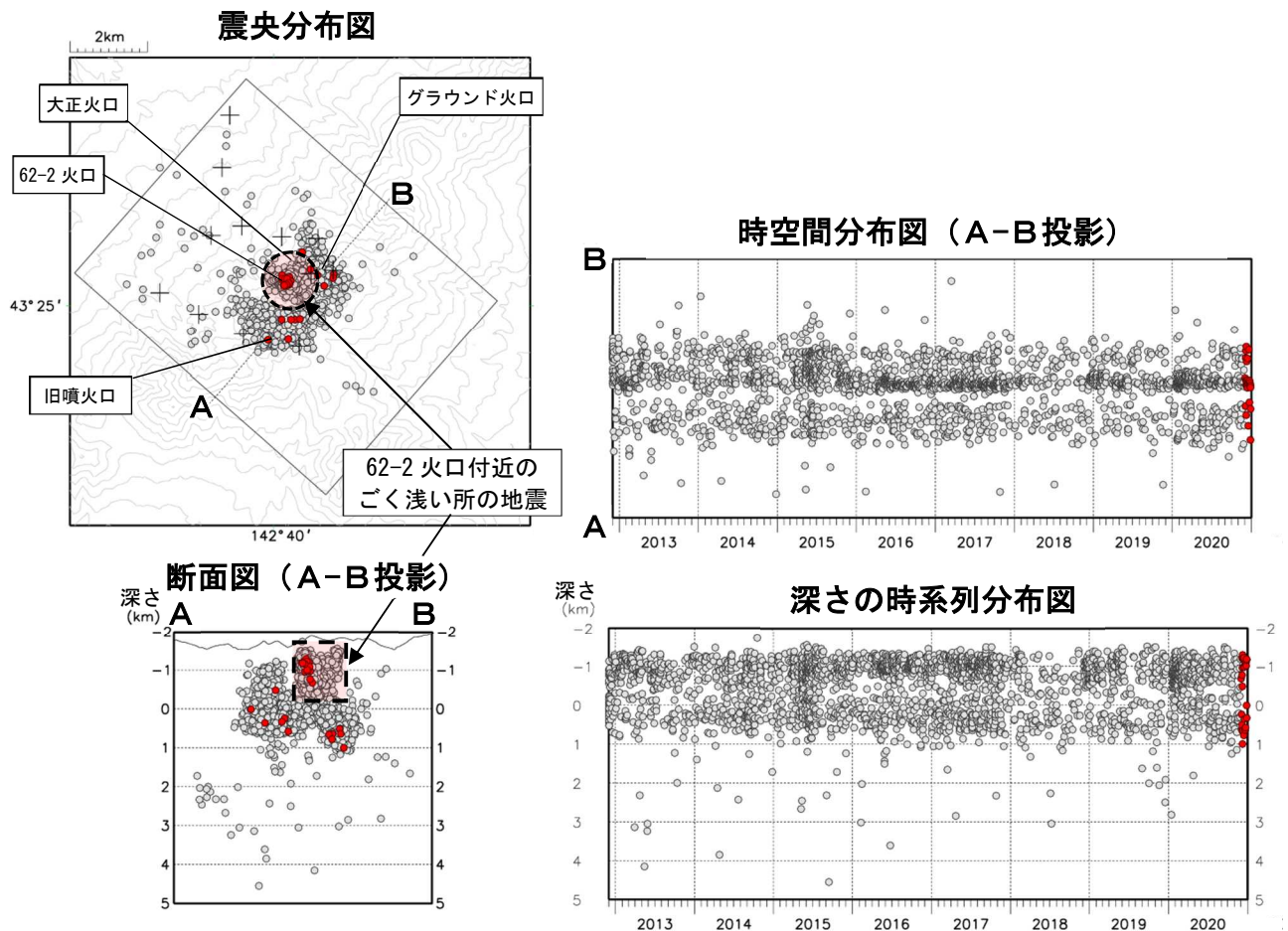
図4 十勝岳 火山性地震の震源分布（2012年12月～2020年12月） ●：2012年12月～2020年11月の震源 ●：2020年12月の震源 +：地震観測点
