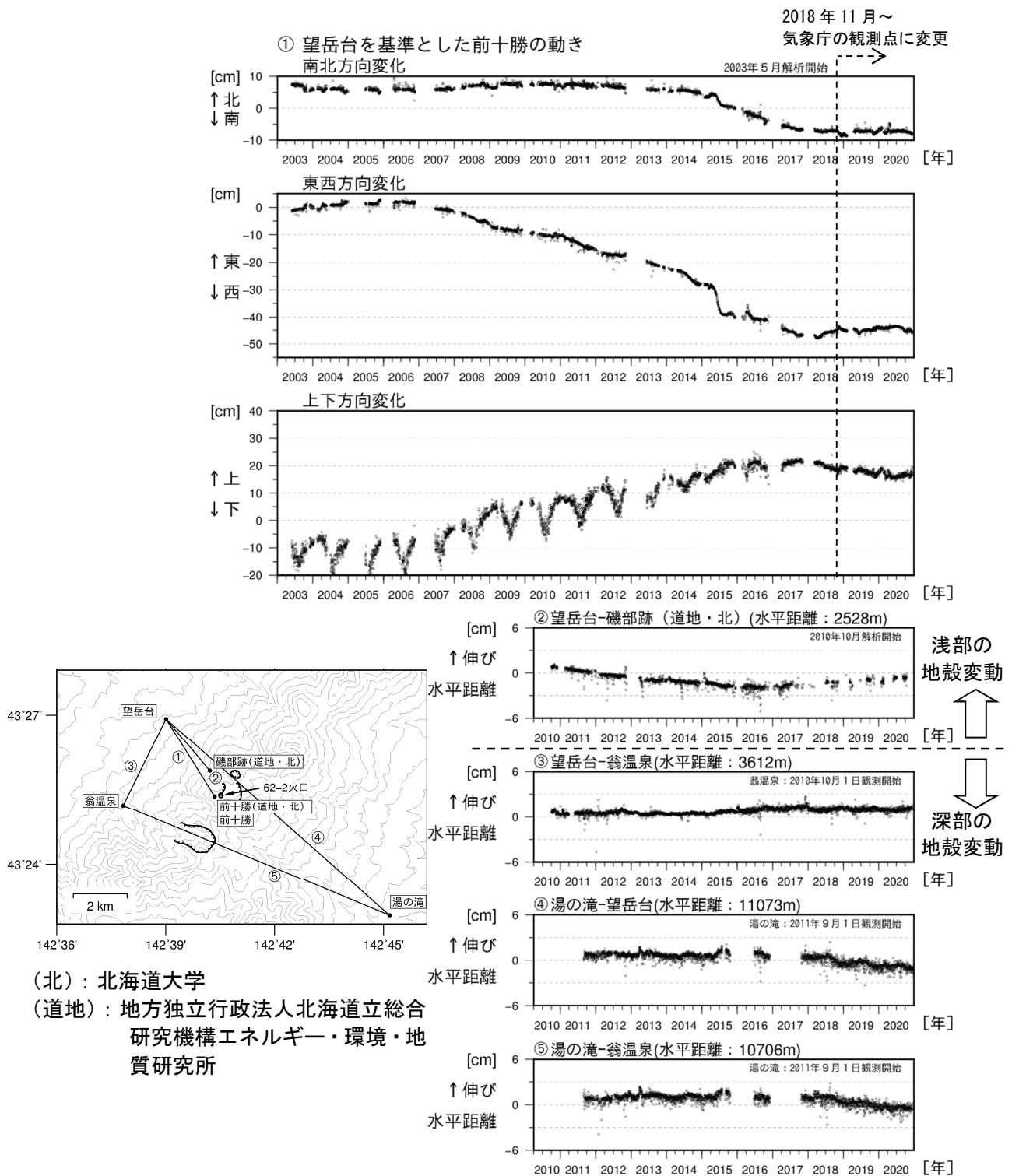
図6 十勝岳 GNSS連続観測による南北・東西・上下方向変化及び水平距離変化（2003年5月～2020年12月）、観測点配置図
