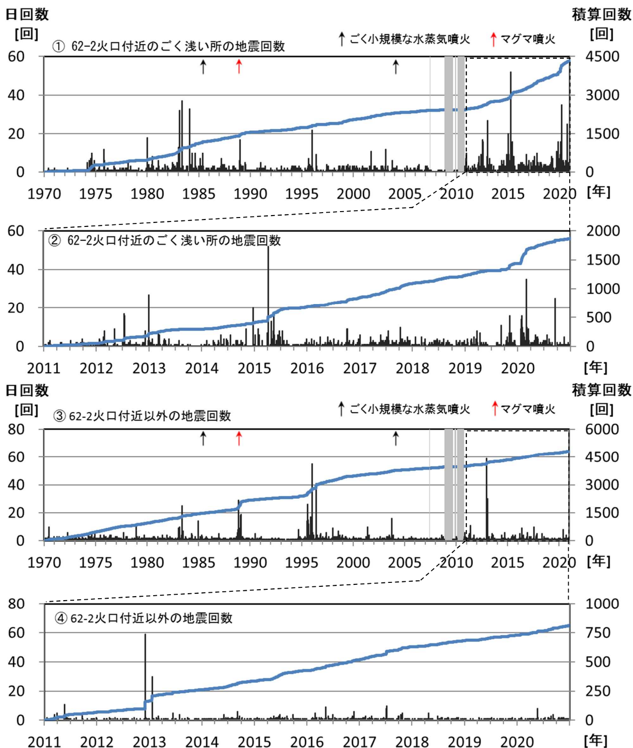
図5 十勝岳 地震の日回数及び積算回数（①③：1970年～2020年12月 ②④：2011年～2020年12月）
