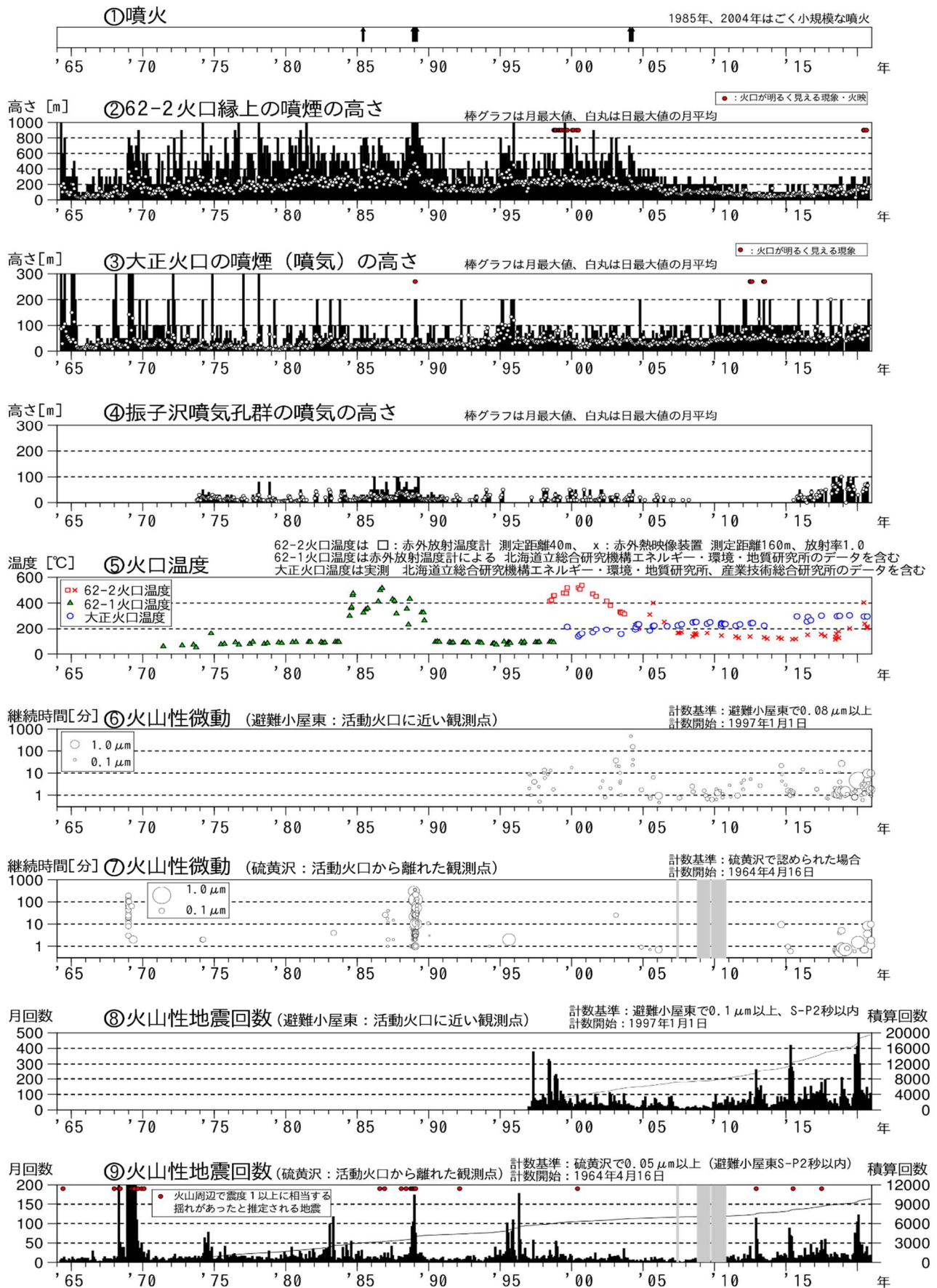
図1 十勝岳 火山活動経過図（1964年1月～2020年12月）
