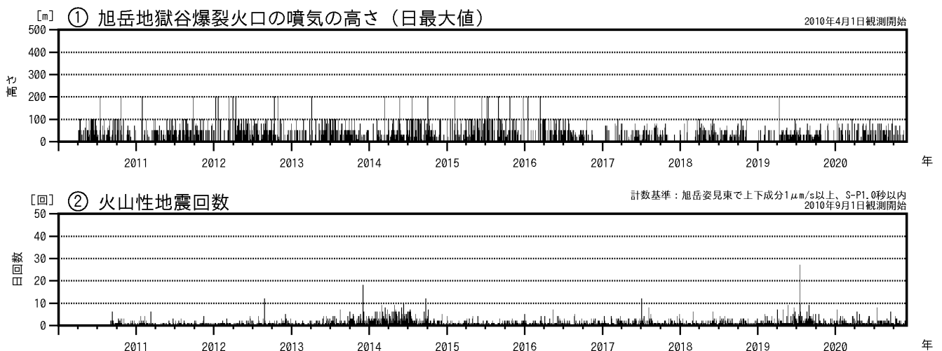
図1 大雪山 火山活動経過図（2010年4月～2020年11月）
