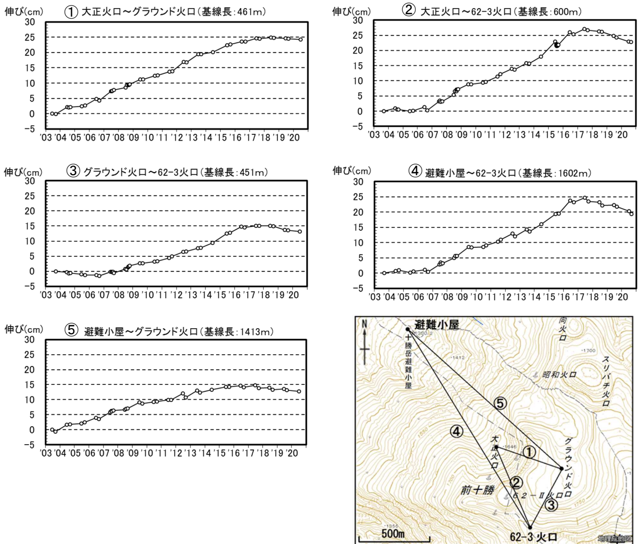
図7 十勝岳 GNSS繰り返し観測による基線長変化（2003年9月～2020年9月）及び観測点配置図 GNSS基線①～⑤は観測点配置図の①～⑤に対応しています。 2020年9月のグラウンド火口の観測データは欠測しています。
