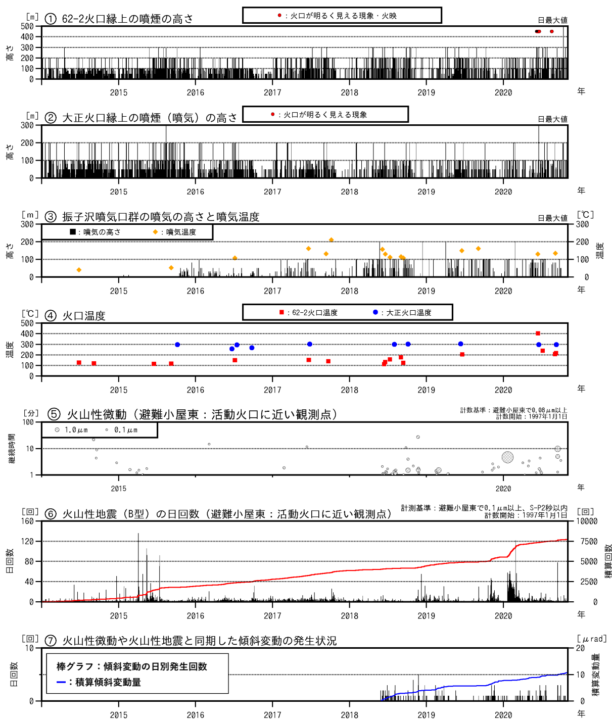
図2 十勝岳 火山活動経過図（2014年1月～2020年10月）
