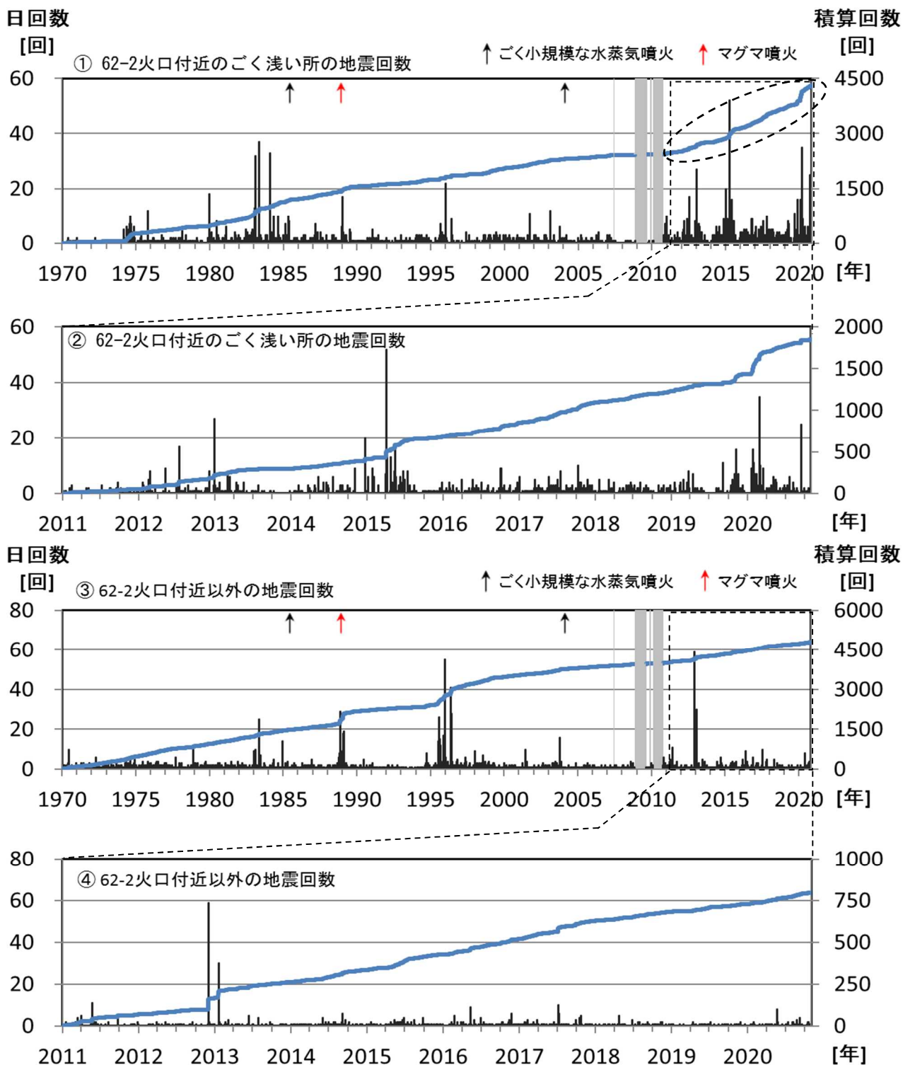
図5 十勝岳 地震の日回数及び積算回数（①③：1970年～2020年10月 ②④：2011年～2020年10月） 硫黄沢観測点（山麓点）で計測した回数（計数基準：0.05 \mu m以上）を示します。 ①、②は主に62-2火口付近のごく浅い所（図4中の破線に囲まれた領域内）で発生したと推測されるB型地震の回数を示します。また③、④の「62-2火口付近以外」とは、主にグラウンド火口周辺や旧噴火口付近などで発生したと推測されるA型地震の回数を示します。 図中の、青線は積算回数を示し、灰色の部分に欠測を示します。
