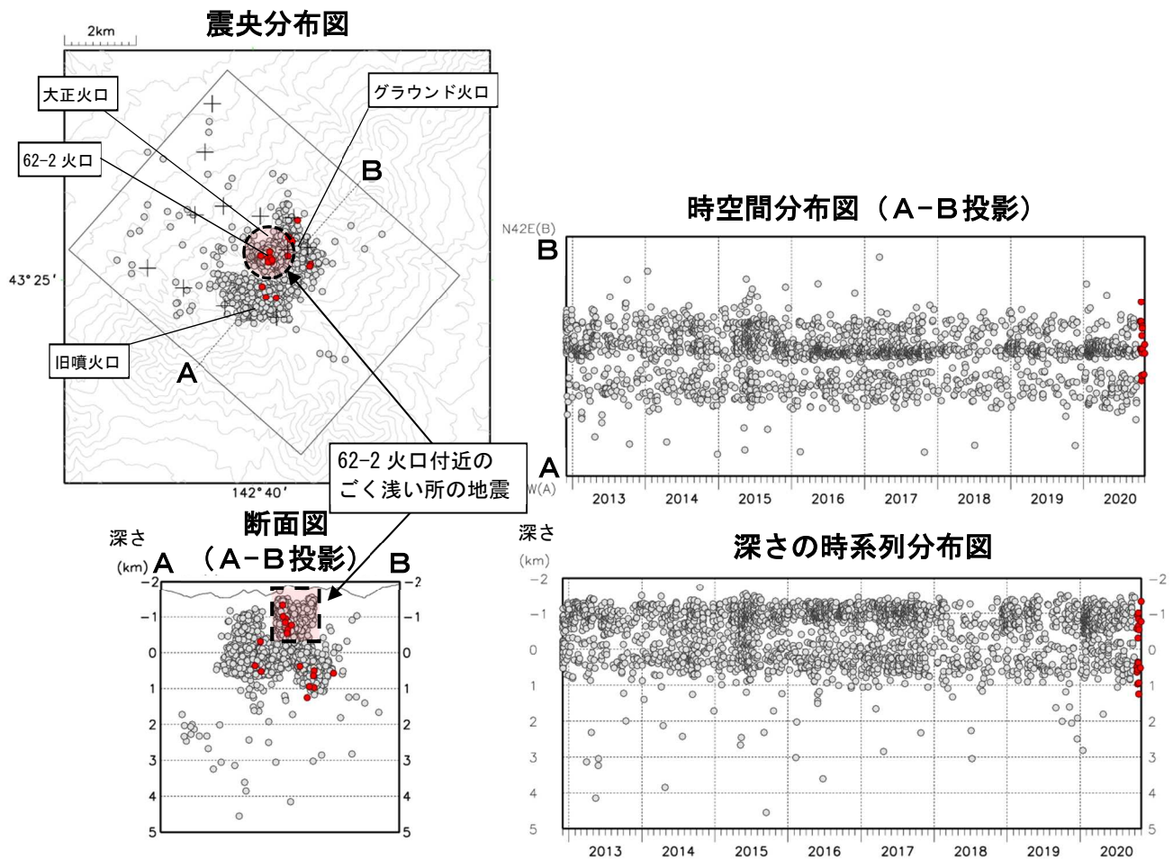
図4 十勝岳 火山性地震の震源分布 (2012年12月～2020年10月)
