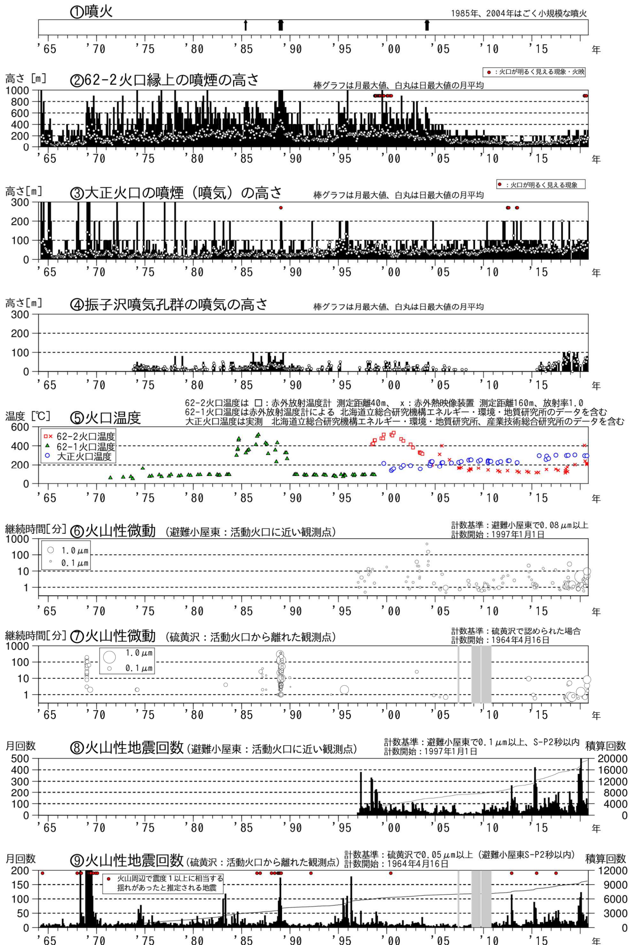
図1 十勝岳 火山活動経過図（1964年1月～2020年10月）
