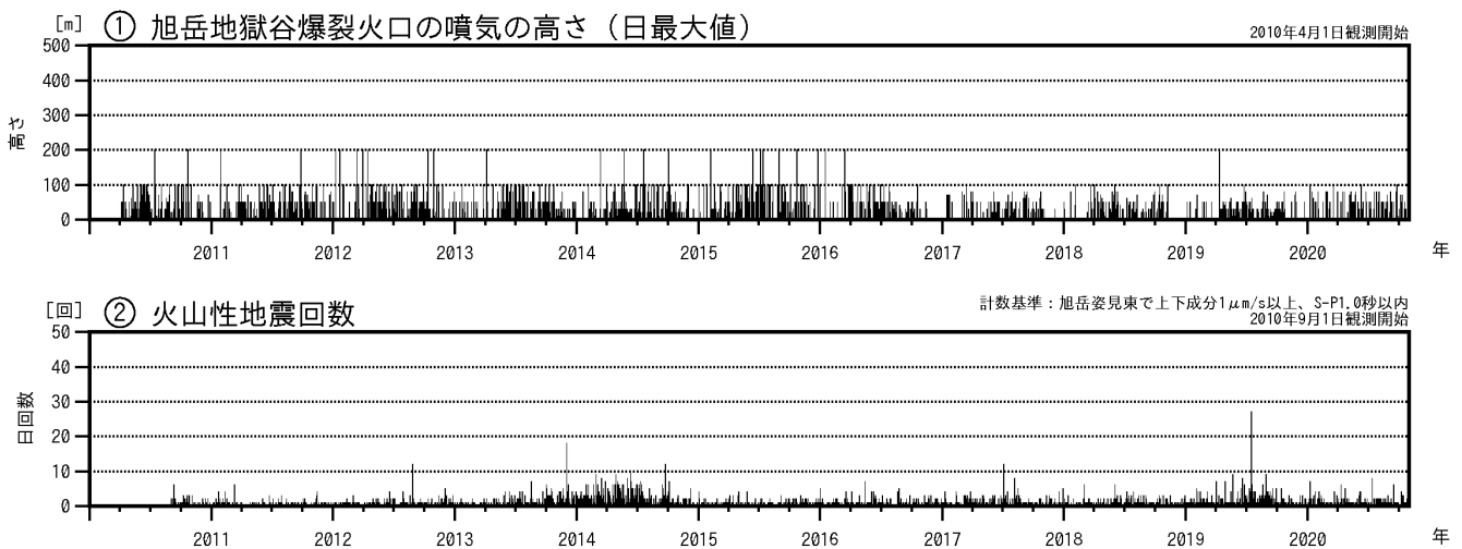
図1 大雪山 火山活動経過図（2010年4月～2020年10月）
