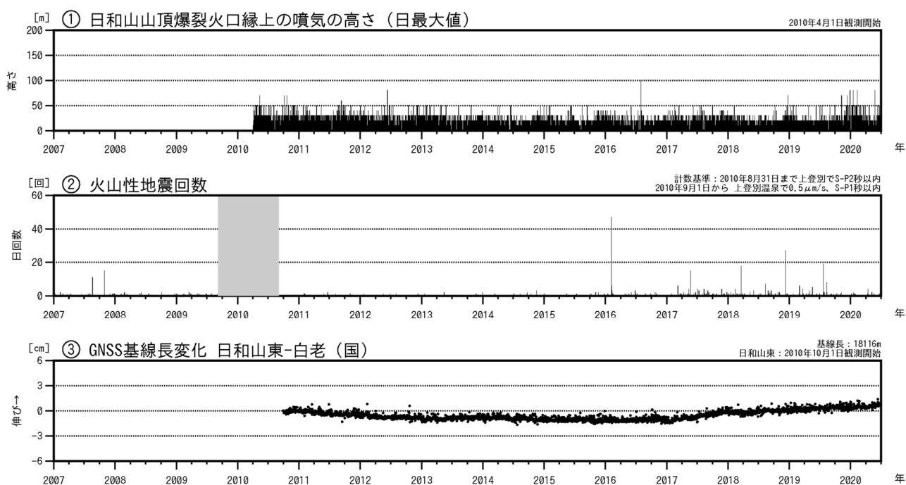
図2 倶多楽 火山活動経過図（2007年1月～2020年6月） ②の灰色の期間は機器障害による欠測を示します。 ③のGNSS基線は右配置図の基線に対応しています。 ③のGNSS基線は「平成23年（2011年）東北地方太平洋沖地震」及び「平成30年北海道胆振東部地震」に伴うステップを補正しています。 ・倶多楽周辺で、2017年頃から観測されている基線長の変化が継続しています。
