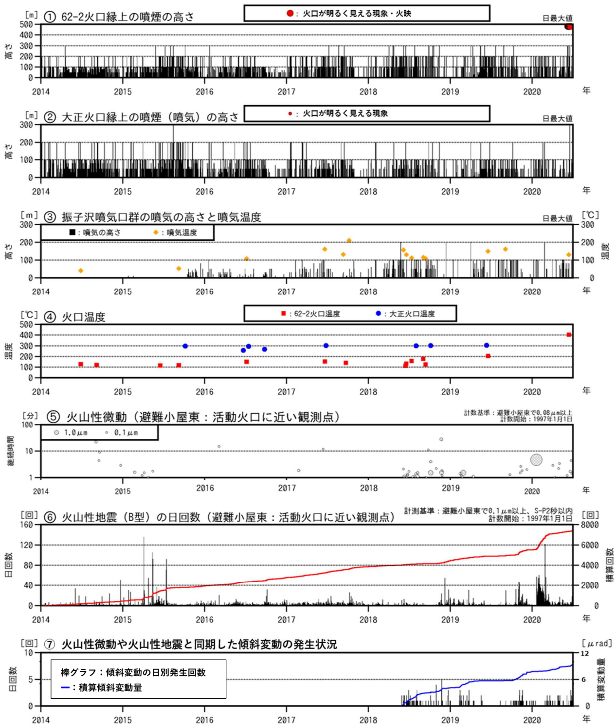
図2 十勝岳 火山活動経過図（2014年1月～2020年6月）
