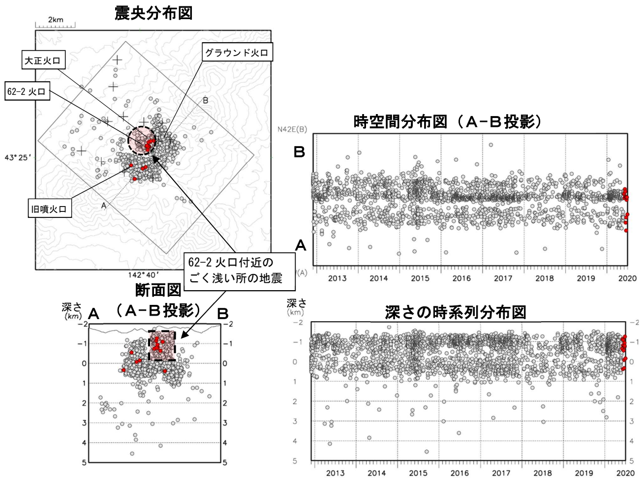
図8 十勝岳 火山性地震の震源分布（2012年12月～2020年6月） ●：2012年12月～2020年5月の震源 ●：2020年6月の震源 +：地震観測点
