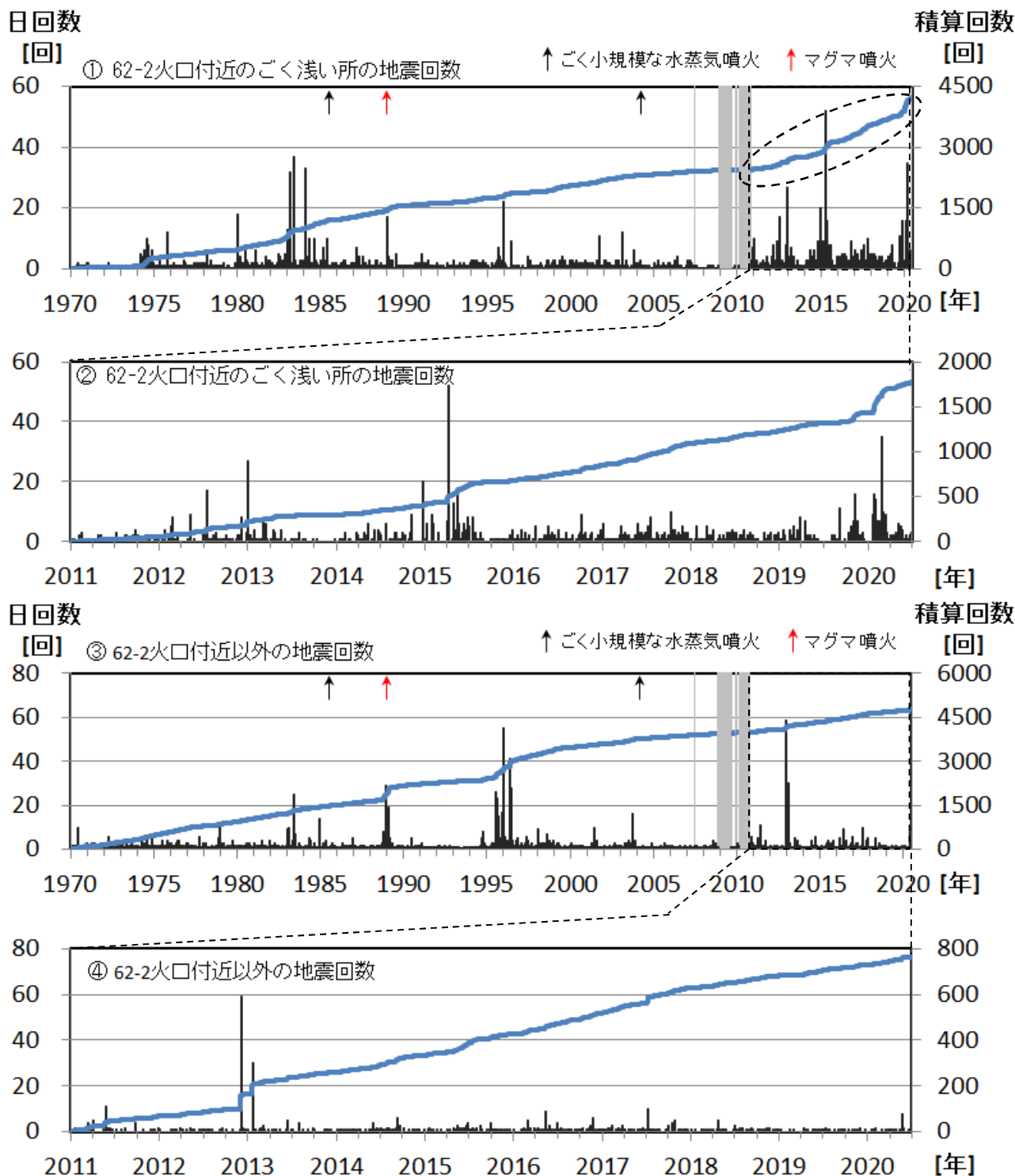
図9 十勝岳 地震の日回数及び積算回数 (①③: 1970年~2020年6月 ②④: 2011年~2020年6月) 硫黄沢観測点 (山麓点) で計測した回数 (計数基準: 0.05 μm以上) を示します。 ①、②は主に62-2火口付近のごく浅い所 (図8中の破線に囲まれた領域内) で発生したと推測されるB型地震の回数を示します。また③、④の「62-2火口付近以外」とは、主にグラウンド火口周辺や旧噴火口付近などで発生したと推測されるA型地震の回数を示します。 図中の、青線は積算回数を示し、灰色の部分は欠測を示します。
