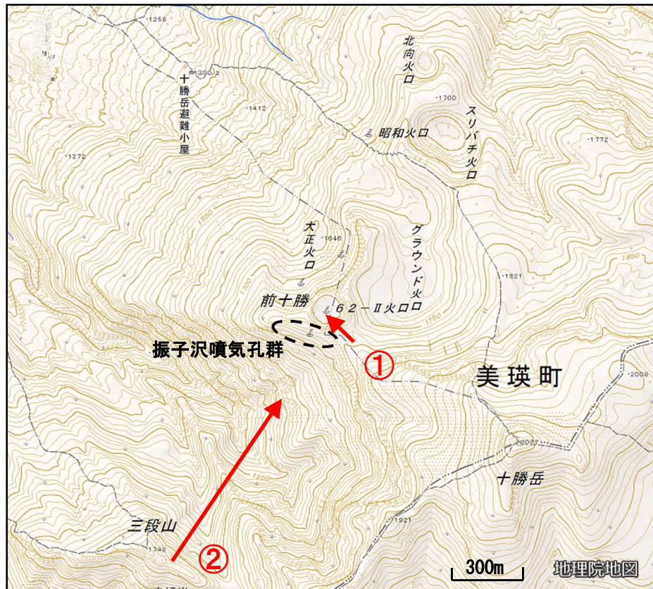
図5 十勝岳 図6、7の写真及び赤外熱映像の撮影方向
