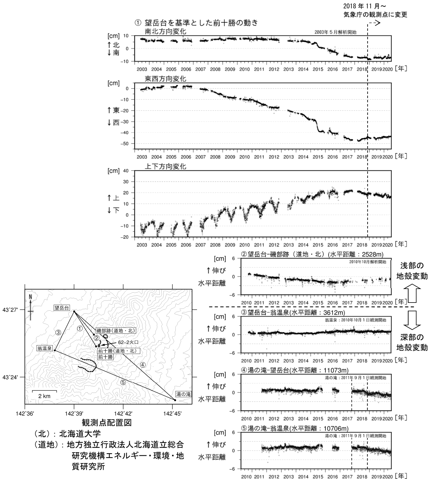
図10 十勝岳 GNSS連続観測による水平距離及び上下変化（2003年5月～2020年6月）
