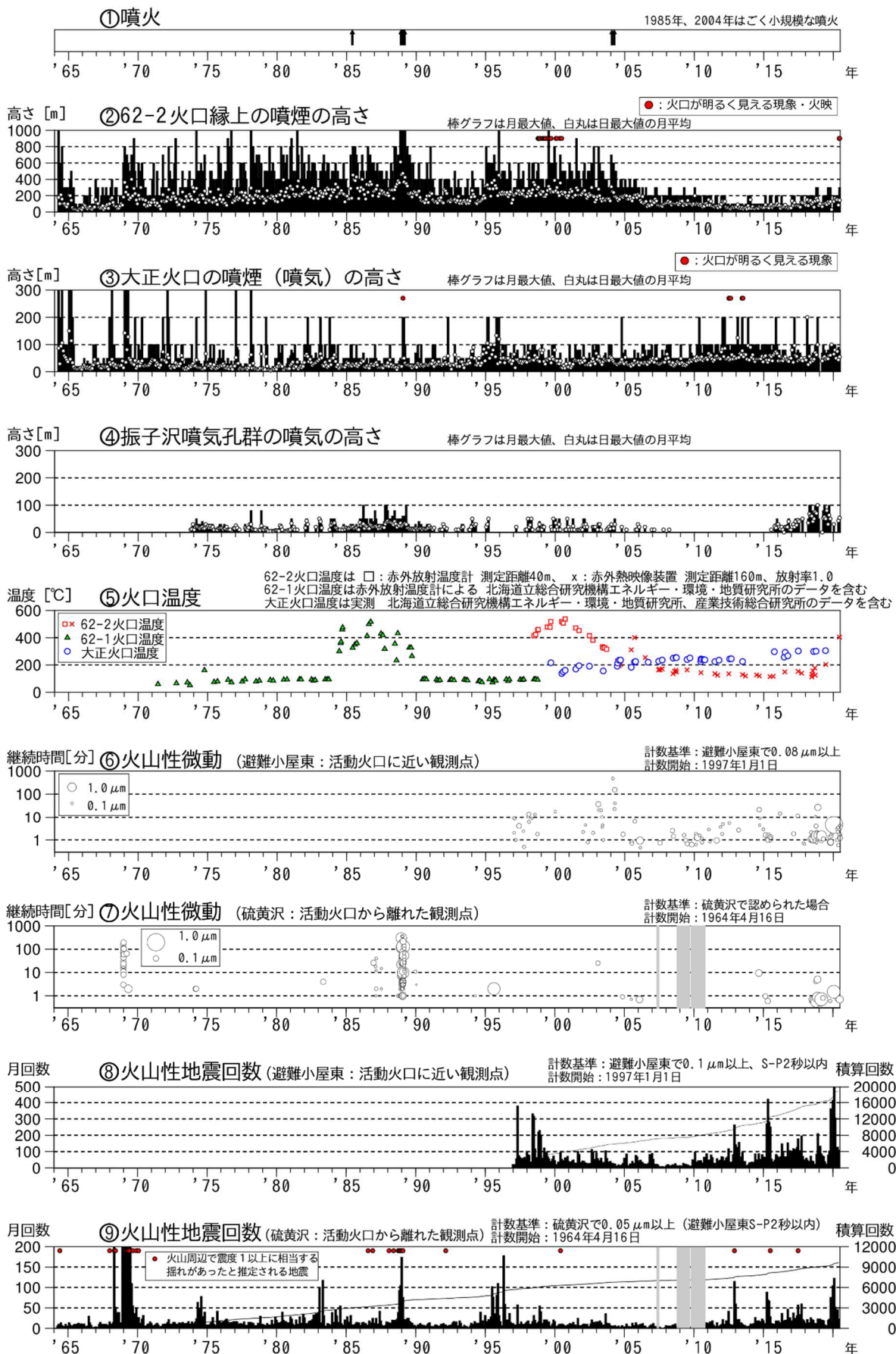
図1 十勝岳 火山活動経過図（1964年1月～2020年6月）
