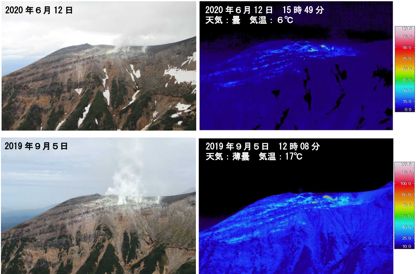
図7 十勝岳 赤外熱映像装置による振子沢噴気孔群の地表面温度分布 三段山（図5-②）から撮影
