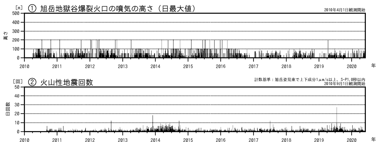
図1 大雪山 火山活動経過図（2010年4月～2020年5月）
