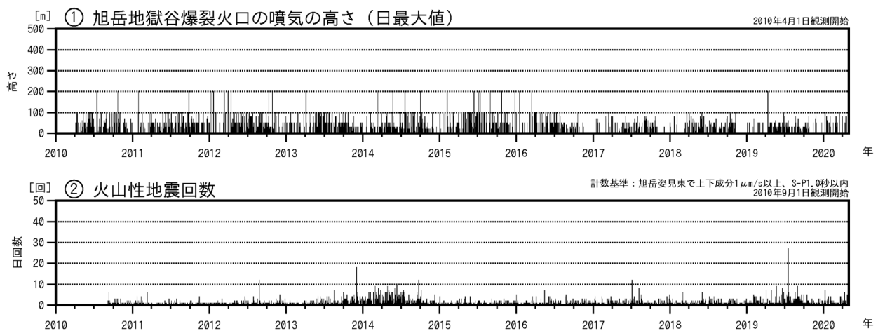
図1 大雪山 火山活動経過図（2010年4月～2020年4月）
