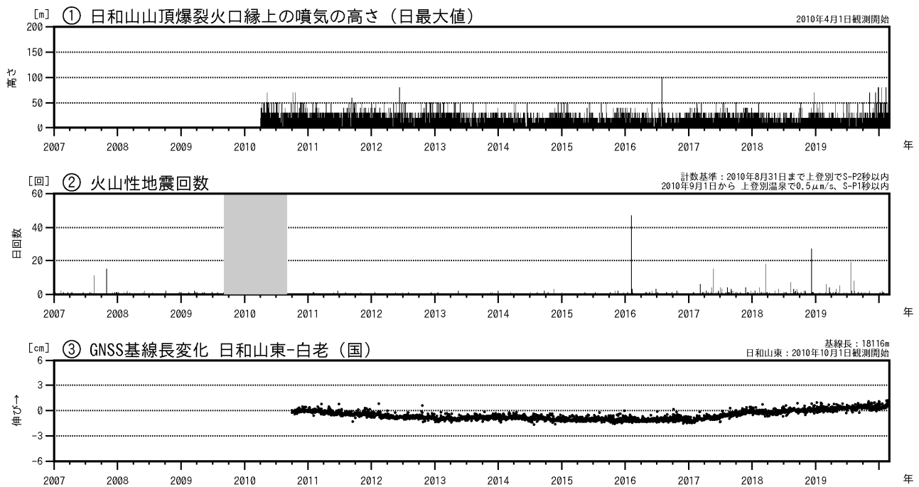
図2 倶多楽 火山活動経過図（2007年1月～2020年2月）
