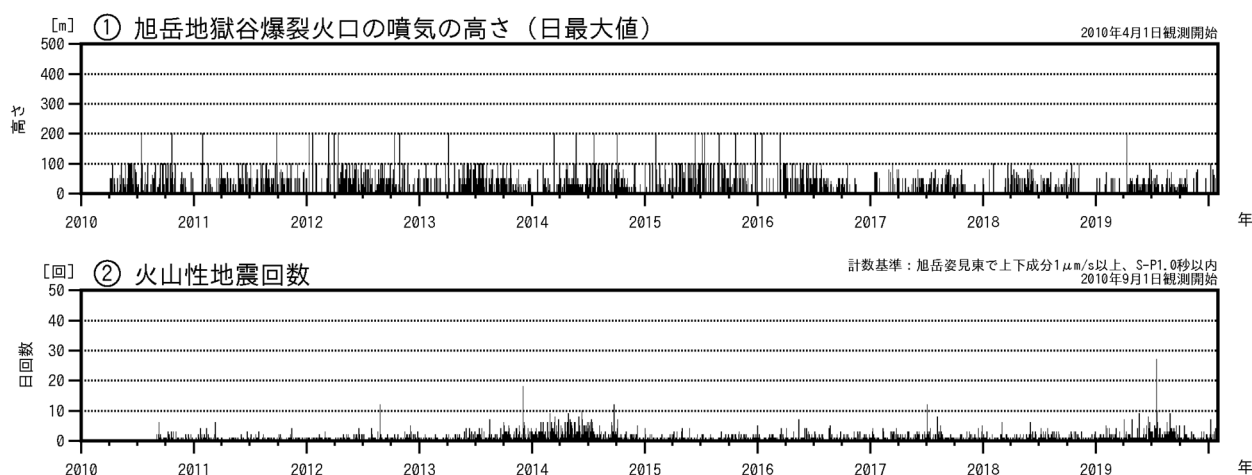
図1 大雪山 火山活動経過図（2010年4月～2020年1月）
