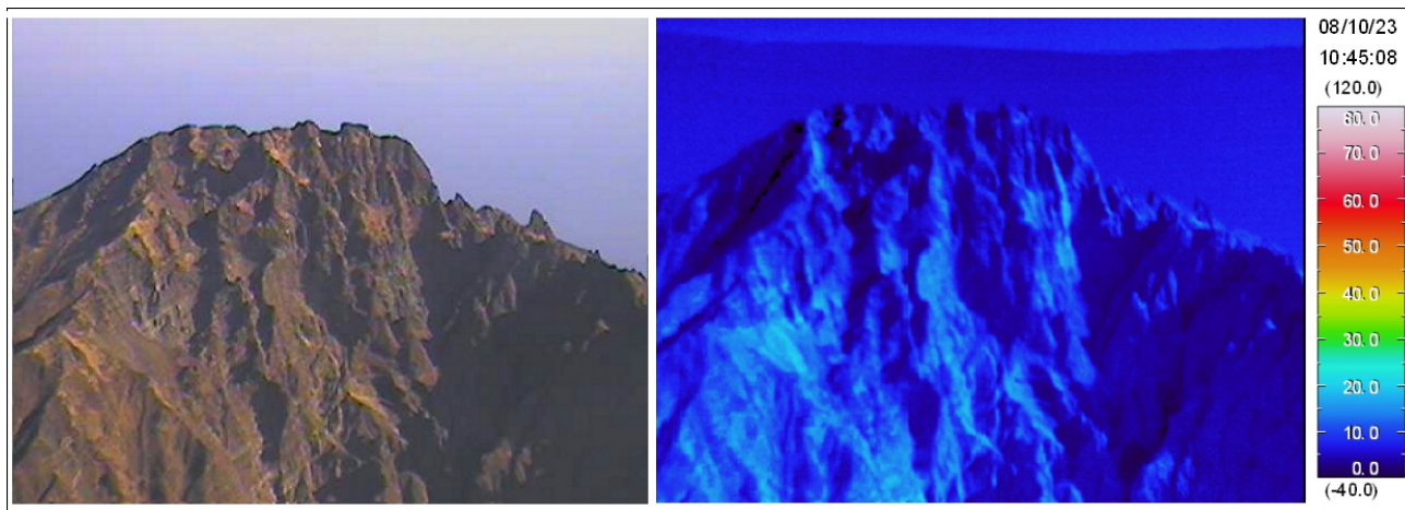
図 3 利尻山 赤外熱映像装置 1) による山頂の地表面温度分布
