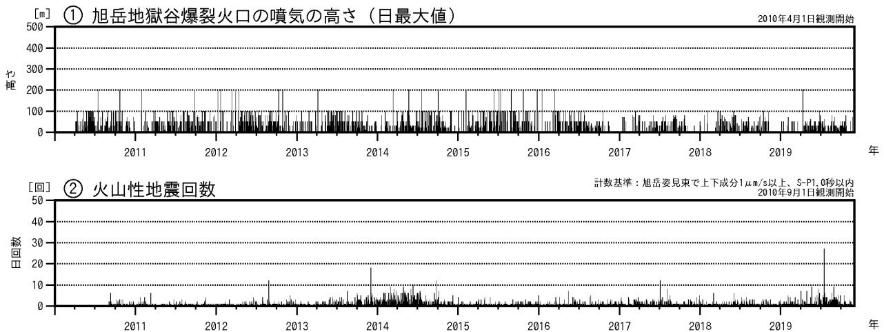
図1 大雪山 火山活動経過図（2010年4月～2019年11月）
