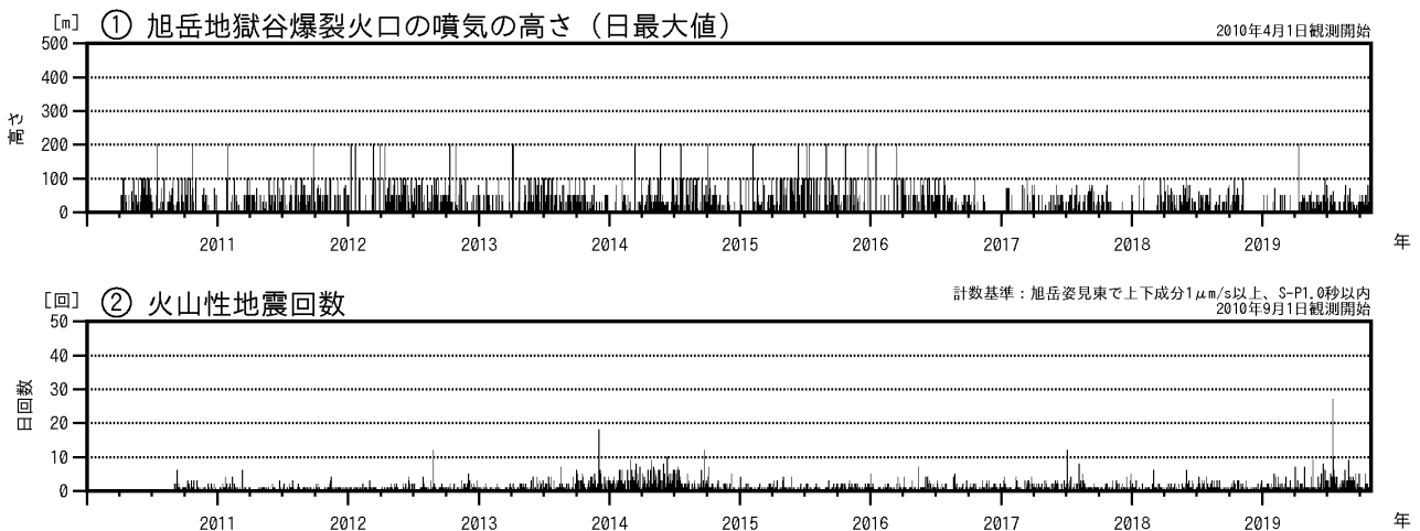
図1 大雪山 火山活動経過図（2010年4月～2019年10月）
