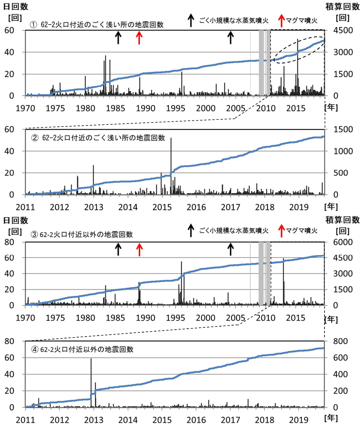
図9 十勝岳 地震の日回数及び積算回数（①③：1970年～2019年9月 ②④：2011年～2019年9月） 硫黄沢観測点（山麓点）で計測した回数（計数基準：0.05 \mu m以上）を示します。 ③、④の「62-2火口付近以外」とは、グラウンド火口周辺や旧噴火口付近などのことを指します。 図中の、青線は積算回数を示し、灰色の部分欠測を示します。
