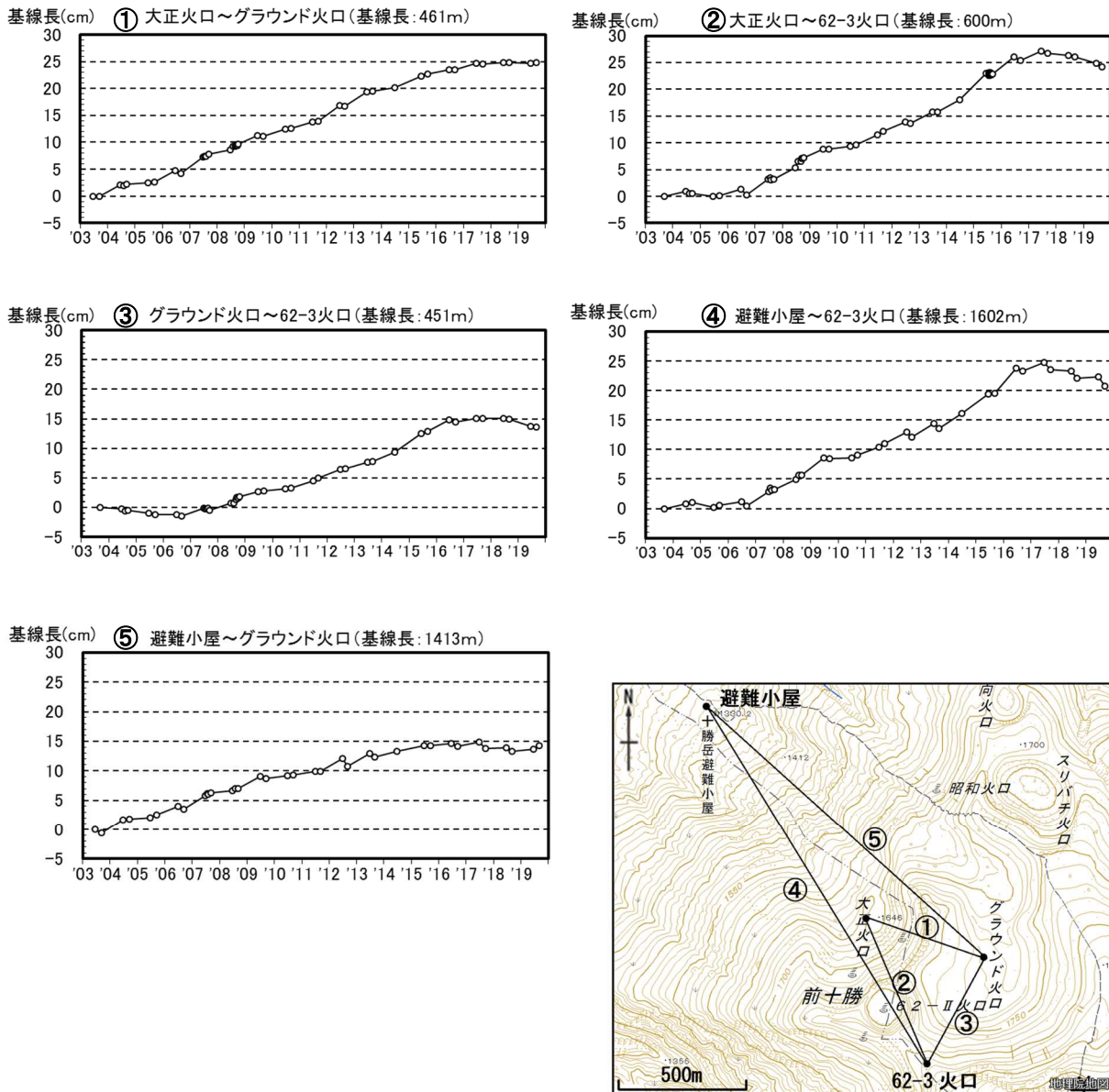
図11 十勝岳 GNSS繰り返し観測による基線長変化（2003年9月～2019年9月）及び観測点配置図 GNSS基線①～⑤は観測点配置図の①～⑤に対応しています。
