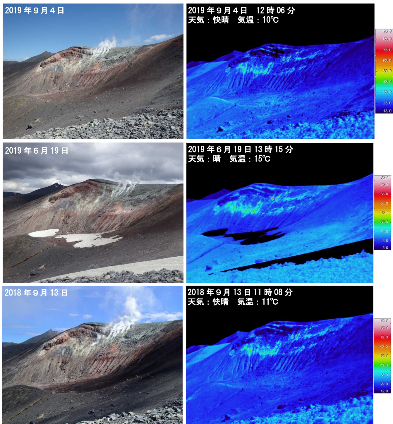
図7 十勝岳 赤外熱映像装置による大正火口東壁の地表面温度分布 南西側（図3の④）から撮影
