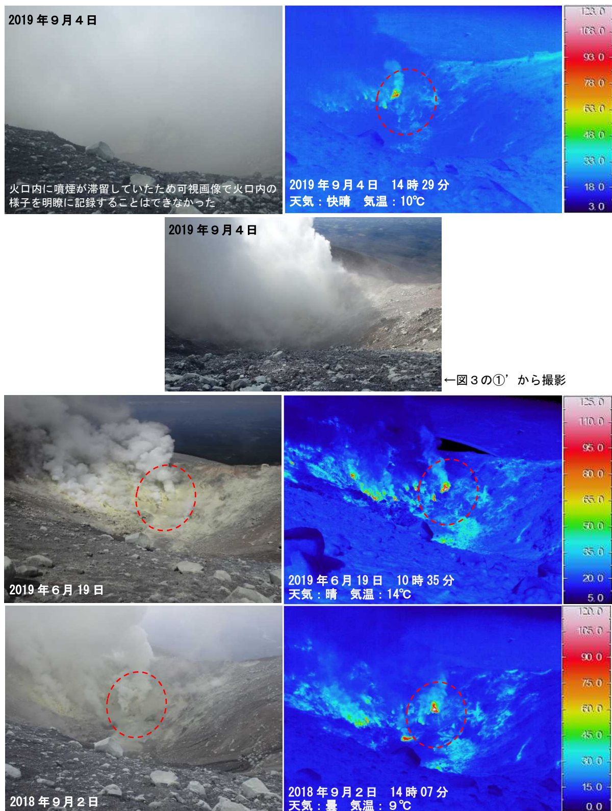
図4 十勝岳 赤外熱映像装置による62-2火口内の地表面温度分布 2段目以外はすべて南東側（図3の①）から撮影
