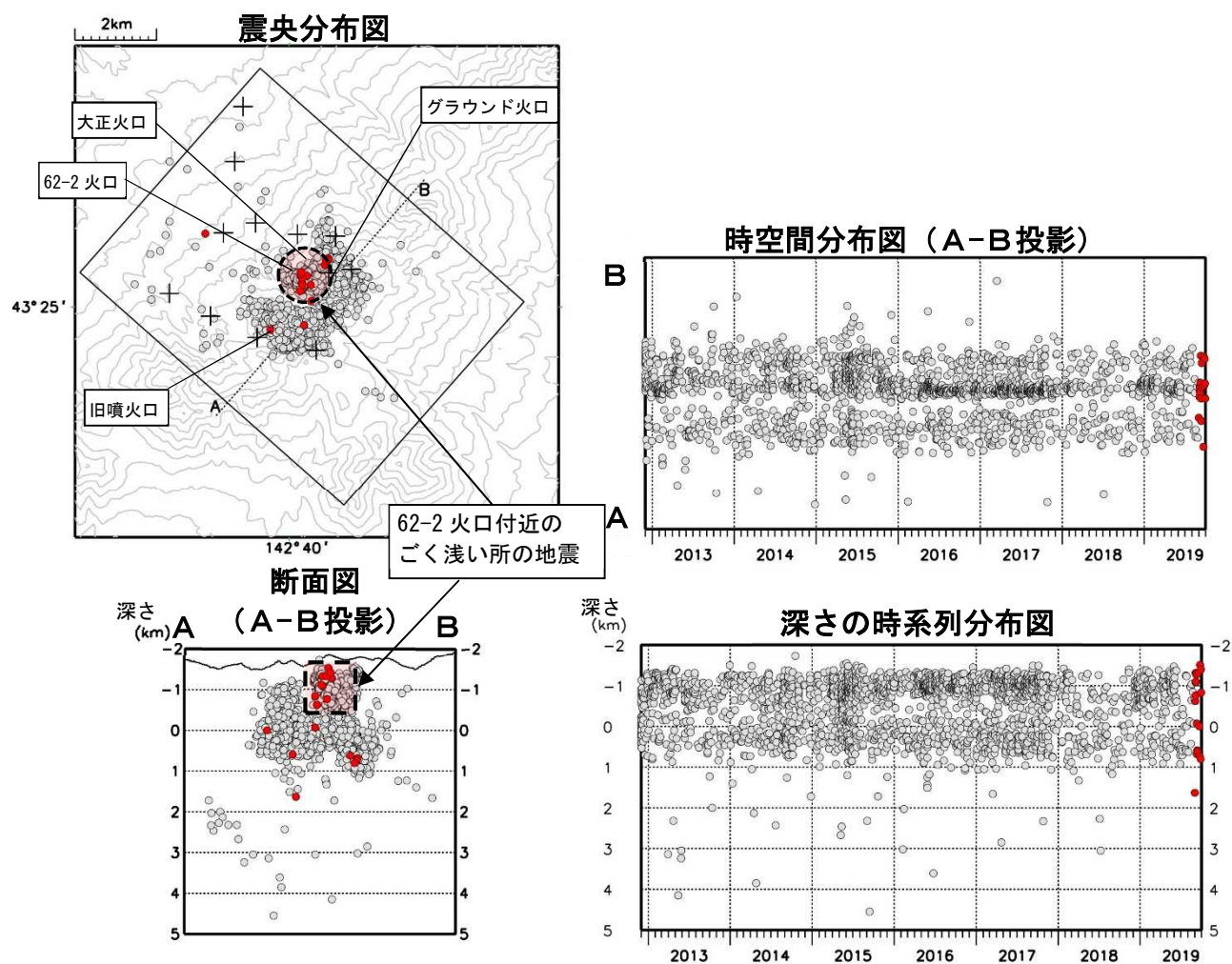
図8 十勝岳 火山性地震の震源分布（2012年12月～2019年9月） ●：2012年12月～2019年8月の震源 ●：2019年9月の震源 +：地震観測点
