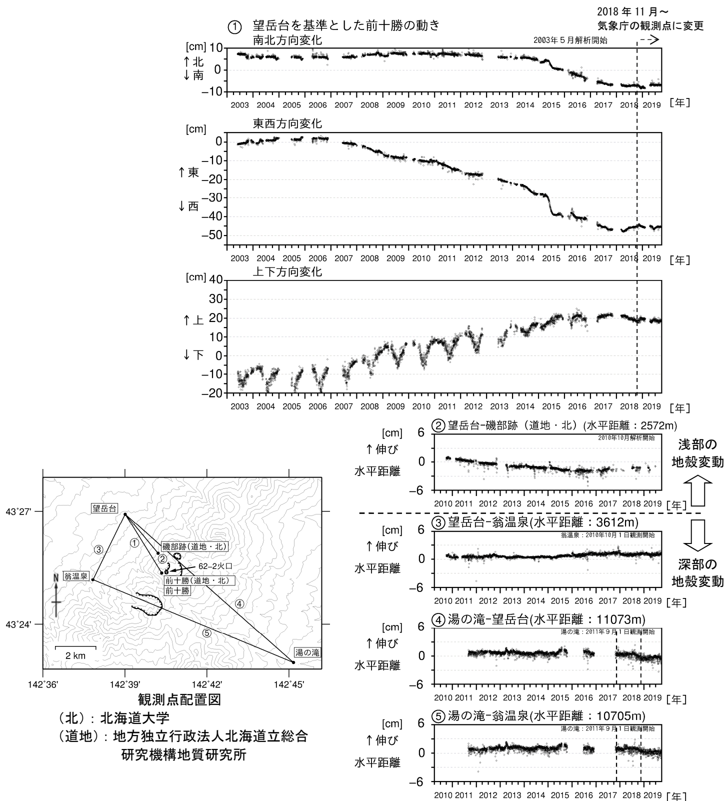
図10 十勝岳 GNSS連続観測による水平距離及び上下変化（2003年5月～2019年9月）
