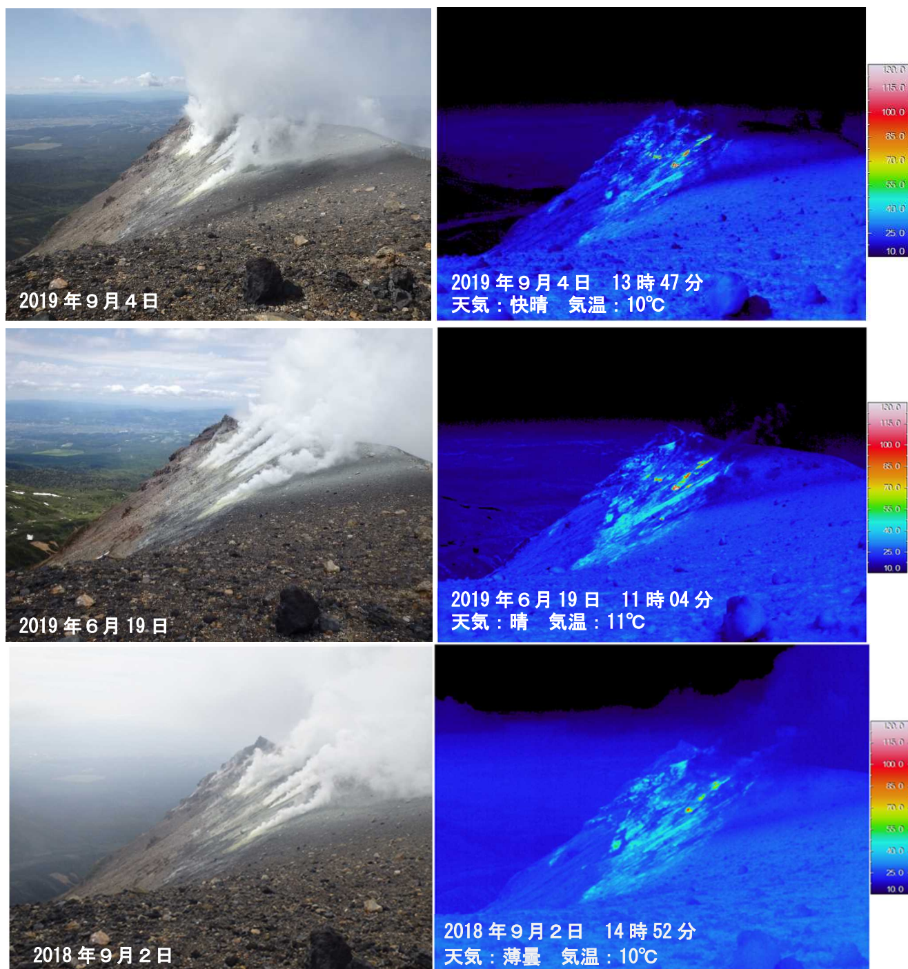
図5 十勝岳 赤外熱映像装置による振子沢噴気孔群の地表面温度分布 南東側（図3の②）から撮影
