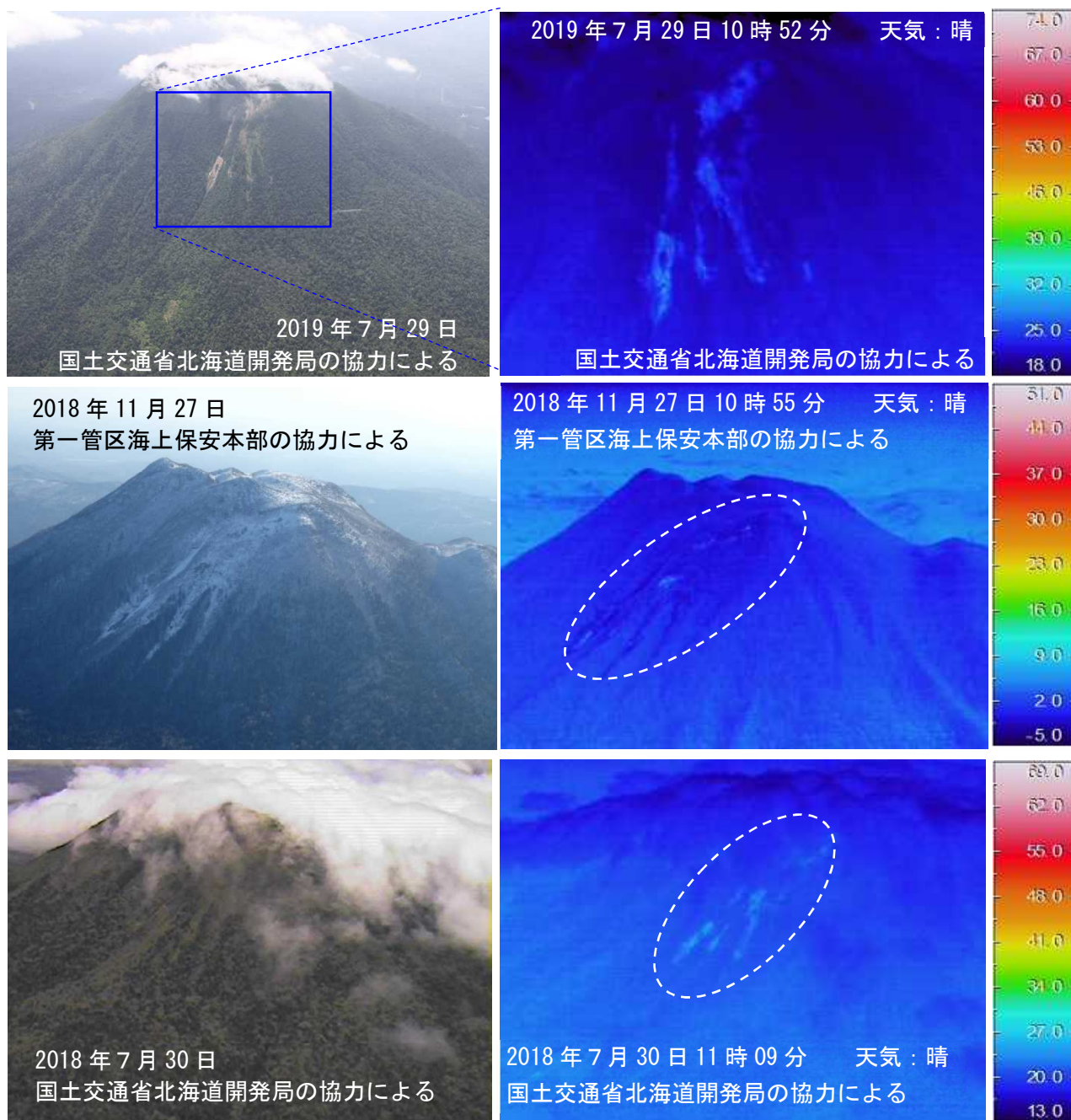
図2 雄阿寒岳 赤外熱映像装置による北西斜面の地表面温度分布の比較
