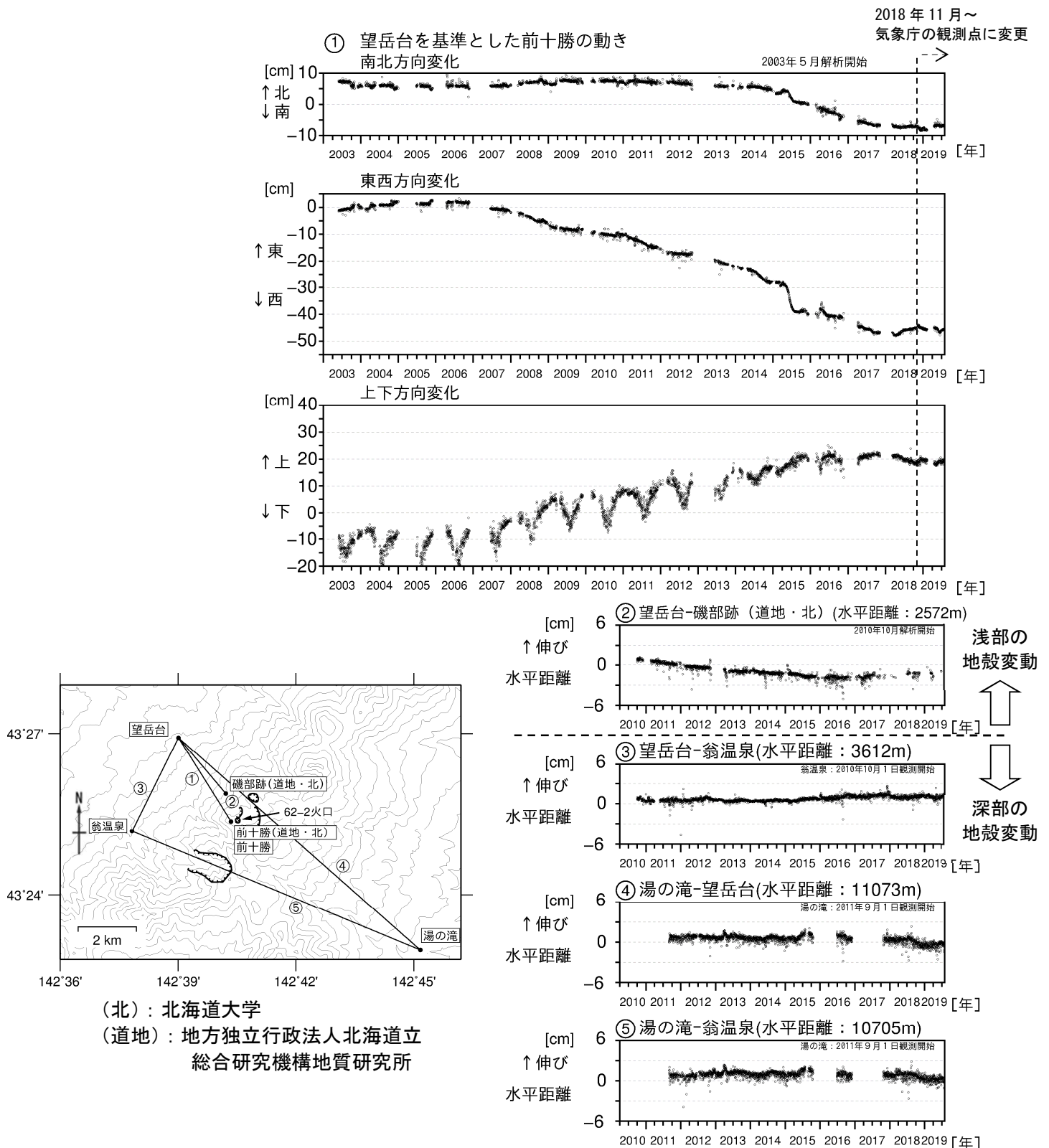
図5 十勝岳 GNSS連続観測による水平距離及び上下変化（2003年5月～2019年7月）及び観測点配置図
