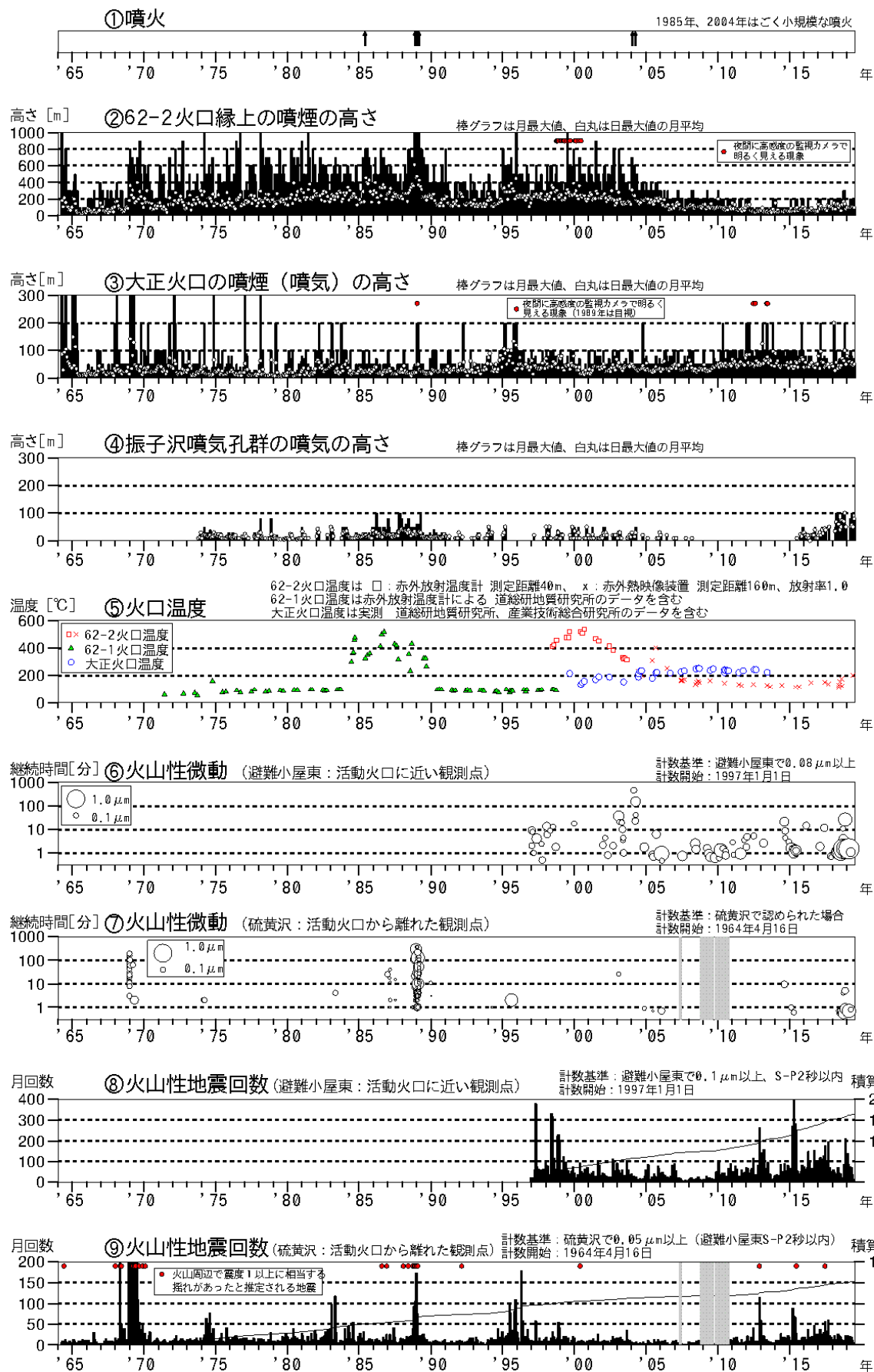
図1 十勝岳 火山活動経過図（1964年1月～2019年7月）
