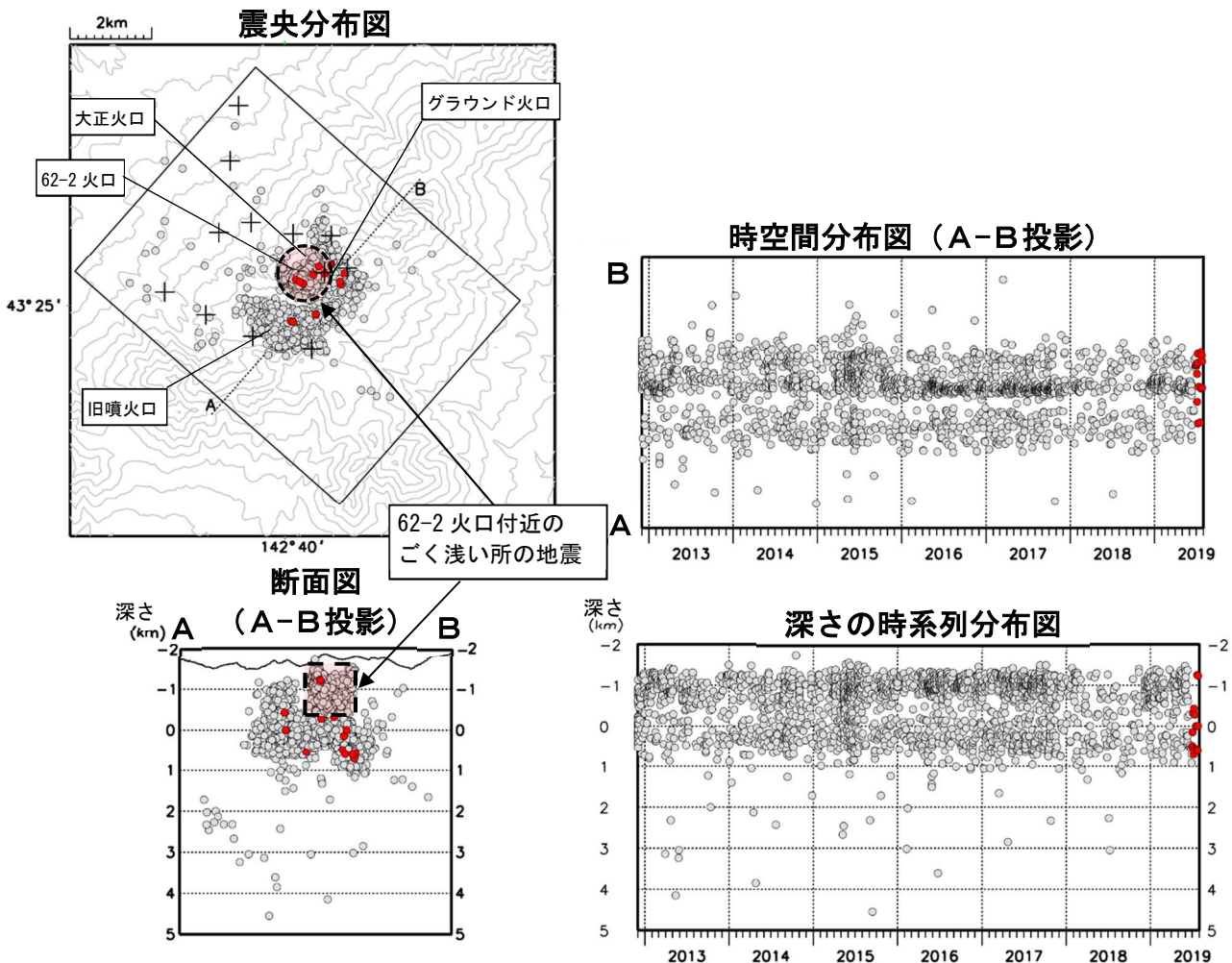
図3 十勝岳 火山性地震の震源分布（2012年12月～2019年7月）
