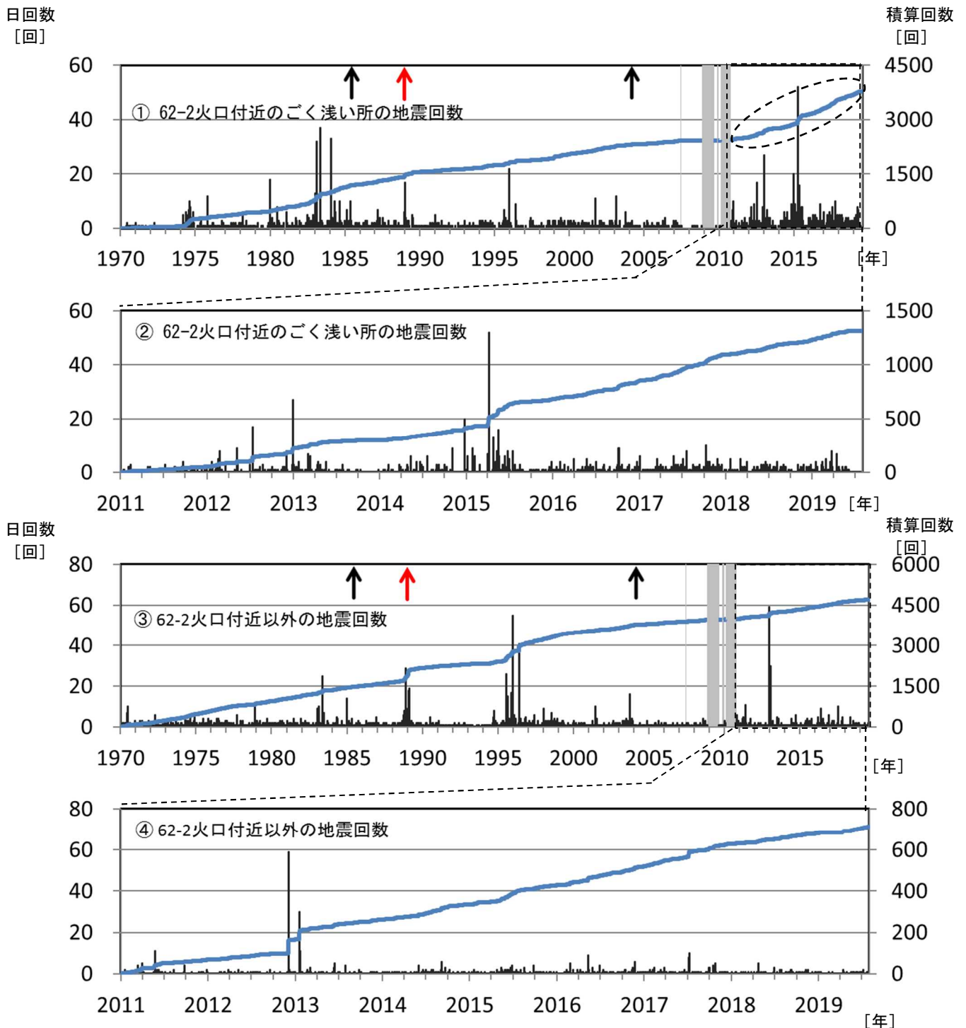
図4 十勝岳 地震の日回数及び積算回数（①、③：1970年～2019年7月 ②、④：2011年～2019年7月）
