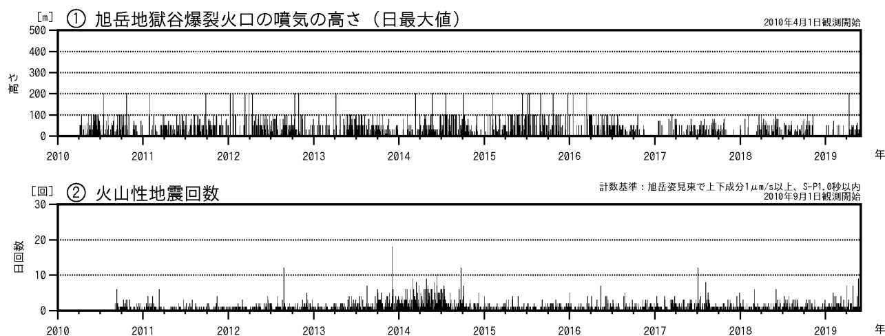
図1 大雪山 火山活動経過図（2010年4月～2019年5月）
