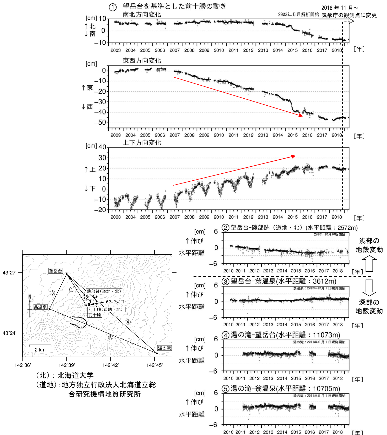
図 5 十勝岳 GNSS連続観測による水平距離及び上下変化（2003年 5 月～2019年 4 月）及び観測点配置図 GNSS基線①～⑤は観測点配置図の①～⑤に対応しています。 GNSS基線の空白部分は欠測を示します。 2010年10月と2016年 1 月に解析方法を変更しています。 ・基線①では2006年頃から62-2火口浅部の膨張を示す動き（赤矢印）が観測されていましたが、2017年秋頃から停滞し、2018年春頃から収縮を示す動きに転じた可能性があります。
