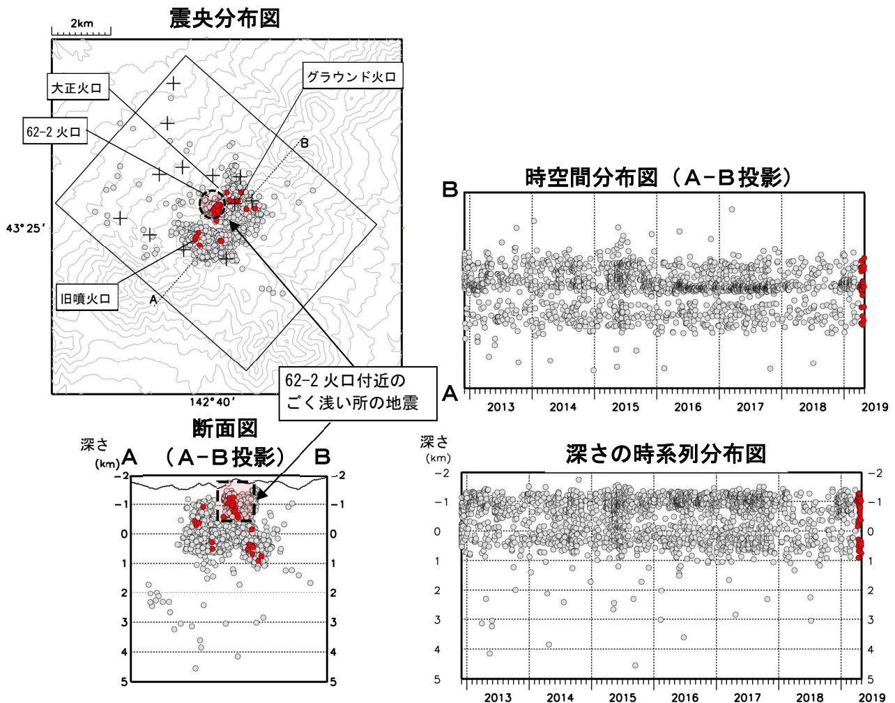
図3 十勝岳 火山性地震の震源分布（2012年12月～2019年4月）
