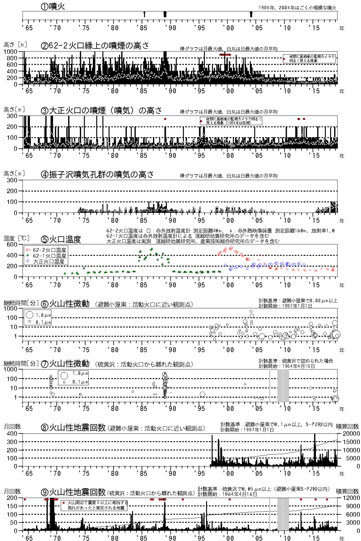
図1 十勝岳 火山活動経過図（1964年1月～2019年4月）
