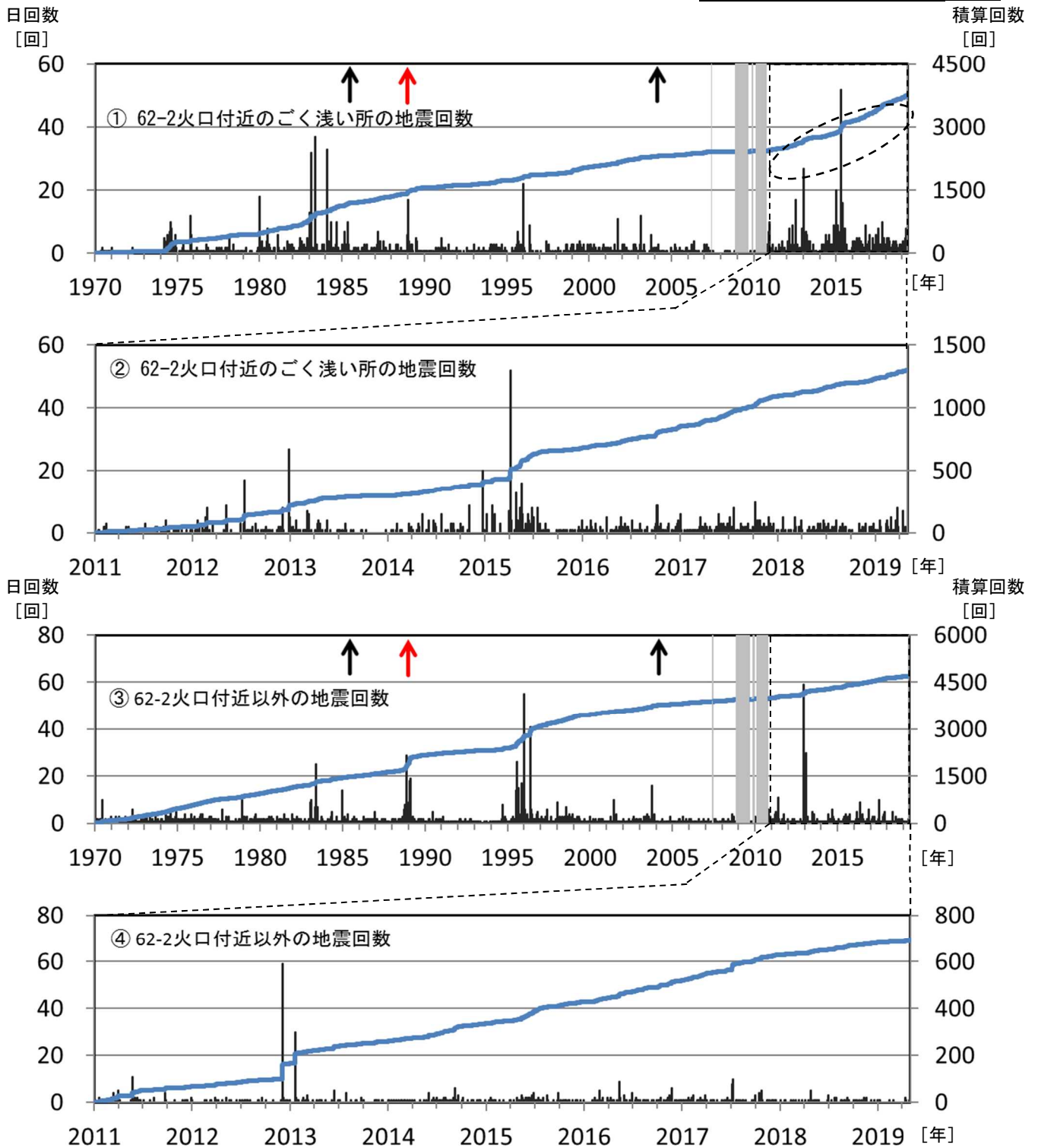
図4 十勝岳 地震の日回数及び積算回数（①、③：1970年～2019年4月 ②、④：2011年～2019年4月）
