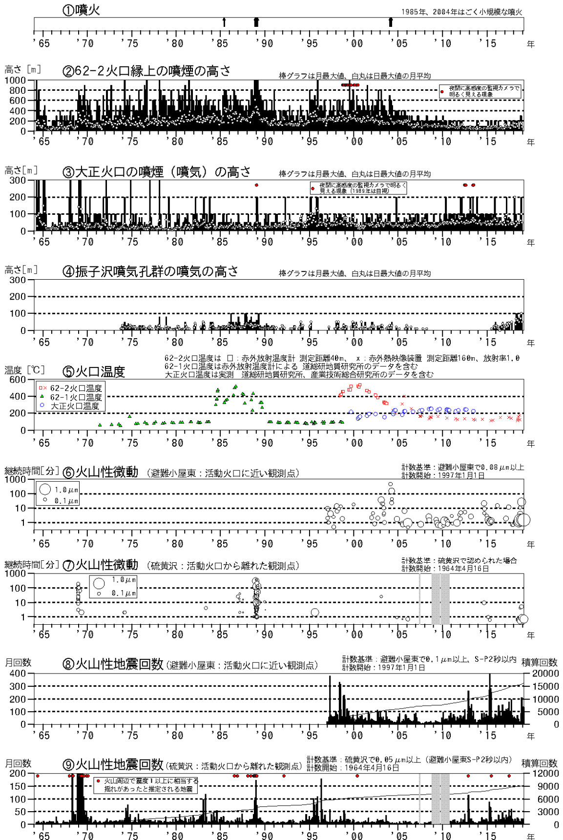
図1 十勝岳 火山活動経過図（1964年1月～2019年2月）
