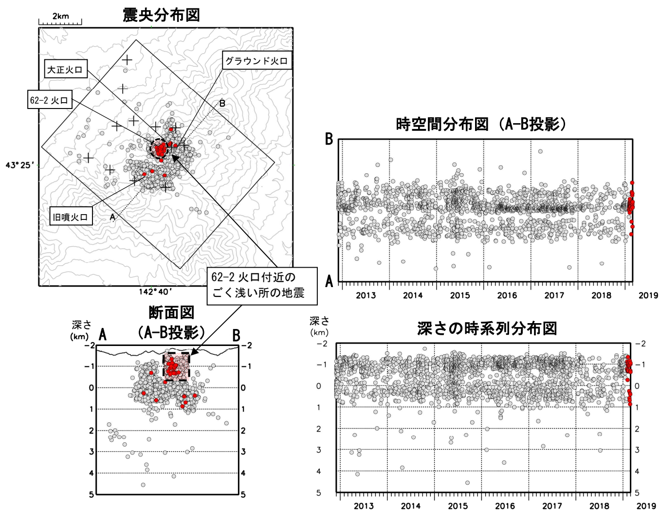
図 3 十勝岳 火山性地震の震源分布（2012年12月～2019年 2 月）
