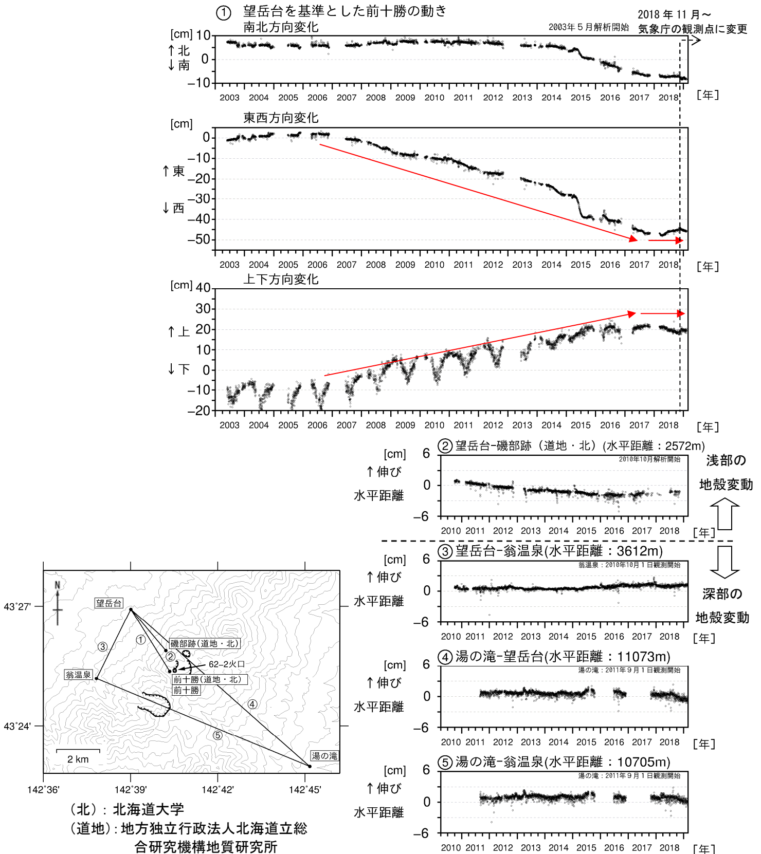
図 5 十勝岳 GNSS連続観測による水平距離及び上下変化（2003年 5 月～2019年 2 月）及び観測点配置図
