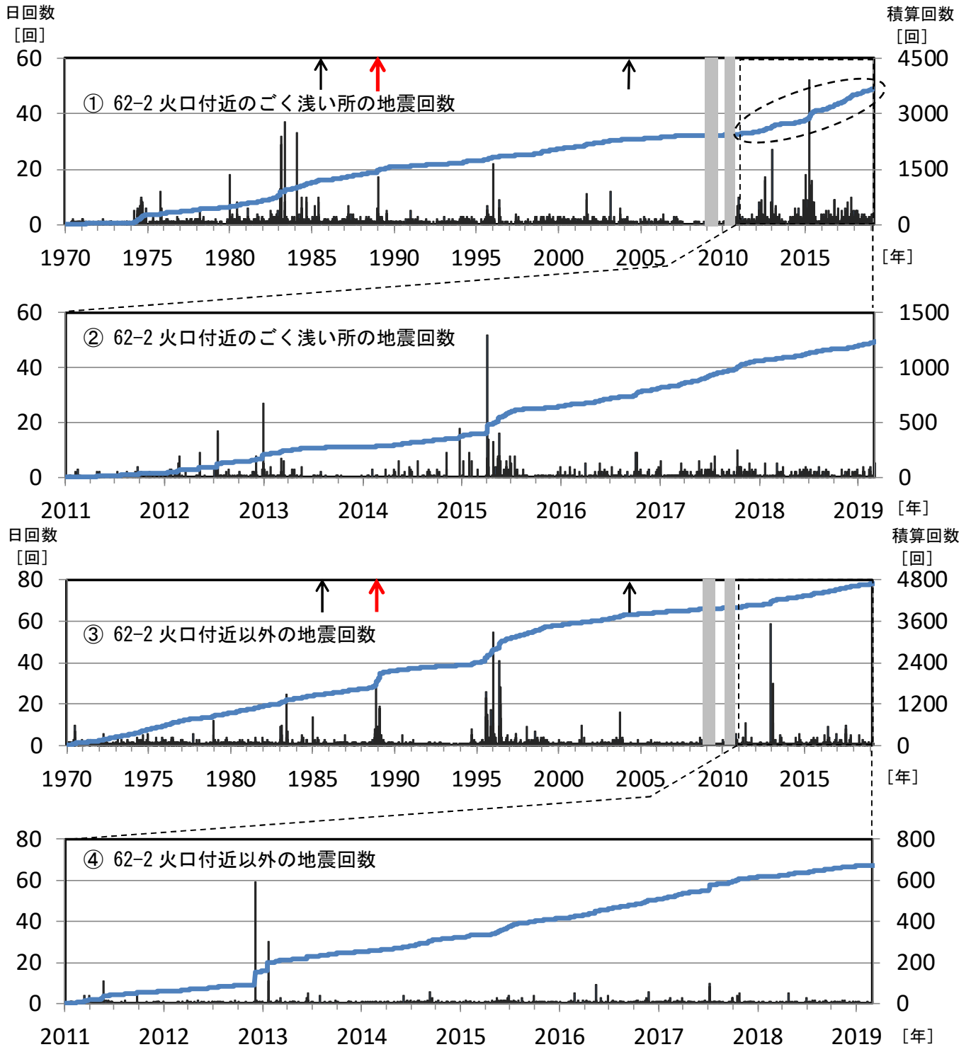
図4 十勝岳 地震の日回数及び積算回数（①、③：1970年～2019年2月 ②、④：2011年～2019年2月）
