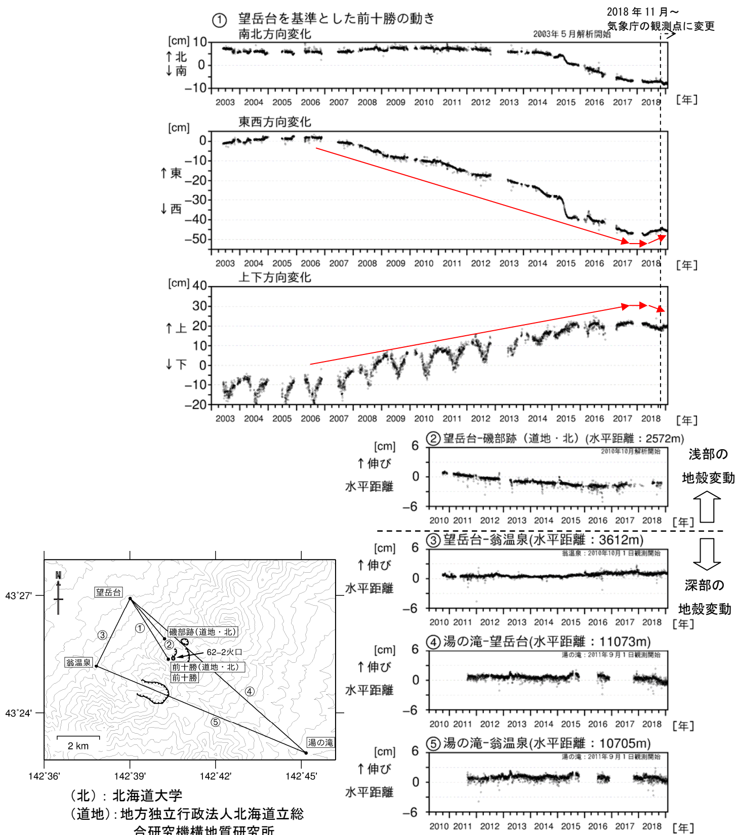
図6 十勝岳 GNSS連続観測による水平距離及び上下変化 (2003年5月～2019年1月) 及び観測点配置図
