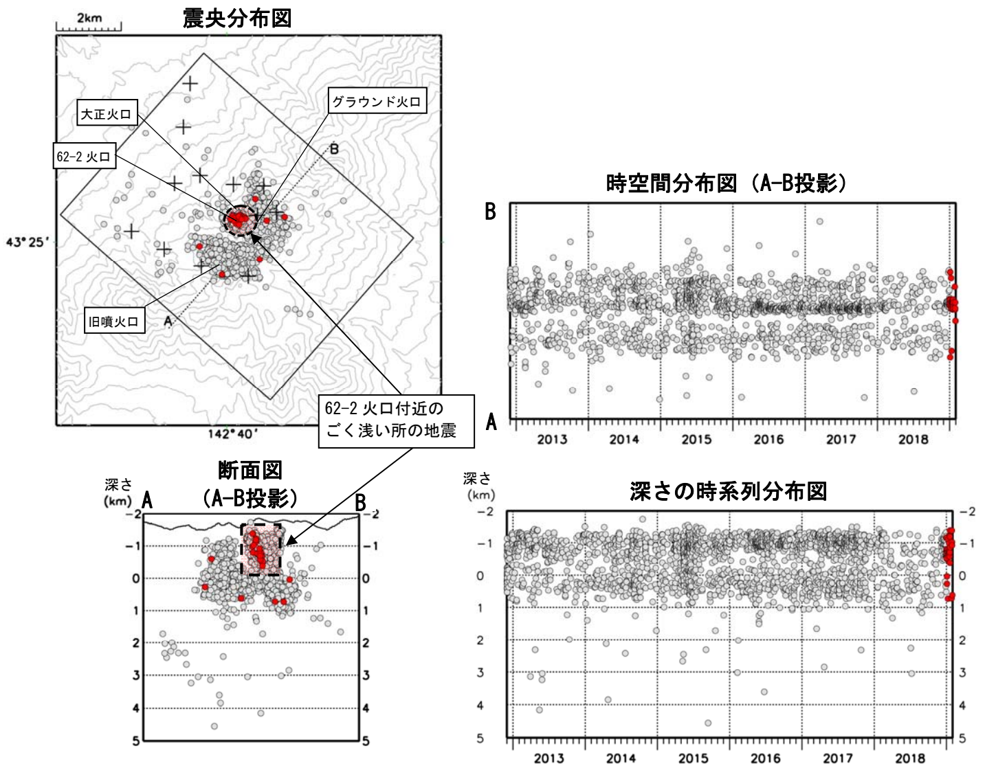
図4 十勝岳 火山性地震の震源分布 (2012年12月～2019年1月)
