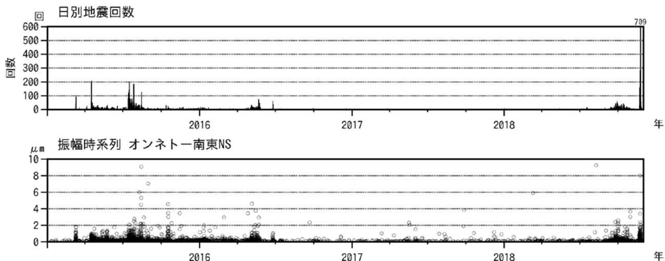
図7 雌阿寒岳 火山性地震の日別回数（上段）及びオンネトー南東（南北成分）の変位振幅時系列（下段） （2015年1月1日～2018年11月27日12時）
