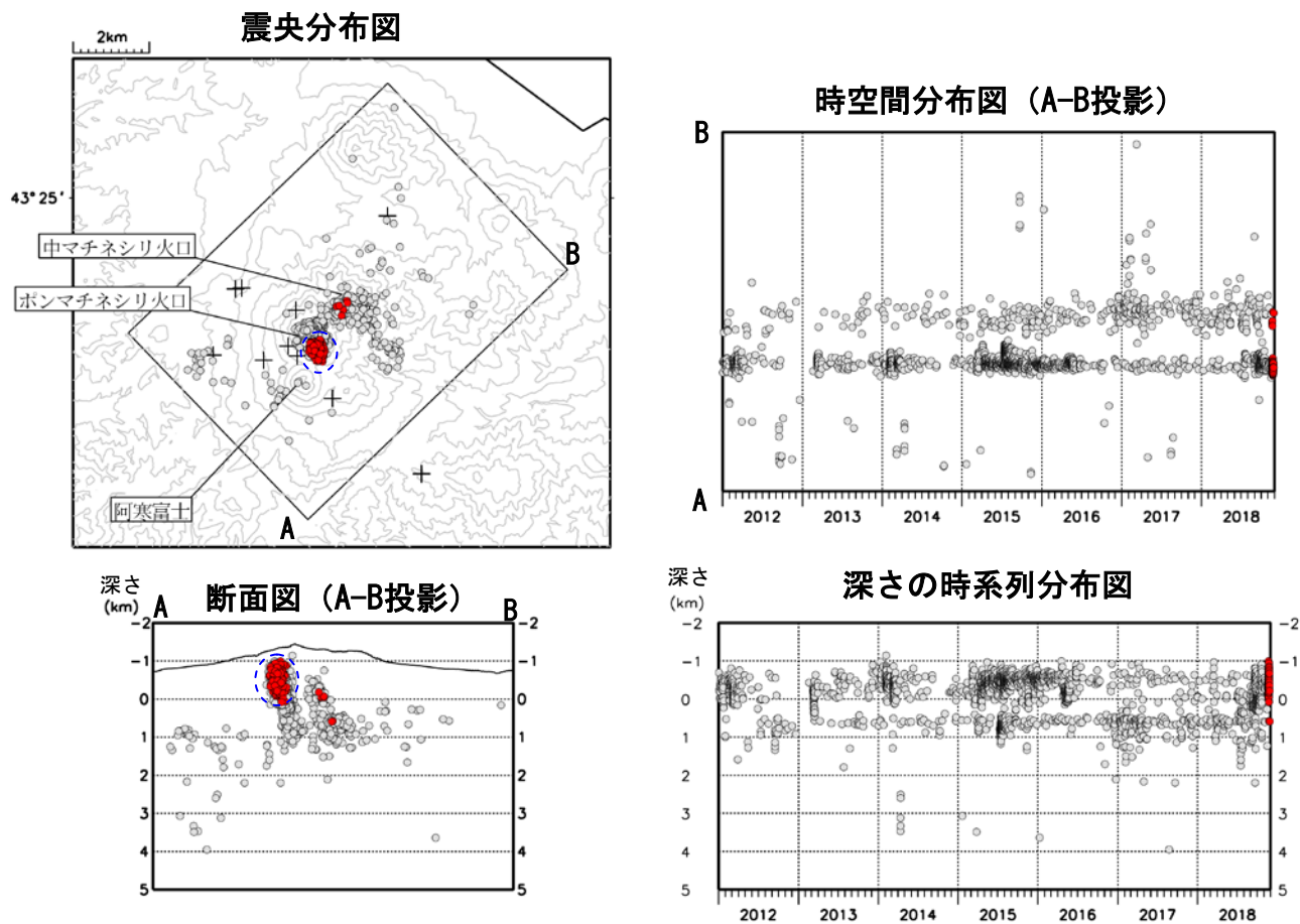
図 9 雌阿寒岳 火山性地震の震源分布（2012年1月～2018年11月27日）
