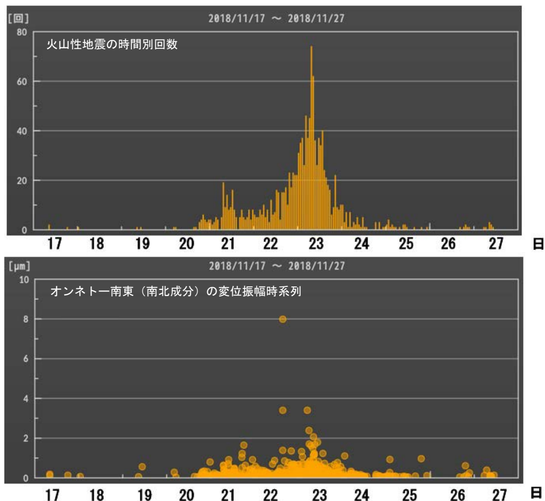
図8 雌阿寒岳 火山性地震の時間別回数（上段）及びオンネトー南東（南北成分）の変位振幅時系列（下段）（11月17日00時～27日12時） ・24日以降、火山性地震は減少しています。
