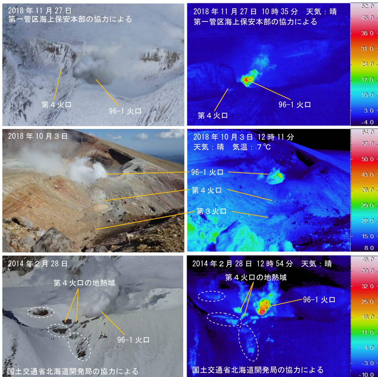
図 3 雌阿寒岳 赤外熱映像装置によるポンマチネシリ第 4 火口の地表面温度分布
