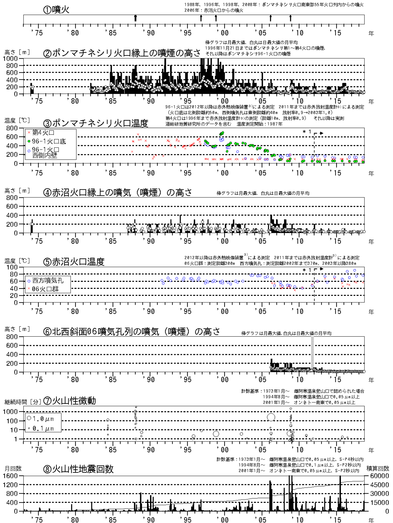
図1 雌阿寒岳 火山活動経過図（1973年1月～2018年9月）
