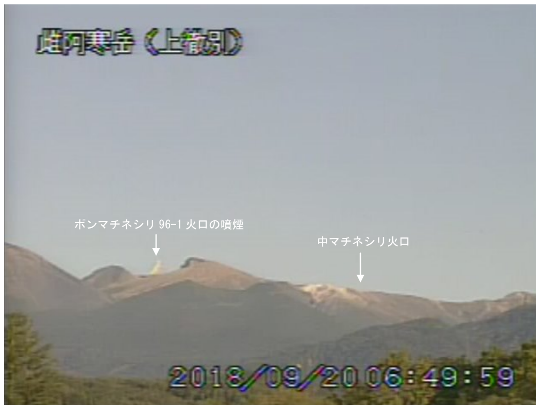
図 3 雌阿寒岳 南東側から見た山体の状況 （9月20日、上徹別監視カメラによる）
