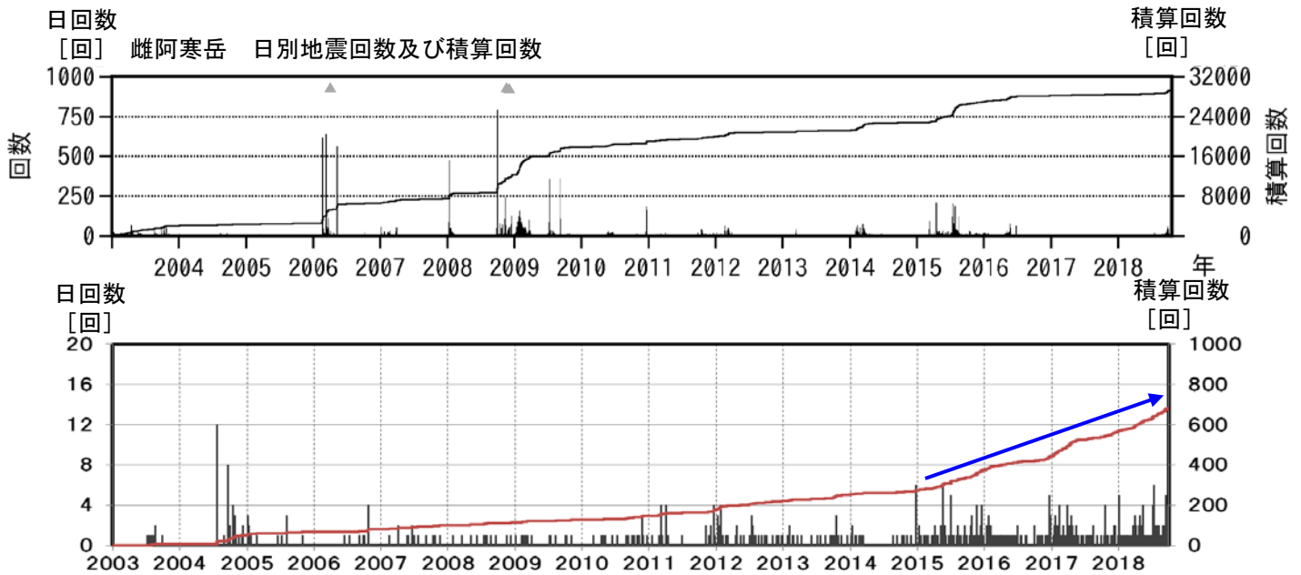
図5 雌阿寒岳 火山性地震の日別回数及び積算回数（2003年1月～2018年9月）
