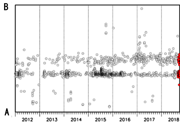
時空間分布図（A-B投影）
