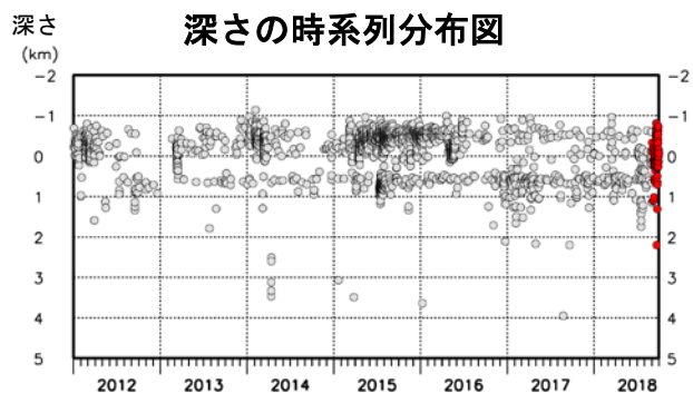
図6 雌阿寒岳 火山性地震の震源分布（2012年1月～2018年9月）
