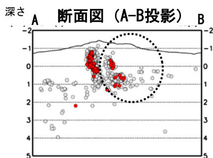
図6 雌阿寒岳 火山性地震の震源分布（2012年1月～2018年9月）
