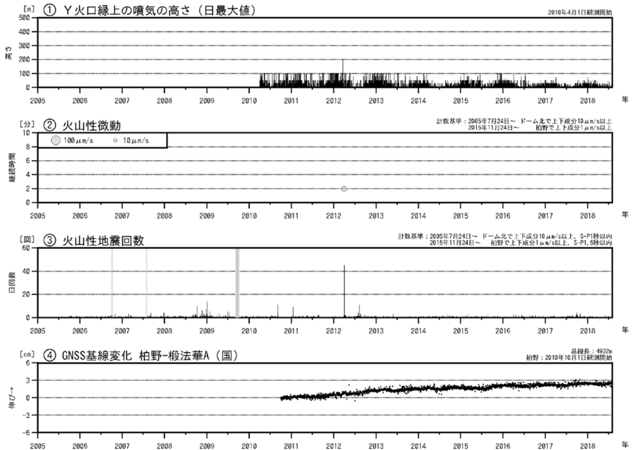
図2 恵山 火山活動経過図（2005年7月～2018年7月）
