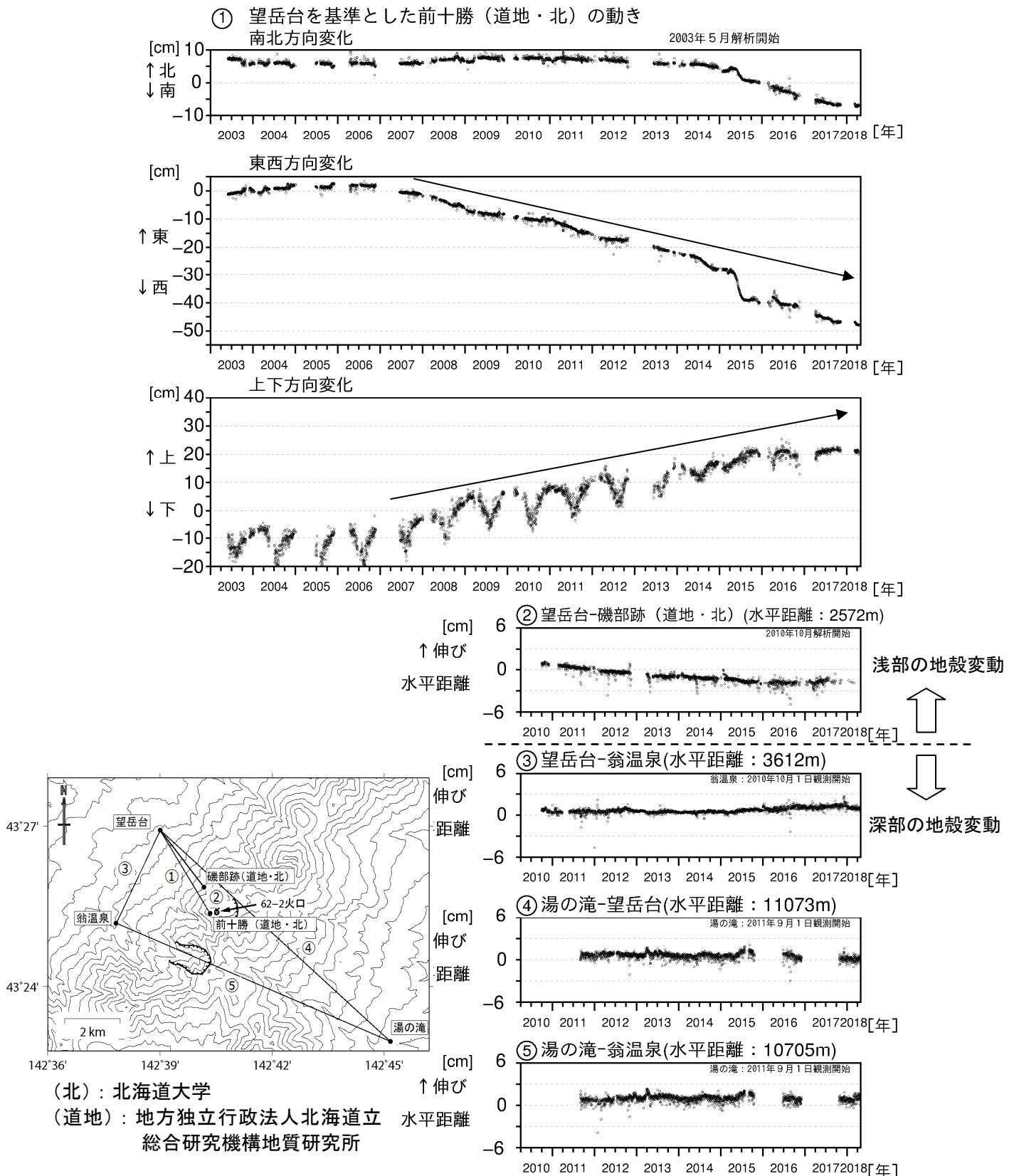
図6 十勝岳 GNSS連続観測による水平距離及び上下変化（2003年5月～2018年4月）とGNSS観測点配置図
