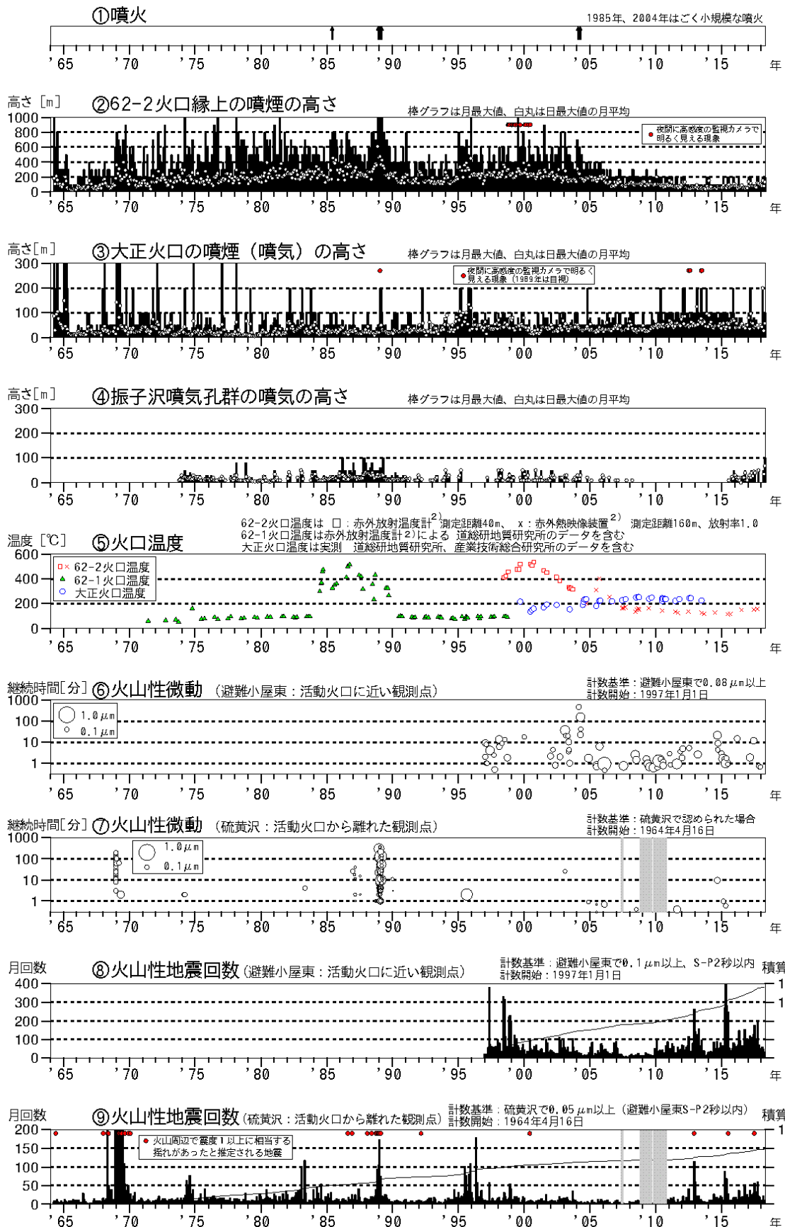
図1 十勝岳 火山活動経過図（1964年1月～2018年4月）
