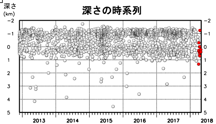
図4 十勝岳 火山性地震の震源分布（2012年12月～2018年4月） ●印：2012年12月～2018年3月の震源 ●印：2018年4月の震源 ＋印：地震観測点
