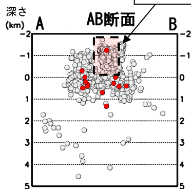
図4 十勝岳 火山性地震の震源分布（2012年12月～2018年4月） ●印：2012年12月～2018年3月の震源 ●印：2018年4月の震源 ＋印：地震観測点
