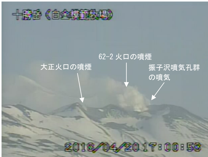
図2 十勝岳 北西側から見た火口周辺の状況 （4月20日、白金模範牧場監視カメラによる）
